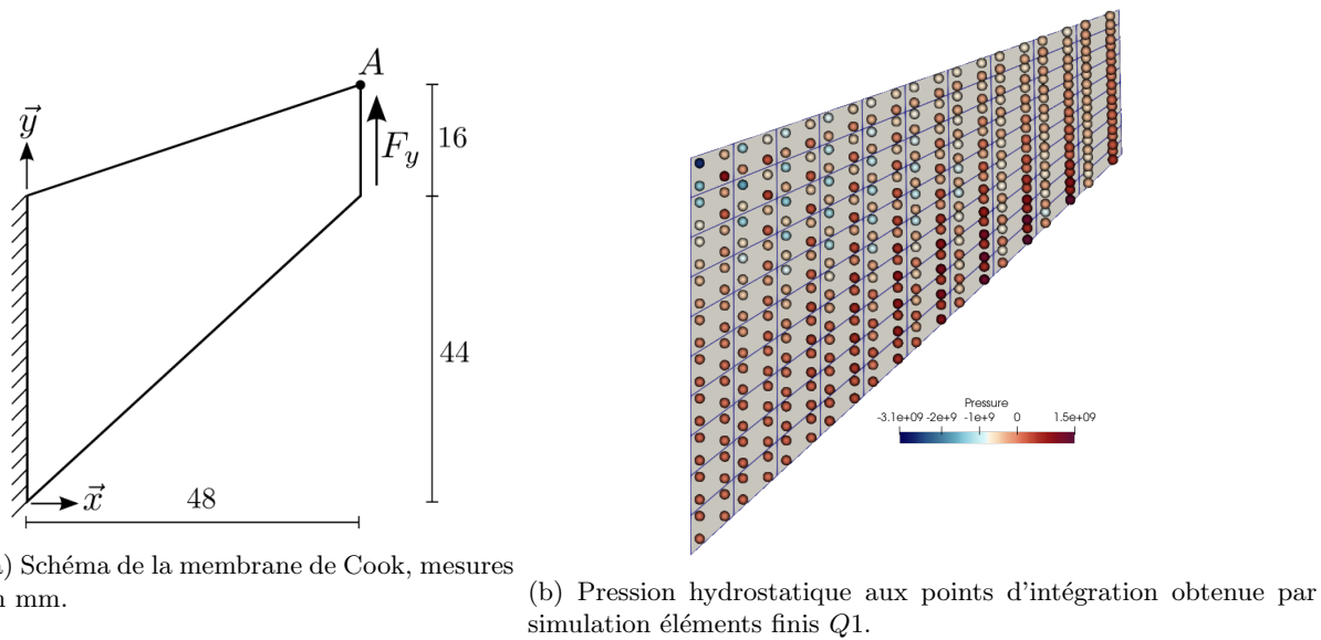
Figure 1.3: Membrane de Cook élastique quasi-incompressible : illustration du phénomène de verrouillage volumique.
