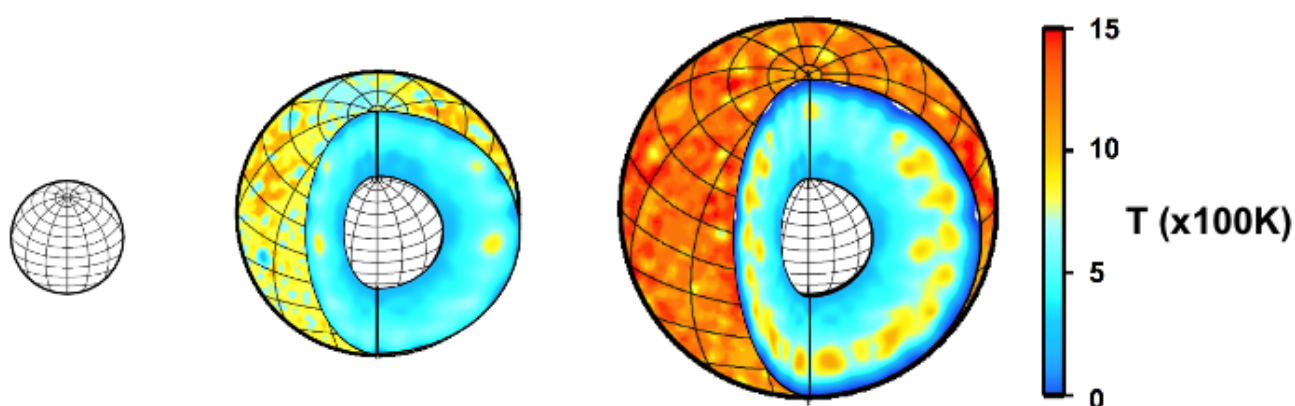
FIGURE 5 – Représentation de l'évolution topographique et thermique d'une planète en croissance à partir d'un objet tellurique de rayon 500 km (gauche) jusqu'à l'accrétion d'une planète de 3000 km de rayon. Après chaque impact la protoplanète grossit et une partie de l'énergie cinétique est dissipée sous forme de chaleur en profondeur (centre). À la fin de l'accrétion, les vitesses d'impact étant plus élevées, l'intensité du chauffage par impact est plus grande dans les parties externes de la planète (droite).
