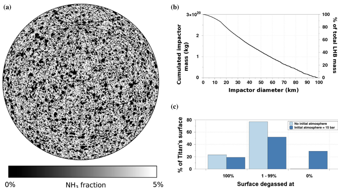
FIGURE 32 – (a) Distribution du \text{NH}_3 à la surface de Titan après un épisode de LHB (b) distribution des tailles d'impact cumulées pendant ce LHB et (c) taux de dégazage à la surface de Titan après le LHB pour la distribution illustrée dans le panel (a) (D'après Marounina et al. (2015)).
