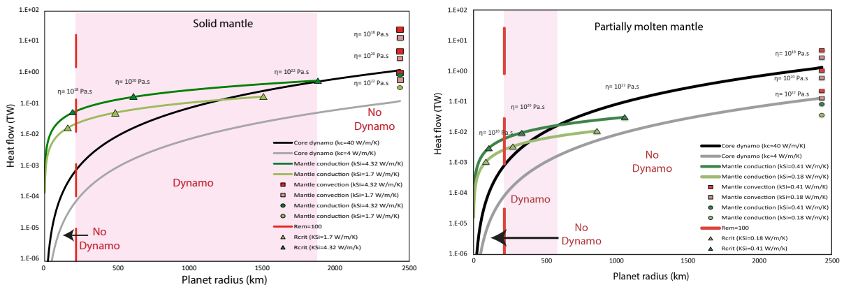
FIGURE 17 – Flux de chaleur en fonction du rayon planétaire pour un manteau planétaire entièrement solide (gauche) ou partiellement fondu (droite). Les lignes noires et grises représentent le flux de chaleur critique nécessaire à une dynamo thermique pour une conductivité thermique du noyau de 40 et 4 W/m/K, respectivement. Les lignes vertes foncées et claires représentent le flux de chaleur du manteau dans un régime conductif pour la gamme de conductivité thermique des silicates obtenue expérimentalement. Les triangles verts représentent la taille critique de la planète pour laquelle Ra = Ra_c , ce qui correspond donc au flux de chaleur minimum à la CMB, pour une viscosité du manteau allant de 10^{18} à 10^{22} Pa.s. Les valeurs extrapolées à R = R_{\text{Mercure}} = 2440 km sont également représentées avec des cercles verts pour les transferts de chaleur conductifs et des carrés rouges et roses pour les cas convectifs avec les viscosités du manteau indiquées à proximité. La ligne pointillée rouge représente la valeur critique pour Re_m = 100 . À gauche de cette ligne, une dynamo est peu probable. La zone probable pour un rayon de planète capable d'alimenter une dynamo est représentée par la zone ombrée en rose. À partir de Freitas et al. (2021).
