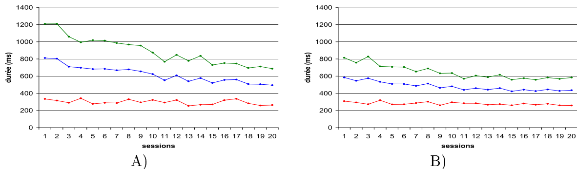
FIG. 55 – Temps de réaction spécifique sur le clavier SEB associé au système KeyGlass
