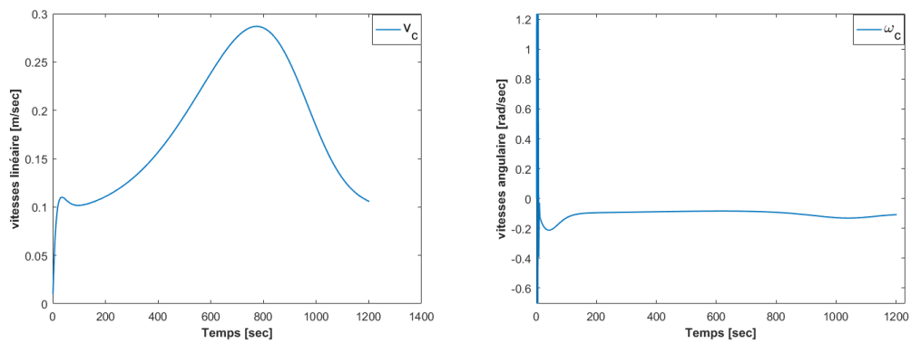
(c) Vitesse linéaire du robot
