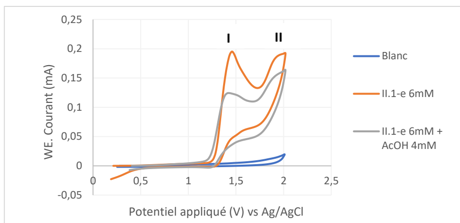
Figure II-5. Voltammogramme cyclique pour l'oxydation de II.1-e en présence de AcOH
