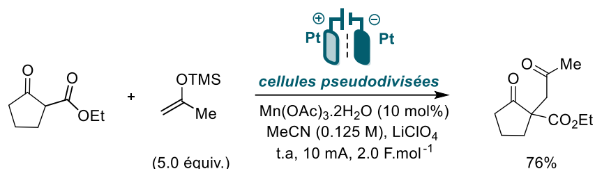
Schéma II-33. Addition de \beta -cétocesters à des éthers d'énol silylés, travaux de Hilt
