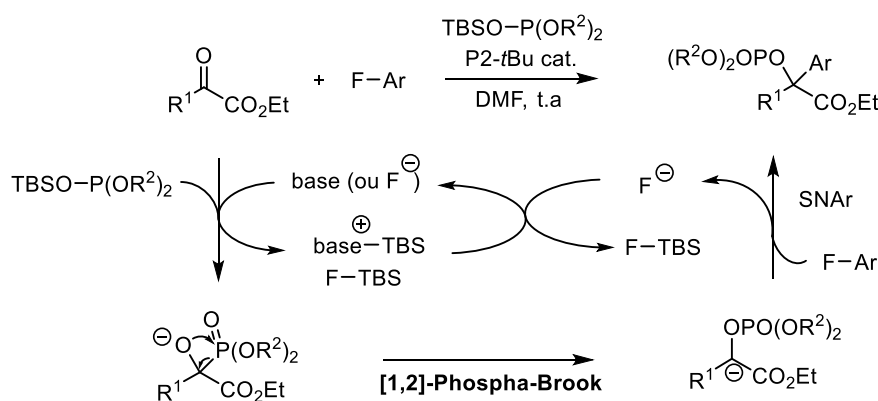
Schéma III-13. Système réactionnel pour l'arylation des \alpha -cétoesters
