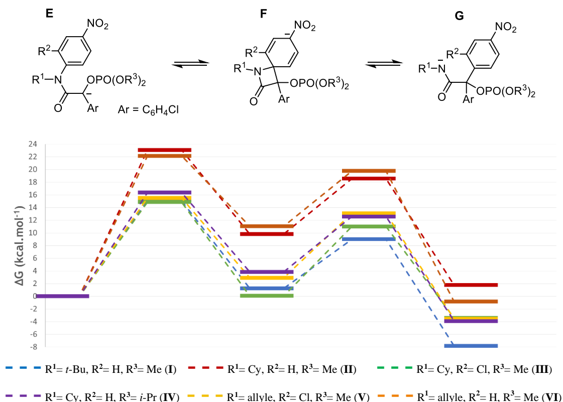
Figure III-3. Profils énergétiques associés au réarrangement de Truce-Smiles pour les substrats modèle
