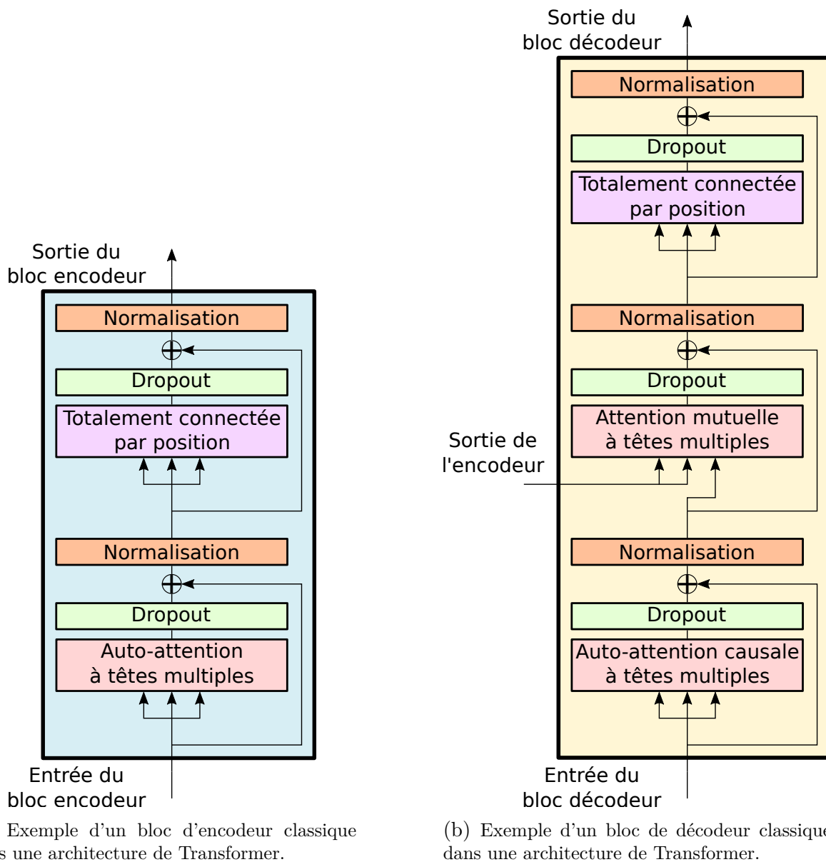
FIGURE 3.5 – Schéma d'un bloc d'encodeur (a) et d'un bloc de décodeur (b) typiquement utilisés dans les architectures de Transformer.
