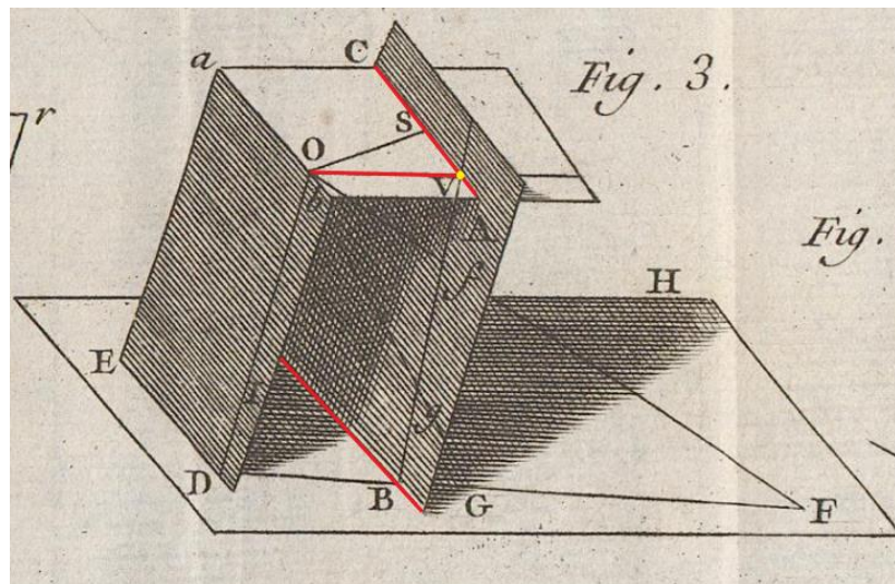
Illustration 33. Figure représentant les différentes lignes constituant la représentation en perspective d'après Taylor. Traduction française du traité de Taylor, 1757, pl. 1.
