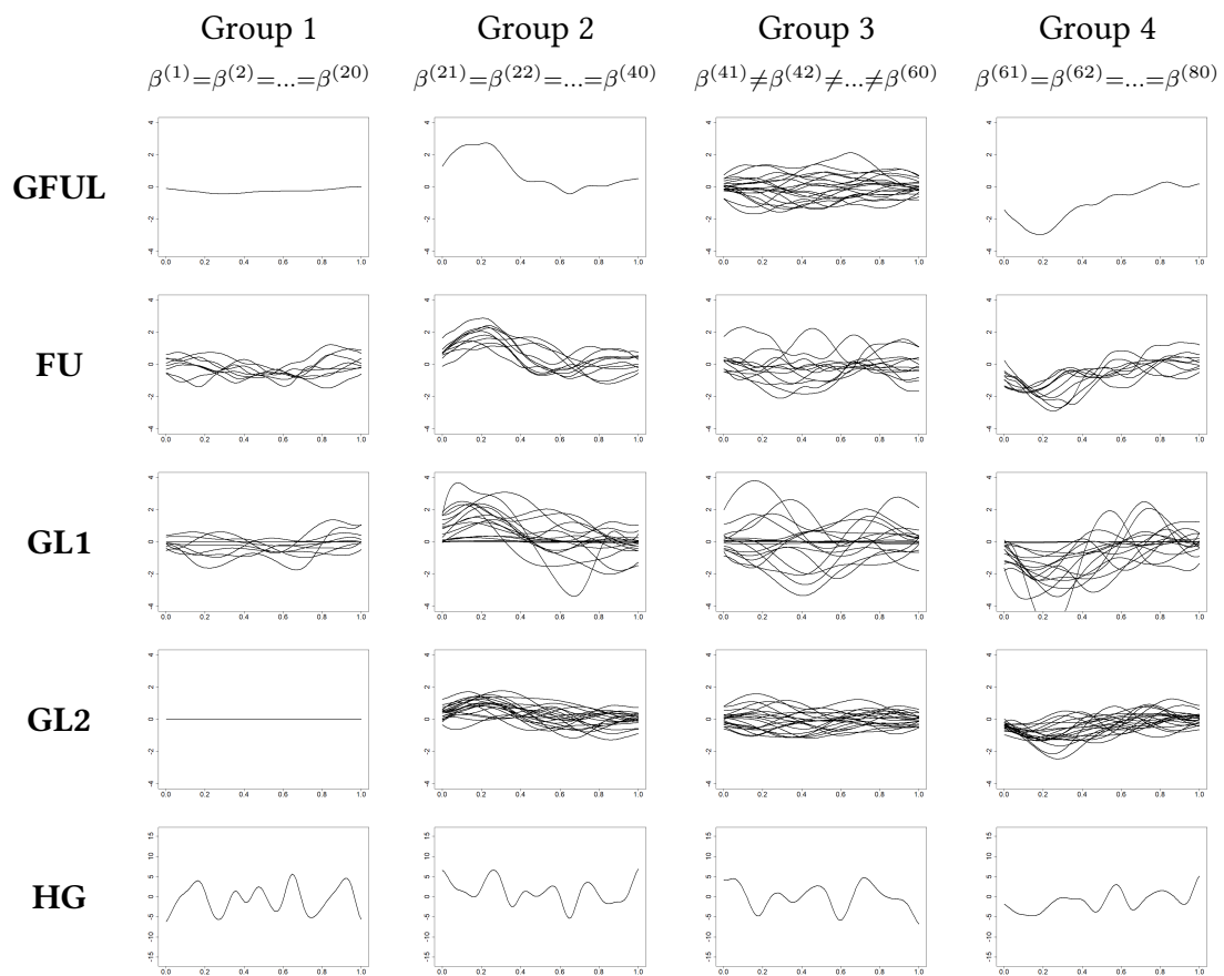
FIGURE 4.7 – Scénario 2- Les estimations de \beta par les différentes méthodes (première expérience).
