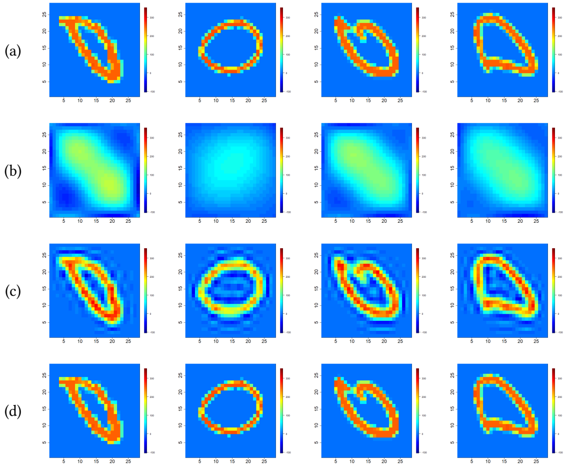
FIGURE 1.2 – Reconstitutions fonctionnelles des observations en (a) à l’aide de B-Splines composée de 4, 16 et 28 fonctions respectivement représentées par (b), (c) et (d).
