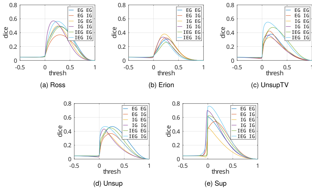
FIGURE 5.5 – Robustesse d'IEG. Dice en fonction du seuil ( thresh ) pour différentes contraintes sur les images de tumeurs en 2\text{mm}^3 . Dans la légende, la méthode de gauche est celle de l'entraînement et celle de droite celle utilisée à l'inférence.
