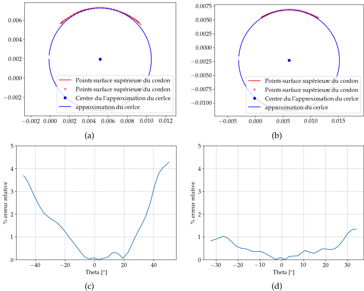
FIGURE 3.11 – Approximation d'un passe de cerce sous la surface libre du bain de fusion; (a) courant de 150 A, (b) courant de 180 A. Pourcentage de l'erreur relative du rayon du cerce entre expérimental et théorique; (a) courant de 150 A, (b) courant de 180 A.
