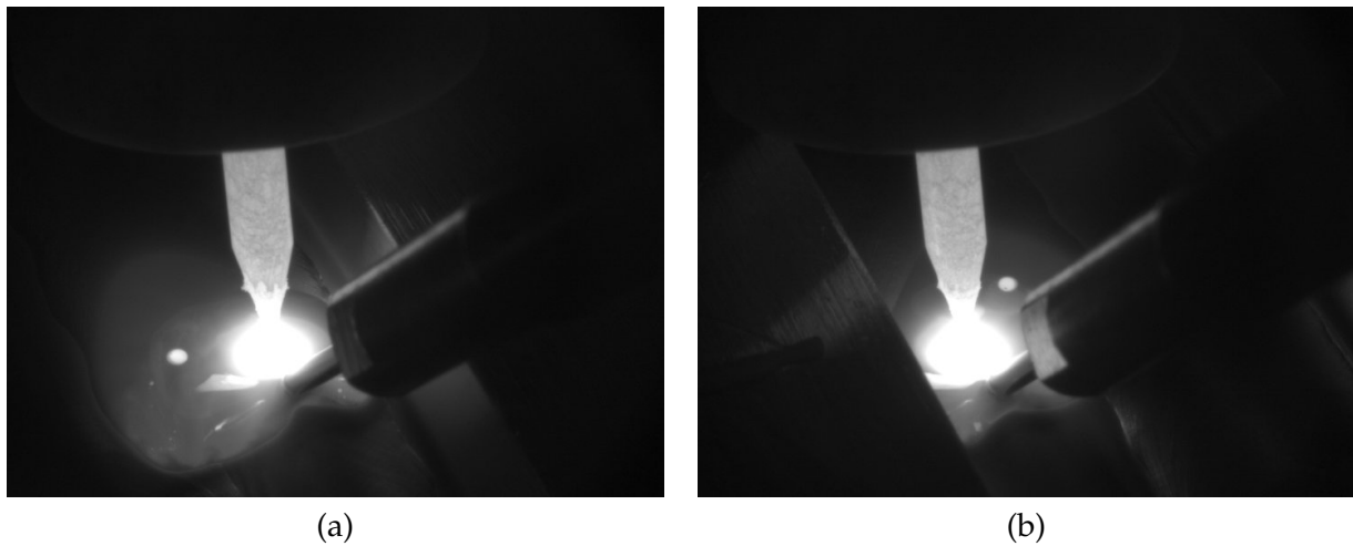
FIGURE 5.6 – (a) Image acquise lors du soudage d'une passe à droite du chanfrein (b) image acquise lors du soudage d'une passe à gauche du chanfrein.
