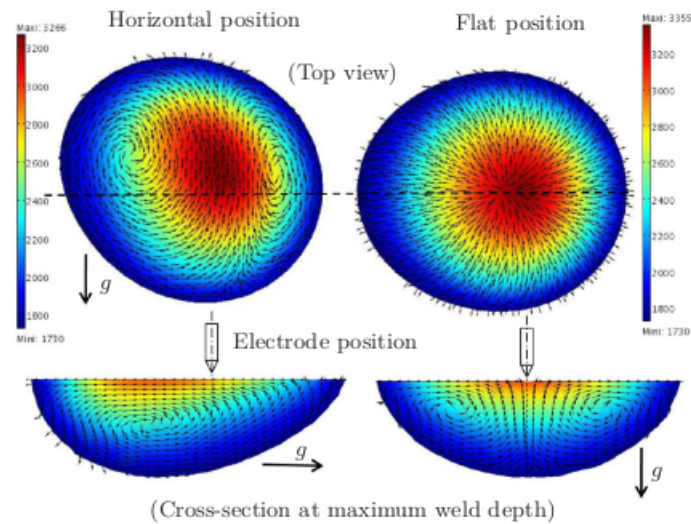
FIGURE 1.19 – Influence de la position de soudage sur la force de flottabilité et l'écoulement pour 150 A de courant d'après Traidia [131].
