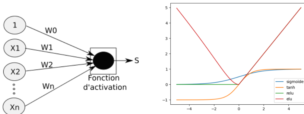
FIGURE 3.18 – (a) Architecture d'un perceptron; (b) exemple de fonction d'activation.
