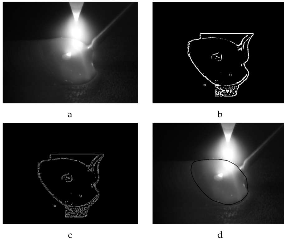
FIGURE 2.22 – (a) Rectification de l'image à partir de la mire de calibration, (b) utilisation du filtre à seuil adaptatif, (c) utilisation du filtre de Canny, (d) détection des bords par la méthode des formes \alpha couplée à la théorie des graphes.
