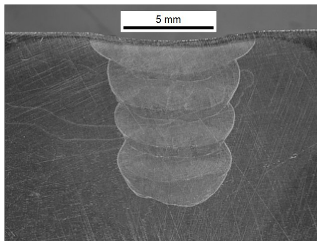
FIGURE 4.4 – Macrographie d'une opération de soudage pour le remplissage du chanfrein étroit.
