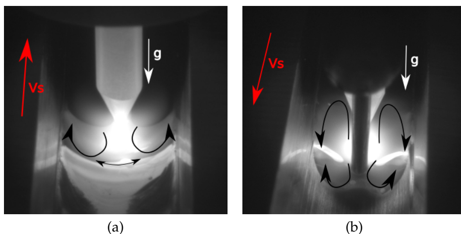
FIGURE 4.7 – (a) Capture d'une image en face arrière du bain de fusion en position à plat, (b) capture d'une image en face avant du bain de fusion en position à plat.
