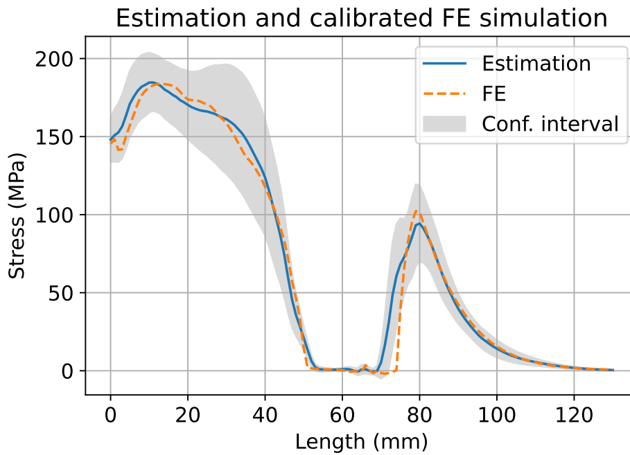
FIGURE 1.41 – Estimation de la contrainte principale maximale, simulation éléments finis et l'intervalle de confiance à partir des données du côté de la caméra infrarouge.
