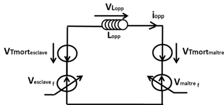
Figure 16 - Schéma de principe présentant les chutes de tension amenées par la mise en place de temps mort.
