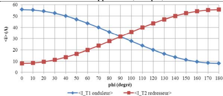
Figure 40 - Exemple de tracé présentant le courant moyen (noté \langle i \rangle ) en fonction du déphasage courant/tension aux bornes de l'inductance d'opposition (noté \phi ), avec m_a=0,95 et I_{\text{opp\_max}}=200\text{A} .
