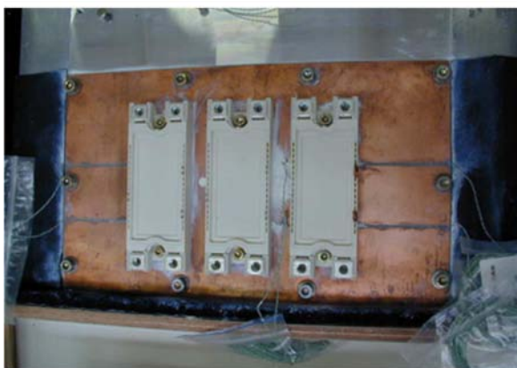
(c) ensemble plaque de refroidissement, semelle d'interface, modules de puissance, thermocouples, mousse isolante et boîte isolante.
