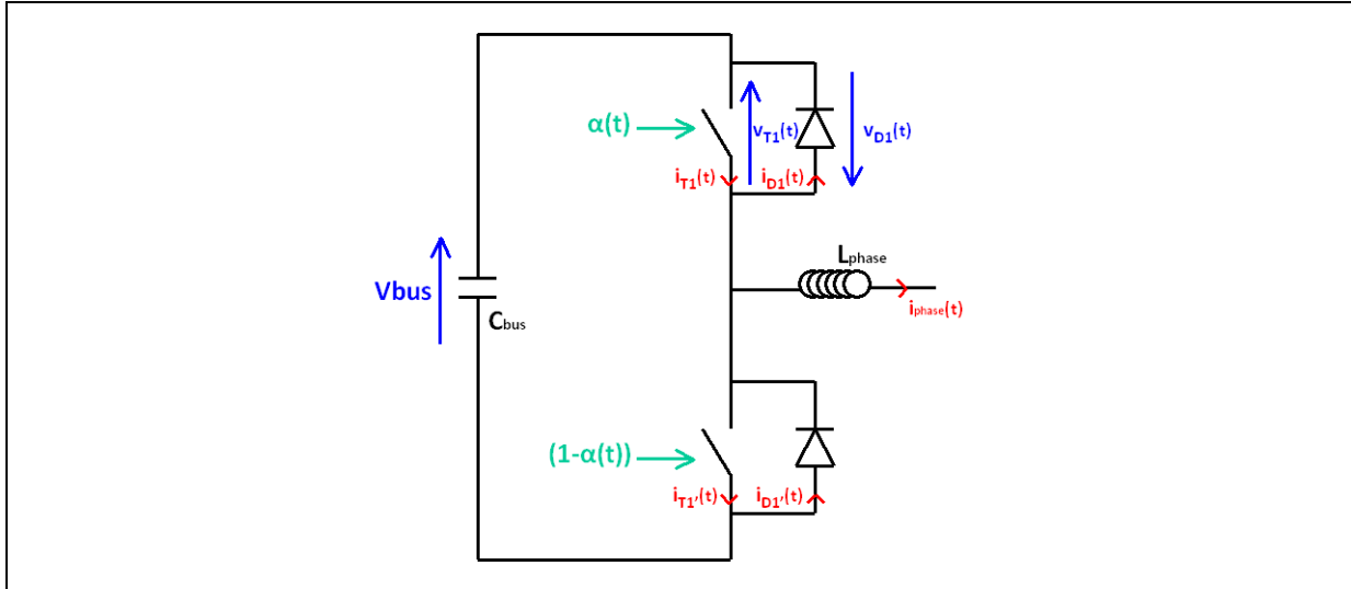
Figure 38 - Schéma de principe d'un bras onduleur et conventions de mesures.
