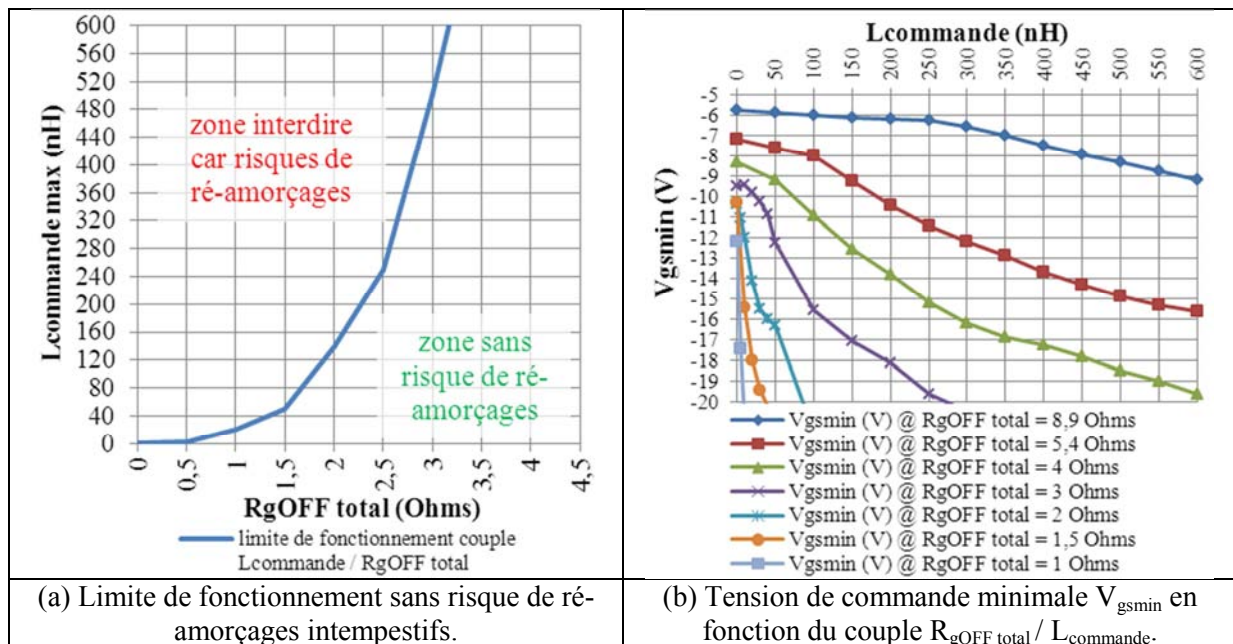
Figure 17 - Résultats des simulations pour le blocage du module MOSFET-SiC ROHM BSM100D12P1C004, pour V_{bus} = 600V , I_{ds} = 200A , T_j = 25^\circ C , V_{gs} = +20V/-5V , pour différentes valeurs d'inductance de la boucle de commande L_{commande} et différentes valeurs de résistances de grille R_{gOFF\ total} .
