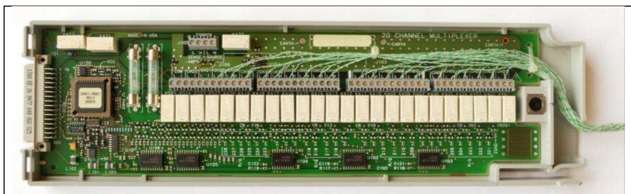
Figure 20 - Photo d'un rack d'acquisition de mesures de l'appareil Agilent 34972A sur lequel sont branchés plusieurs thermocouples de type K.
