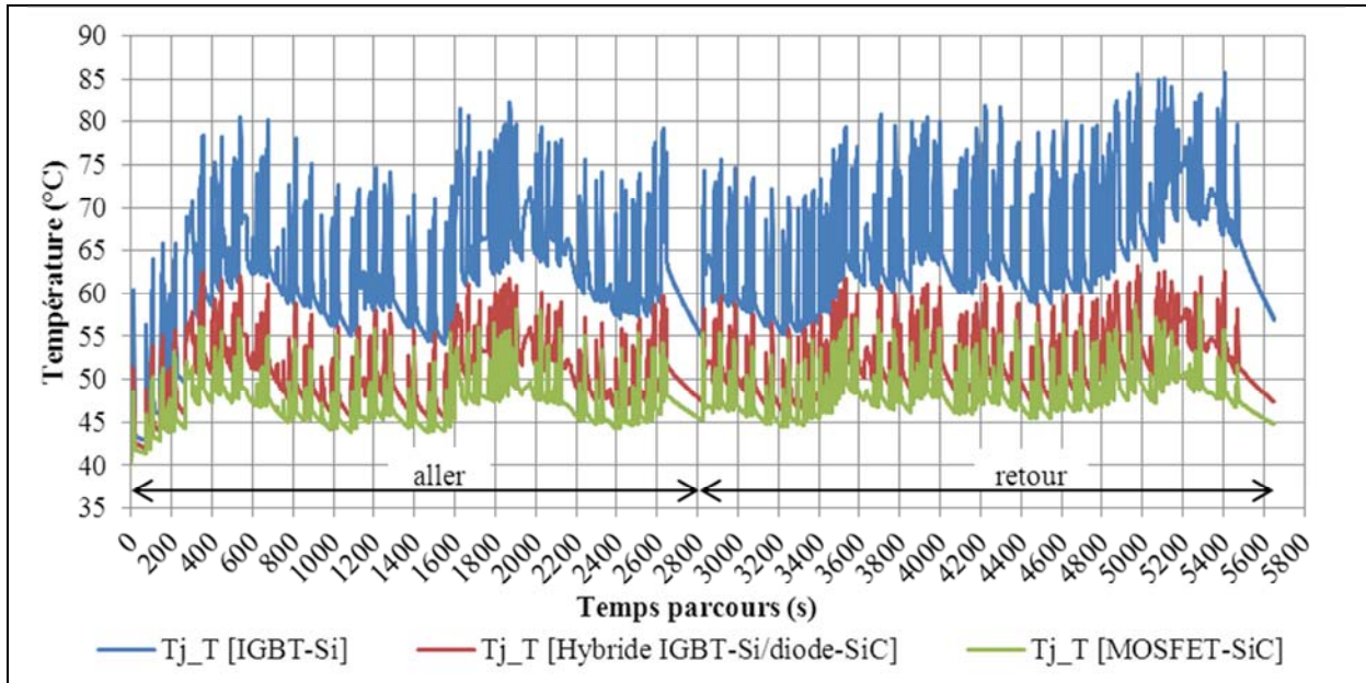
Figure 8 - Relevés des températures de jonction de la partie transistor en fonction du temps de parcours. Comparaison des IGBT-Si actuels (CM800DZ-34H-205) avec les MOSFET-SiC (3 packs E3XL 1700V 250A) et avec le pack hybride (CMH1200DC-34S).
