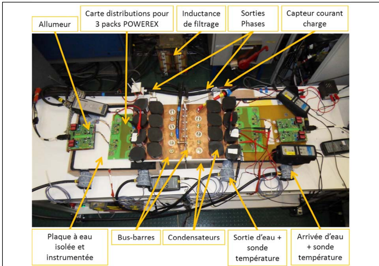
Figure 48 - Images présentant une description de la partie pont en H du banc d'essai (ici, dans une première configuration permettant de tester des packs MOSFET-SiC POWEREX).
