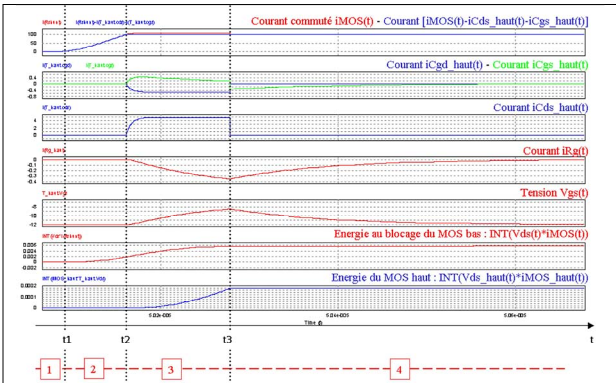
Figure 5 - Résultats de simulation à l'amorçage du MOSFET de puissance. Impacts de l'ajout du MOSFET du haut dans le montage.
