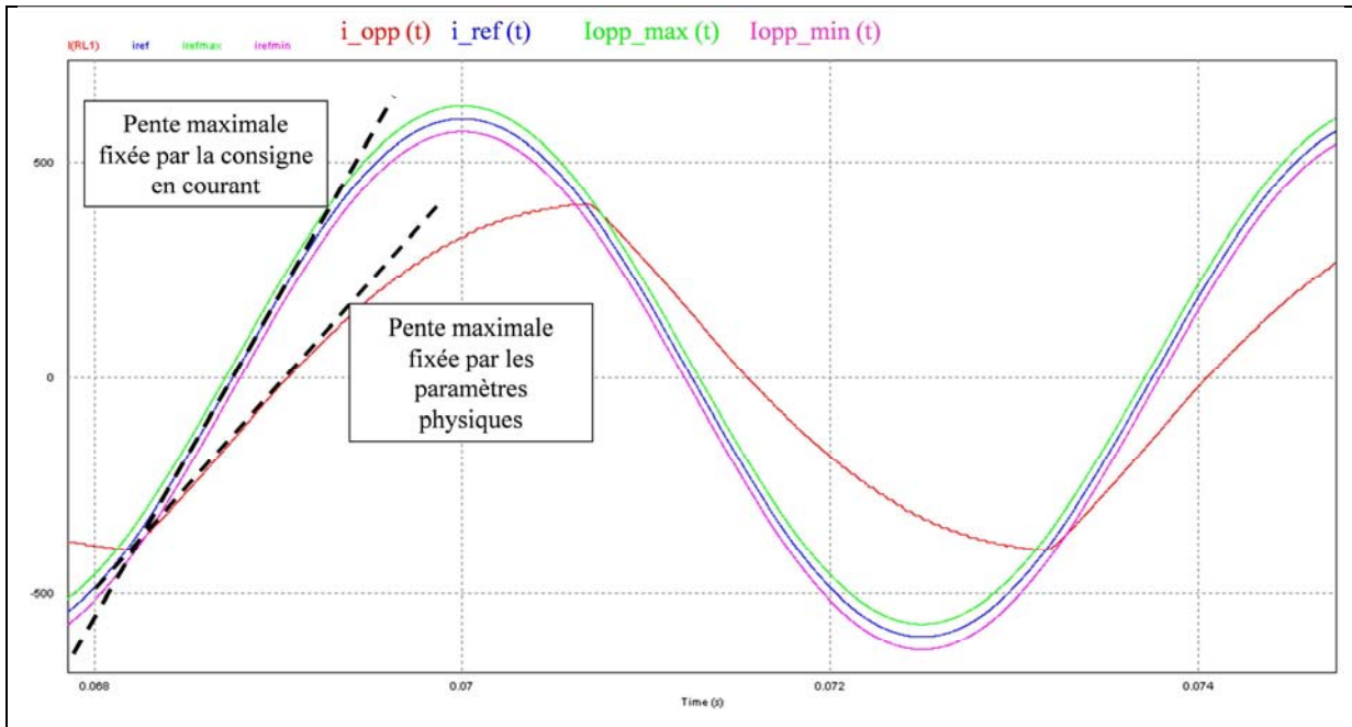
Figure 26 - Relevés PSIM® du courant de consigne et du courant mesuré, ainsi que les bornes minimum et maximum du courant, dans une situation où le choix de la valeur de l'inductance d'opposition n'est pas adapté.
