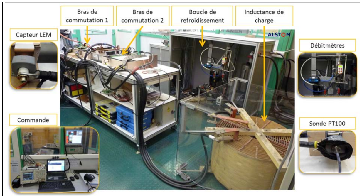
Figure 46 - Images présentant une description du banc d'essai mis en œuvre.
