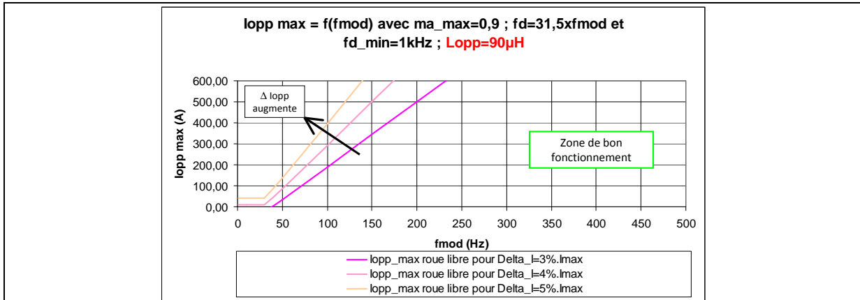
Figure 30 - Graphe du courant de consigne maximum en fonction de la fréquence de modulante, pour une valeur de l'inductance d'opposition de 90\mu H (variation de \Delta I_{opp} ).
