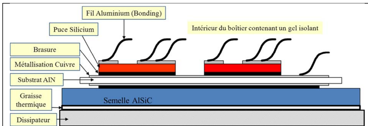
Figure 7 - Coupe schématique d'un pack IGBT monté sur un dissipateur [10].
