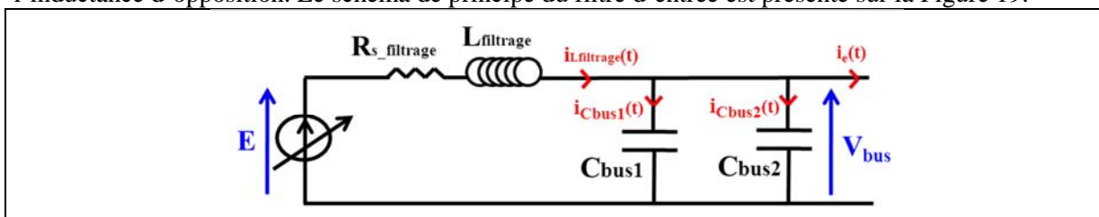
Figure 19 - Schéma de principe du filtre d’entrée.
