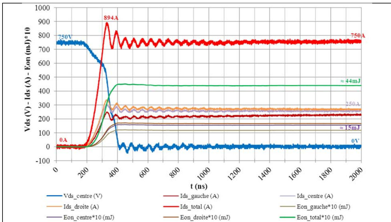
Figure 5 - Formes d'ondes à l'amorçage de 3 packs E3XL MOSFET-SiC 1700V 250A (interrupteur Bas), pour V_{bus} = 750\text{V} , I_{ds} = 750\text{A} , T_j = 150^\circ\text{C} , V_{gs} = +20\text{V}/-5\text{V} .
