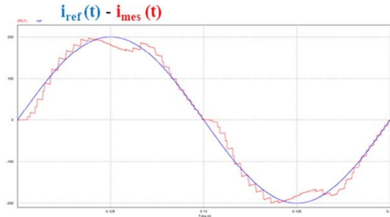
Figure 15 - Formes d'ondes obtenues sous PSIM ® du courant dans l'inductance d'opposition et sa consigne lorsque le déphasage est nul, f_d=2,5kHz et le temps mort valant 10\mu s .
