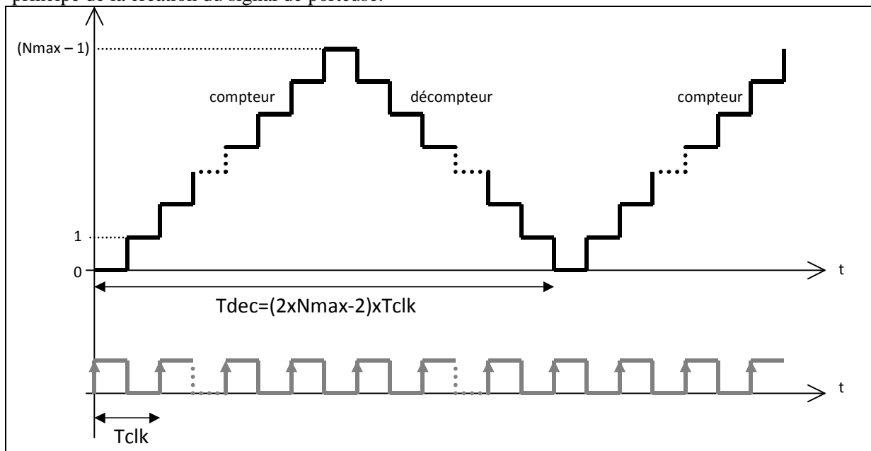
Figure 34 - Schéma simplifié présentant le principe de la création du signal porteuse (numérique).
