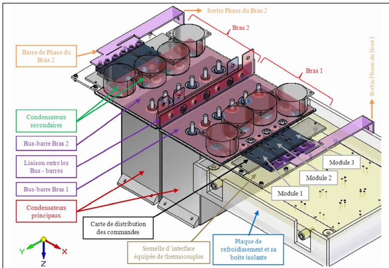
Figure 24 - Conception mécanique finale retenue pour le banc d'essai « méthode d'opposition » (logiciel Solid Edge®), permettant la mise en œuvre de 3 modules de puissance MOSFET-SiC en parallèle.
