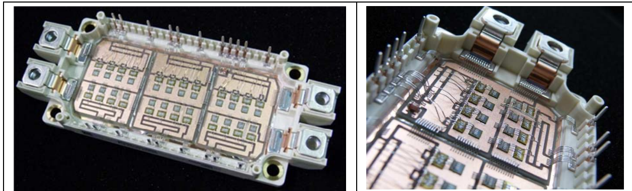
Figure 2 - Pack E3XL MOSFET-SiC 1700V 250A réalisé dans le cadre d'une collaboration entre ALSTOM, ROHM et DANFOSS.
