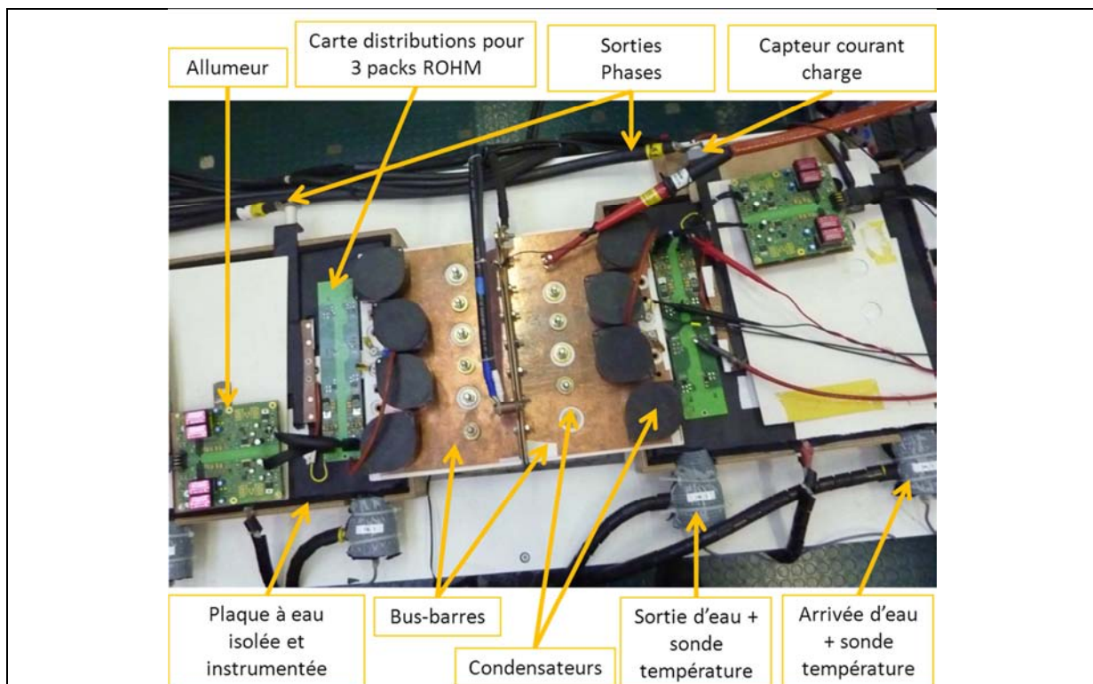
Figure 49 - Images présentant une description de la partie pont en H du banc d'essai (ici, dans une première configuration permettant de tester des packs MOSFET-SiC ROHM ou IGBT-Si F100R12MT4).
