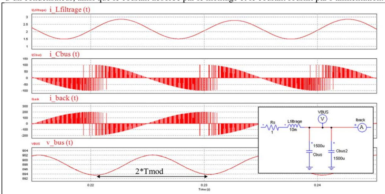
Figure 18 - Relevés de simulation PSIM® présentant notamment la tension et le courant dans les condensateurs de filtrage.
