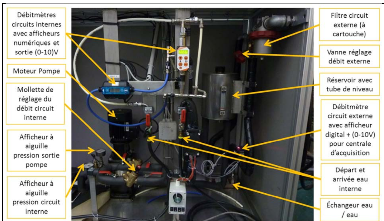
Figure 47 - Images présentant l'intérieur de la boucle de refroidissement.
