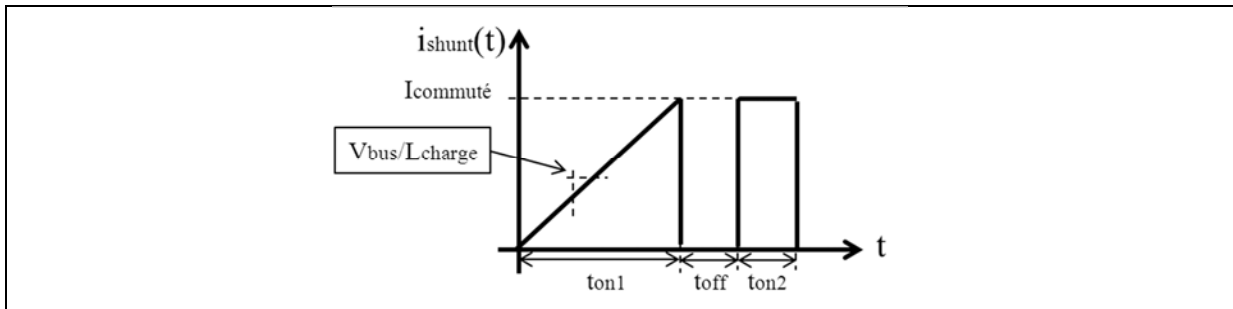
Figure 7 - Hypothèse sur la forme d'onde du courant dans le Shunt lors d'un fonctionnement « double-pulse ».
