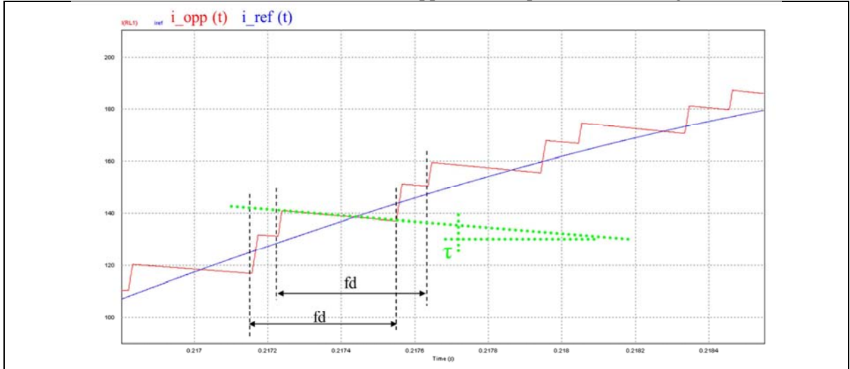
Figure 24 - Formes d'ondes du courant de référence et du courant mesuré dans l'inductance d'opposition, à l'échelle de la fréquence de découpage.
