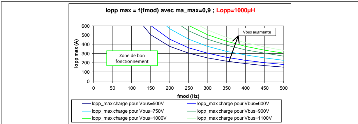
Figure 29 - Graphe du courant de consigne maximum en fonction de la fréquence de modulate, pour une valeur de l'inductance d'opposition de 1mH (variation de V_{bus} ).
