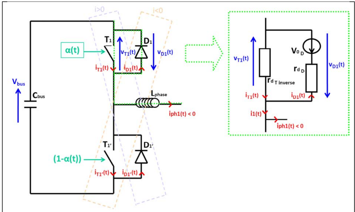
Figure 9 - Schéma de principe d'un bras onduleur et conventions de mesures. Explication de la phase de répartition du courant avec le MOSFET bidirectionnel en courant.
