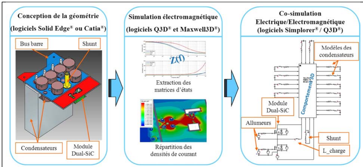
Figure 20 - Exemple d'utilisation des modèles et des simulations dans le but de concevoir un banc de test [8].
