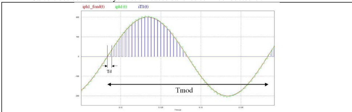
Figure 39 - Formes d'ondes des courants dans un bras d'onduleur.
