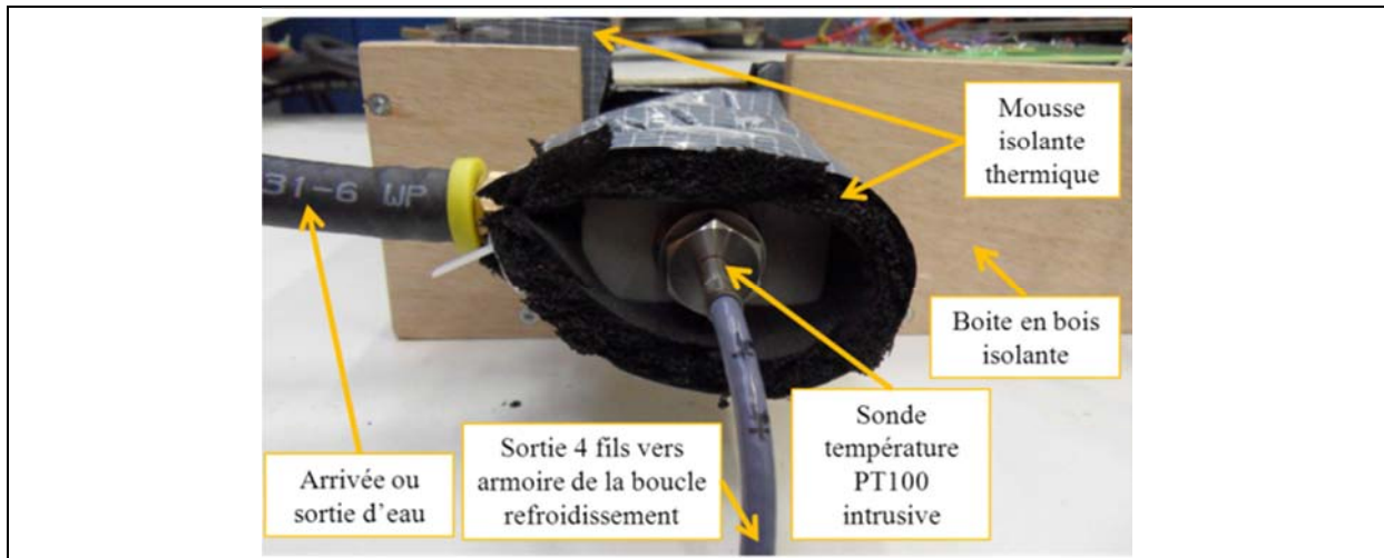
Figure 17 - Sonde de température PT100 installée en entrée ou en sortie d'une plaque de refroidissement.
