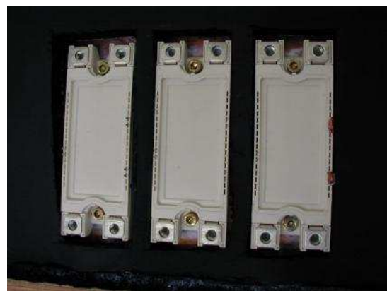
(d) isolation supérieure de l'ensemble de la plaque de refroidissement.
