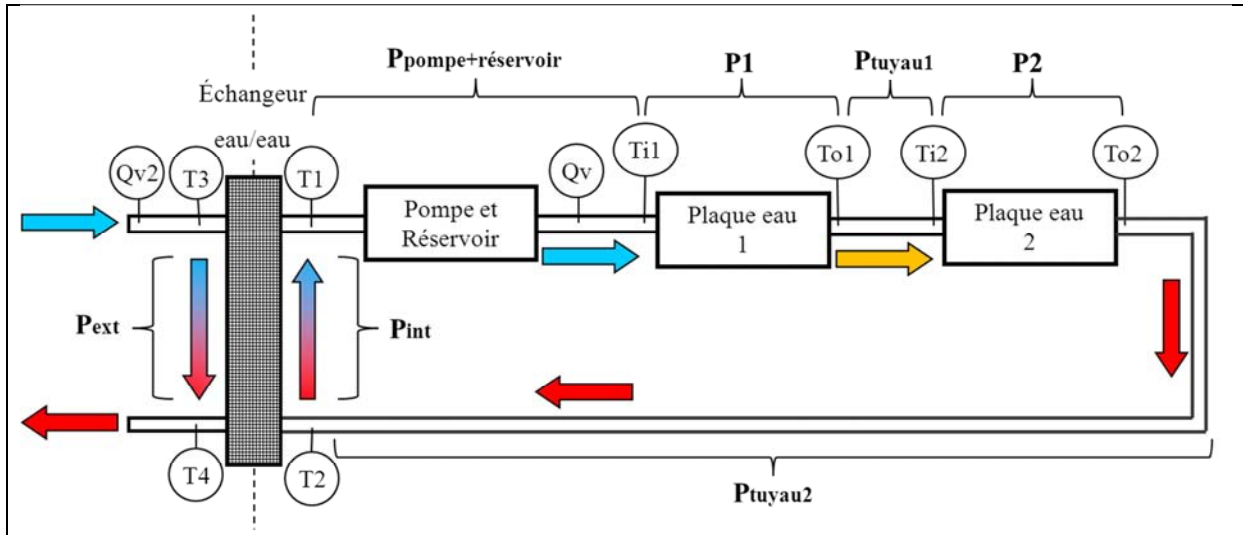
Figure 15 - Schéma de principe de l'ensemble du système de refroidissement.
