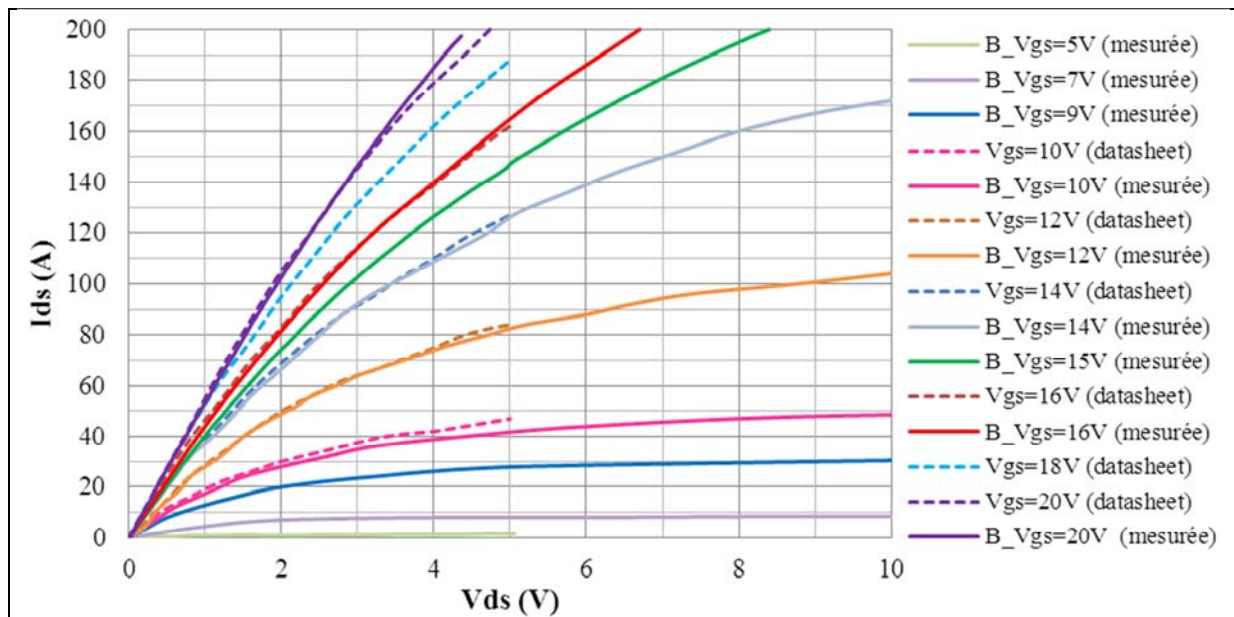
Figure 2 - Caractéristiques statiques en polarisation directe du MOSFET-SiC ROHM BSM100D12P1C004 (n°149A000010R, interrupteur Bas), à la température de 25°C pour différentes valeurs de tension de grille V_{gs} .
