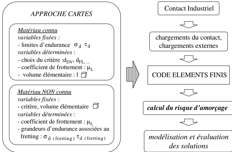
Figure 81 : Apports de la méthodologie « carte » pour identifier les variables nécessaires à la modélisation de l'amorçage induit par fretting.
