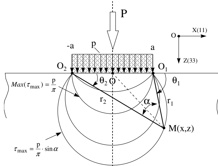
Figure A3-3 : Contact bidimensionnel du contact plan-plan (indenteur souple).
