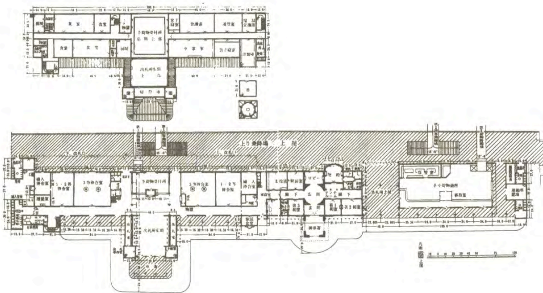
Figure 77 (b) : Plans du rez-de-chaussée et du 1 er étage de la 2 e gare de Kyôto édifïée en 1914
