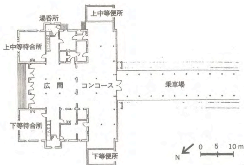
Figure 67 (c) : Plan du rez-de-chaussée de la gare de Shinbashi édiflée à Tôkyô en 1872
