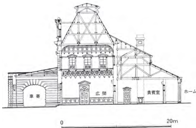
Figure 76 (c) : Coupe transversale de la 2 e gare d'Ôsaka (Umeda) achevée en 1899
