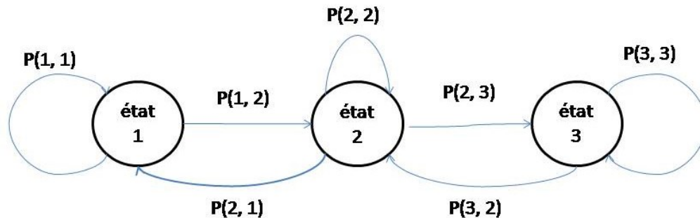
Figure 1 Matrice et graphique d'une chaîne de Markov dont l'espace d'état discret compte 3 états possibles.
