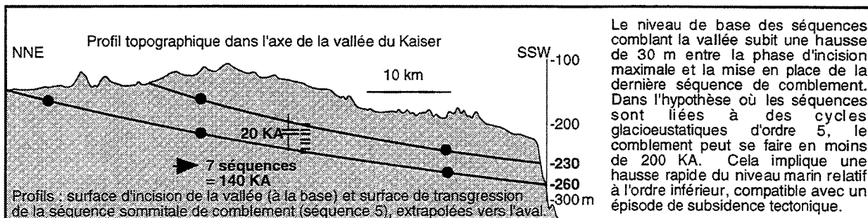
Fig. 139 : Niveaux de base des séquences de comblement de la vallée du Kaiser.
