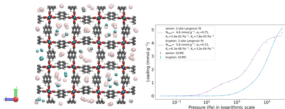
FIGURE R3 – WOJJOV : Représentation d'un MOF [Al(OH)(1,4-NDC)] \cdot 2(H_2O) où NDC signifie naphthalenedicarboxylate. Code couleur : Cu en cyan foncé, C en gris, O en rouge, H en blanc ; Xe en rose et Kr en cyan clair. Sur la droite, les isothermes corps pur du xénon et krypton à 298 K ainsi qu'un modèle d'isotherme à deux sites.
