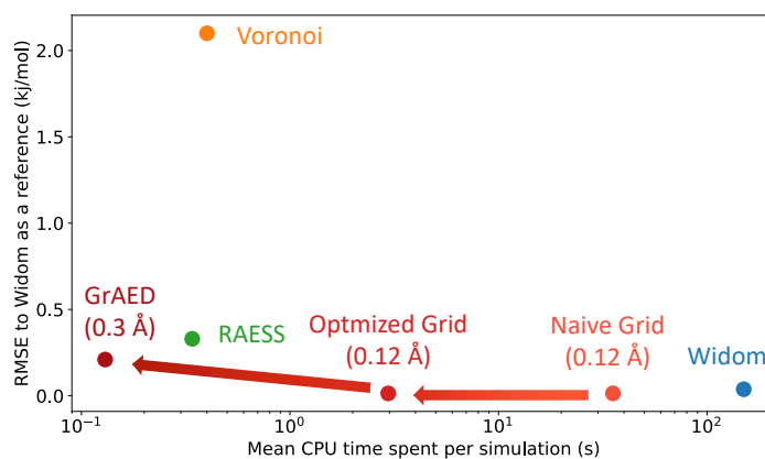
FIGURE R4 – Comparaison de la racine de l'erreur quadratique moyenne sur l'enthalpie d'adsorption du xénon et le temps de simulation par structure pour différentes méthodes d'échantillonnage sur la base de données CoRE MOF 2019 (pour une taille de pore supérieure à 3.7 Å).
