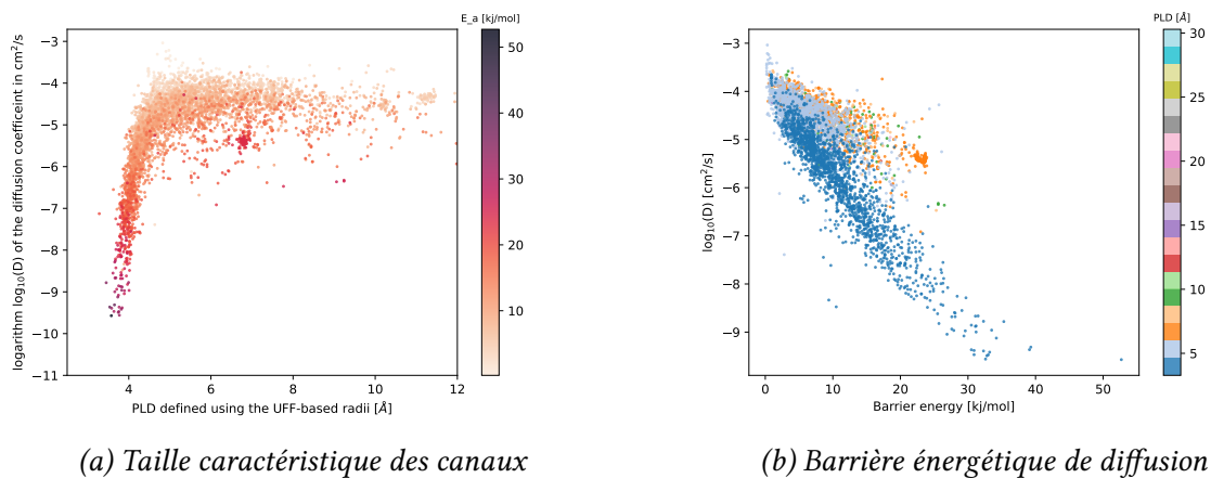
FIGURE R7 – (a) Graphe comparant le logarithme base 10 du coefficient de diffusion du xénon à la taille des canaux mesurée par le diamètre minimal du canal (PLD, en anglais), et les points sont étiquetés par les énergies de barrière. (b) Graphe comparant le logarithme base 10 du coefficient de diffusion du xénon à la barrière énergétique de diffusion, les points sont étiquetés par le diamètre PLD.
