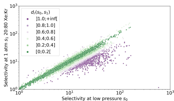
FIGURE R2 – Sélectivité à 1 atm de pression en fonction de la sélectivité à basse pression pour une composition 20:80 Xe/Kr. Les points sont étiquetés selon la différence relative entre les deux sélectivités. Les points violets ont une grande différence relative entre les sélectivités.
