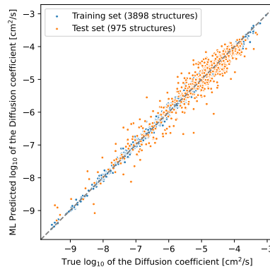
FIGURE R8 – Comparaison du \log_{10} du coefficient de diffusion du xénon prédit par le modèle ML et les valeurs simulées par dynamique moléculaire. La racine de l'erreur quadratique moyenne sur le logarithme base 10 vaut 0.25.
