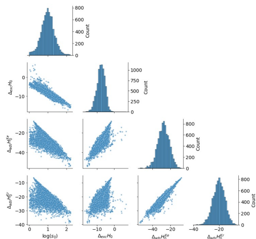
FIGURE R1 – Pour 8 401 MOFs avec une sélectivité Xe/Kr favorable ( s_0 > 1 ), pair-plots entre les différentes grandeurs \log(s_0) , \Delta_{exc}H_0 , \Delta_{ads}H_0^{Xe} et \Delta_{ads}H_0^{Kr} (les enthalpies sont en \text{kJ mol}^{-1} ) en dehors de la diagonale et la distribution de chaque grandeur sur la diagonale.
