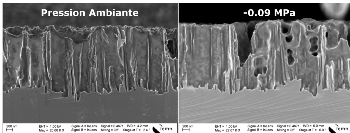
Figure A. 14 Imprégnations par coulage de nanofils de silicium avec du PEDOT:PSS (PH500 Clevis Heraeus, 1 - 1.3 % de solide) réticulé avec 1 %pds de GOPS : impact de la pression d'imprégnation visualisé par MEB. Paramètres de fabrication : température ambiante pour l'imprégnation, temps d'imprégnation de 2 h 45, à pression ambiante ou -0.09 MPa.
