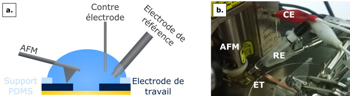
Figure 2. 13 Expérience d'AFM liquide sous activation permettant de mesurer l'évolution de la topographie et de l'épaisseur du film polymère en fonction de la tension électrique : schéma de fonctionnement (a), photo du dispositif (b) ET représente l'électrode de travail, RE la référence et CE la contre.
