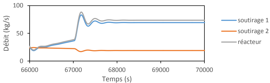
Figure 27 : Exemple de contrôle de la température en sortie de mélangeur du cycle de Rankine de l'intégration 1 (phase 3) en faisant varier le débit de soutirage
