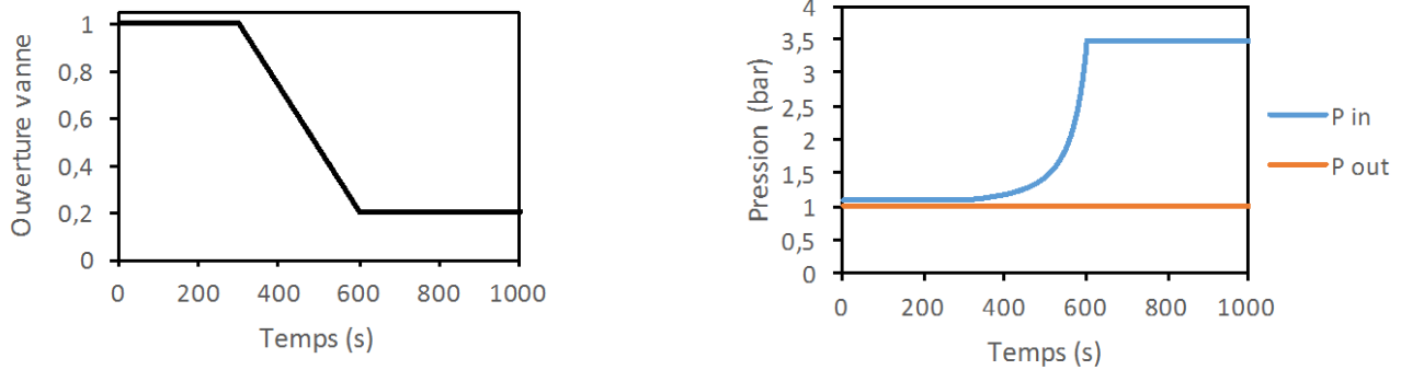
Figure 19 : Variation de l'ouverture de la vanne et de la pression du fluide en entrée en fonction du temps
