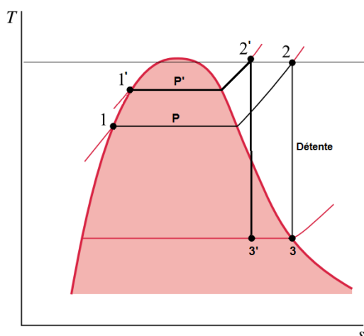
Figure 20 : Diagramme T-S montrant les effets de l'augmentation de pression avec la même température de surchauffe
