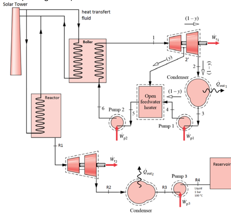
Figure 10 : Schéma représentant la configuration de l'intégration 3 – turbine en charge
