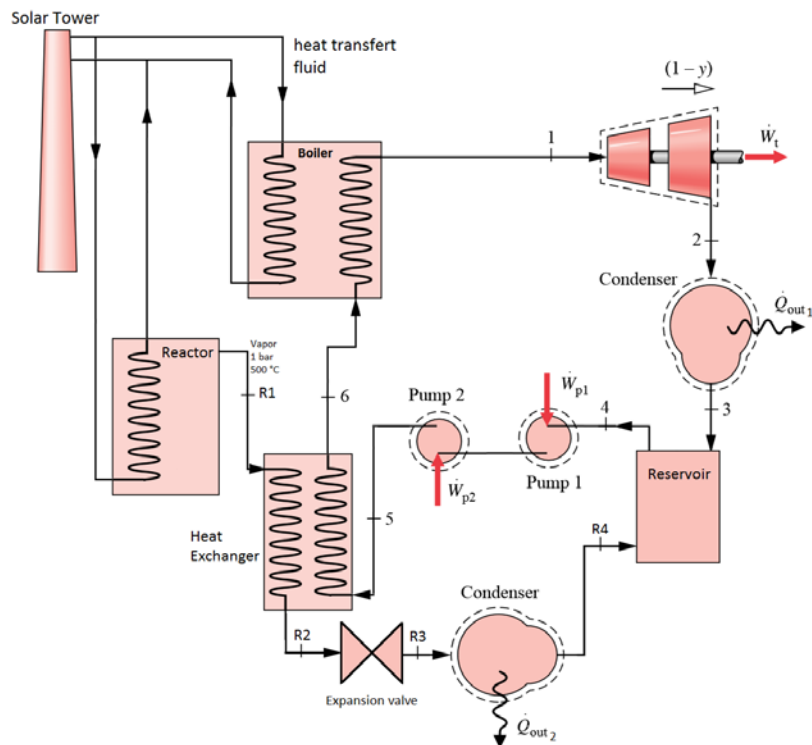
Figure 8 : Schéma représentant la configuration de l'intégration 2 – massive en charge
