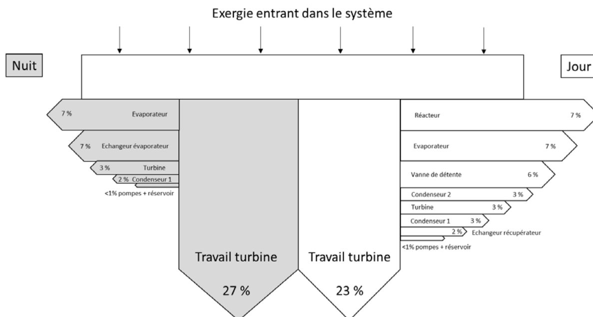
Figure 34 : Bilan exergetique de l'intégration 2
