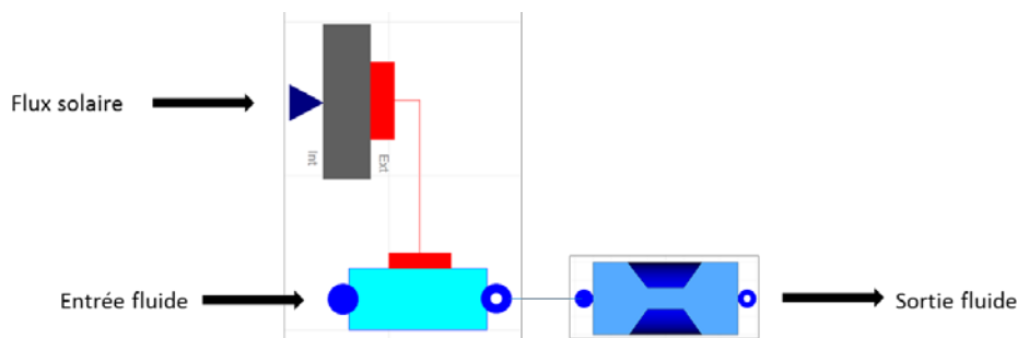
Figure 26 : Schéma représentant les composants du récepteur solaire
