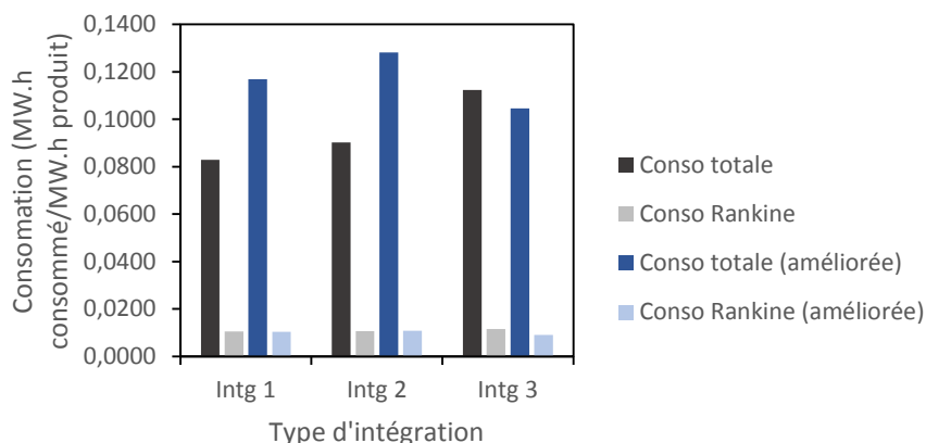
Figure 44 : Consommation des trois intégrations ramenée en \text{MW.h}_{\text{consommé}}/\text{MW.h}_{\text{produit}}
