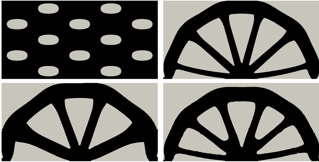
FIGURE 1.8 – Illustration de la Section 1.6 : Initialisation et formes finales pour l’optimisation d’une arche pour, respectivement, la méthode de Gauss-Newton, l’algorithme du gradient et un algorithme de régularisation de la vitesse.
