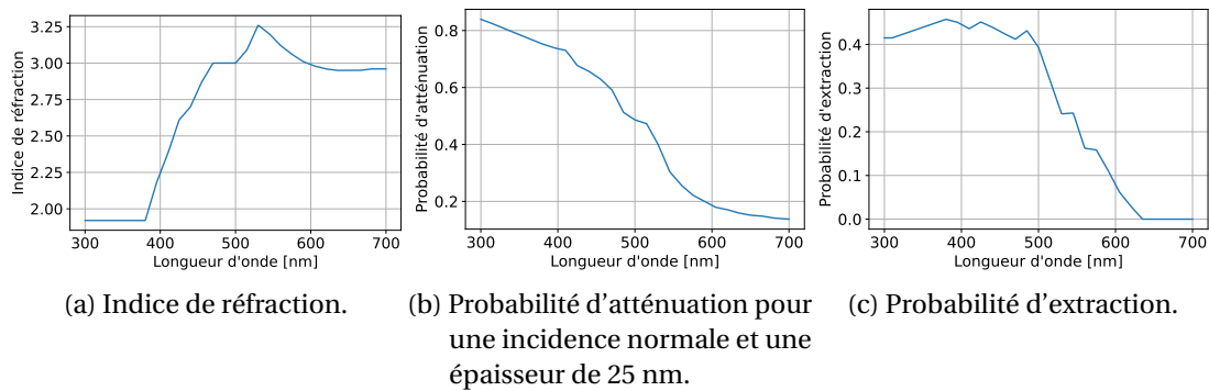
FIGURE 4.3 – Propriétés de la photocathode bialcaline bleue utilisée [MOTTA et SCHÖNERT 2005]. L'indice de réfraction n'étant défini qu'à partir de 380 nm, nous le considérons comme constant pour des longueurs d'onde inférieures.
