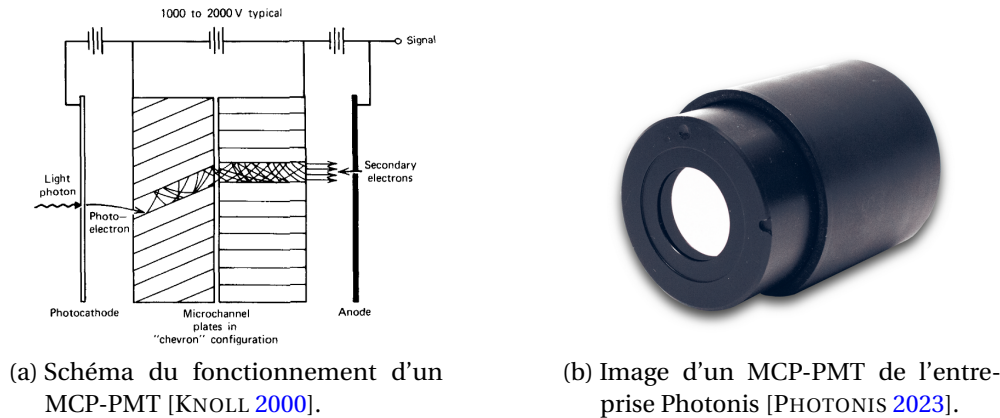
FIGURE 1.12 – Illustration (a) du fonctionnement du MCP-PMT et (b) photographie d'un MCP-PMT.
