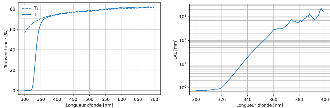
(a) Transmittance théorique T_s (traitillé) et mesurée T (trait continu) à travers un cristal nu de 5 mm d'épaisseur. (b) LAL obtenue à partir de l'Eq 3.2 en prenant T et T_s les transmittances mesurée et théorique présentées sur (a).
