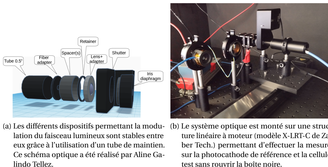
FIGURE 3.13 – (a) Schéma optique et (b) photographie du banc optique permettant la mesure de la PDE à travers la photocathode de référence et les cellules tests.
