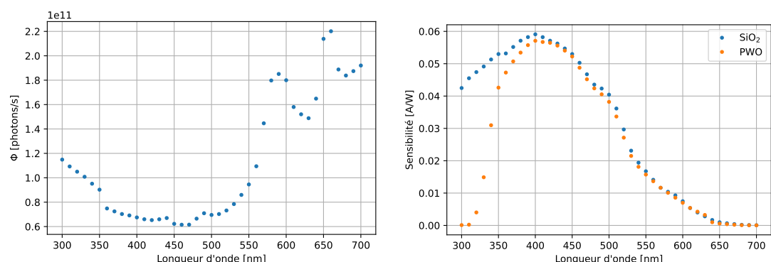
(a) Flux de particules par unité de temps calculé à partir de l'intensité de courant mesurée et de la sensibilité de la photocathode de référence. (b) Sensibilité mesurée pour les cellules tests.
