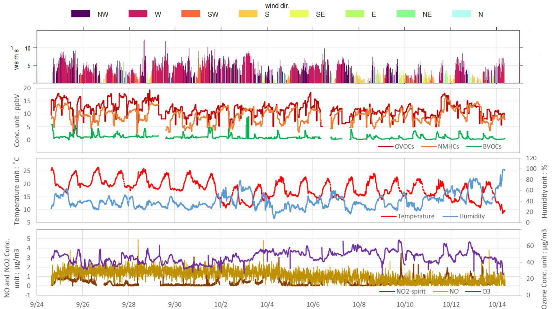
Figure 5-4 Séries temporelles des concentrations moyennes de COV (ppbv), de NO ( \mu\text{g}/\text{m}^3 ), de NO 2 ( \mu\text{g}/\text{m}^3 ), d'ozone ( \mu\text{g}/\text{m}^3 ), d'humidité relative (%) et de la température ( ^{\circ}\text{C} ) pendant la période étudiée, avec les paramètres météorologiques (vitesse du vent en m/s, direction du vent selon un code couleur).
