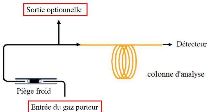
Figure 2-9 Désorption du piège
