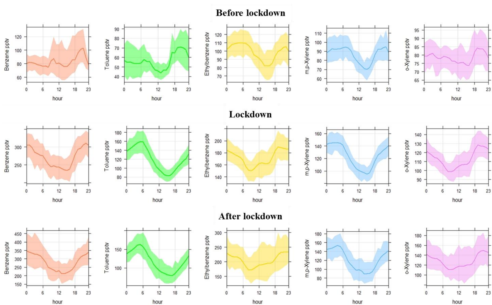
Figure 4-10 Séries de variations diurnes des rapports de mélange du benzène, du toluène, de l'éthylbenzène, du m,p-xylène et de l'o-xylène avant, pendant et après le confinement. Les zones d'ombre représentent les écarts type
