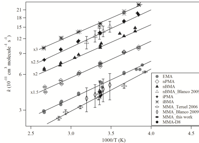
Figure 3-3 Constantes de vitesse k_{1\_OH} et k_{6\_OH} en fonction de 1/T . Les droites d'Arrhenius obtenues entre 257 K et 376 K pour chaque ester. Les barres d'erreur des points individuels sont de 2\sigma . Les barres d'erreur des valeurs (Blanco et al., 2009b; Teruel et al., 2006) ont été publiées par les auteurs. Pour une meilleure vue d'ensemble, les k(T) obtenus pour la nPMA, la nBMA, l'iPMA et l'iBMA ont été multipliés par 1,5, 2, 2,5 et 3, respectivement.
