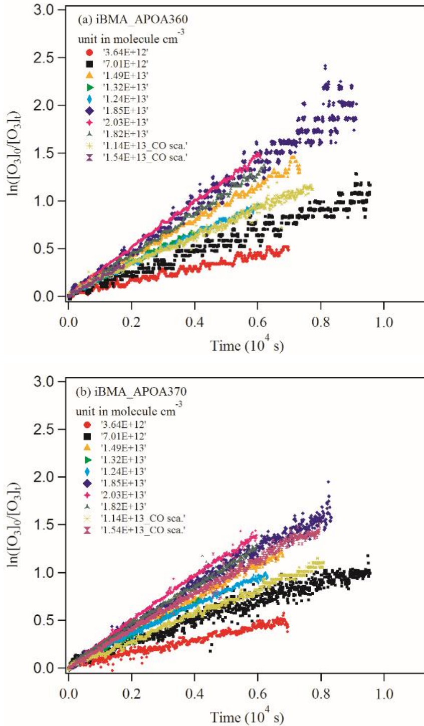
Figure 3-11 Exemple de graphiques de la consommation d' \text{O}_3 en fonction du temps de réaction en présence de différentes concentrations d'iBMA en utilisant deux types de moniteur de \text{O}_3 (APOA360 et APOA370). Note : CO sca. = expériences en présence de CO comme piègeur.
