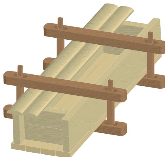
Figure II.46 : Schéma simplifié du système de fermeture « en étau » (S. Duchesne).
