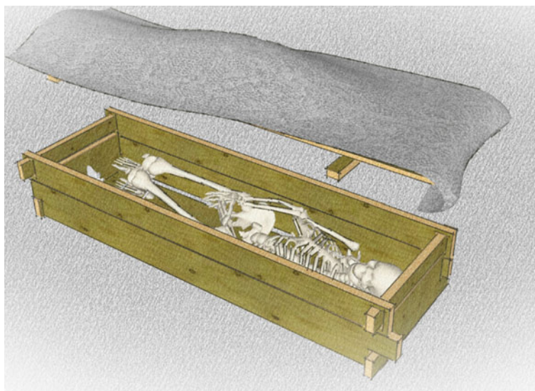
Figure II.45 : Restitution du mode d'assemblage du coffre de la tombe de Ebuguey 1 (Indighirka) (évocation : N. Sénégal).
