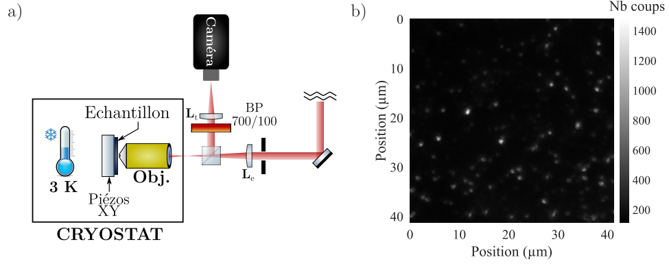
FIGURE 2.6 – Imagerie en champ large de molécules à température cryogénique. a) Montage expérimental d'imagerie en configuration d'épifluorescence. La lentille L_e sert à focaliser le faisceau au niveau du plan focal arrière de l'objectif. En sortie de l'objectif le faisceau est donc en principe collimaté et excite l'échantillon en champ large. Sa focale est de f_e = 150 mm, de sorte que la taille du champ excité soit d'environ 70 \times 70 \mu\text{m} . La fluorescence, collectée par le même objectif, est réfléchiée par un cube séparateur 50/50 et est conjuguée au capteur d'une caméra par une lentille dite "tube" L_t de focale f_t = 400 mm. La fluorescence est filtrée spectralement par un filtre bandpass centré sur 700 nm avec une fenêtre passante large de 100 nm afin de se débarrasser de l'intensité du laser réfléchiée par l'échantillon; b) Image d'épifluorescence en champ large ( P_{laser} = 2 mW). L'excitation est résonante avec la ZPL et le temps d'intégration vaut 1 s.
