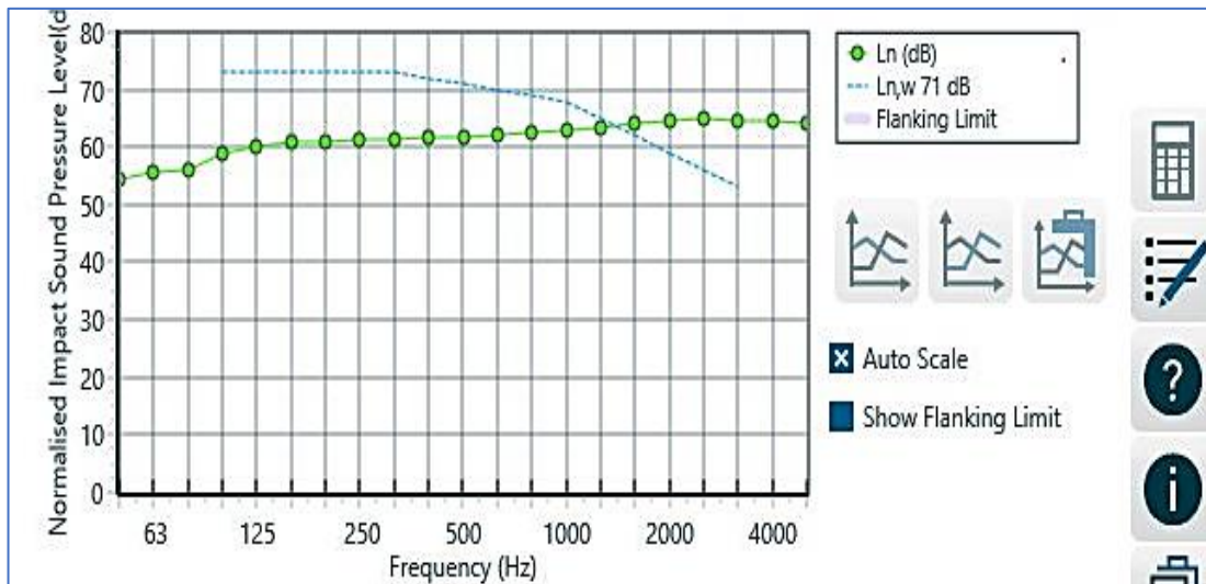
Figure 150 : Performance acoustique d'un plancher en béton de 20cm. Source : INSUL, 2022
