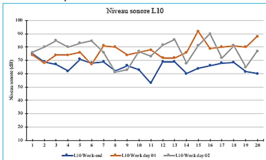
Figure 96 : Fluctuations de niveau sonore statistique L10 en mois de Février sur les 20 stations. Source : Auteur, 2022
