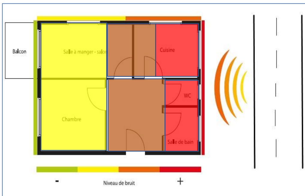
Figure 119 : Exemple explicatif de l'agencement souhaitable des pièces face au bruit routier. Source : Auteur, 2022
