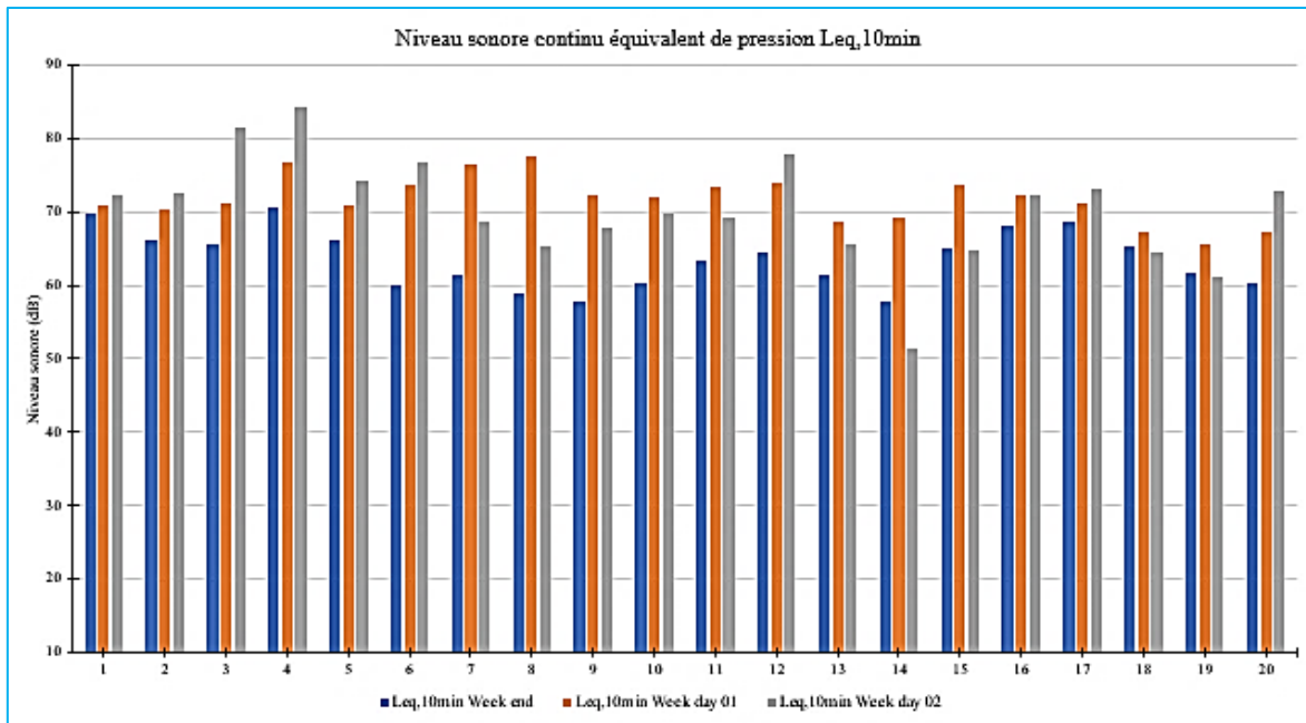
Figure 98 : Fluctuations de niveau sonore Leq,10min sur les 20 stations en mois de Mars. Source : Auteur, 2022
