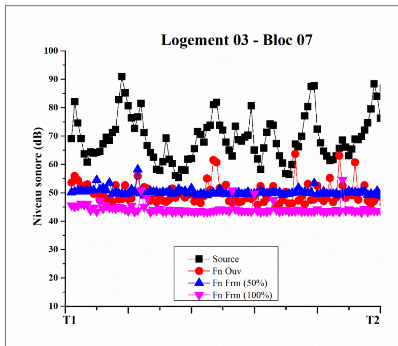
Figure 118 : Spectres sonores des niveaux de pression acoustique (Lp) du logement 03. Source : Auteur, 2022
