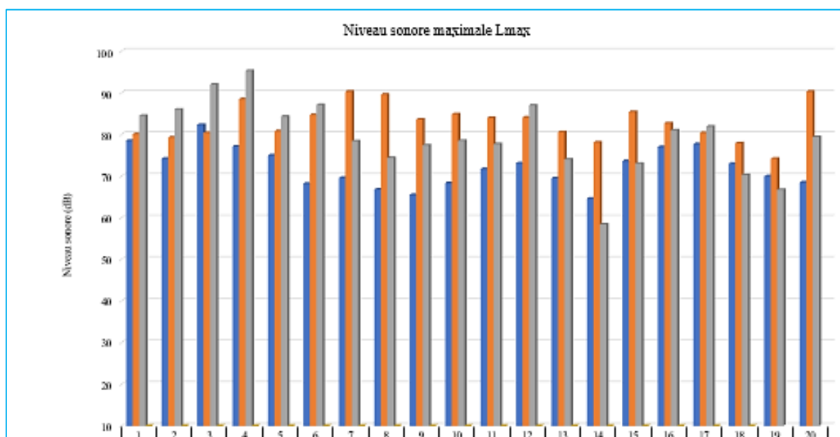
Figure 101 : Fluctuations de niveau sonore maximale Lmax sur les 20 stations en mois de Mars. Source : Auteur, 2022
