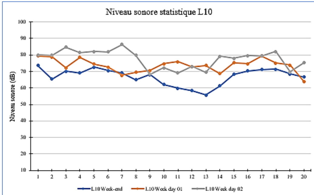
Figure 104 : Fluctuations de niveau sonore statistique L10 sur les 20 stations en mois de Juin. Source : Auteur, 2022
