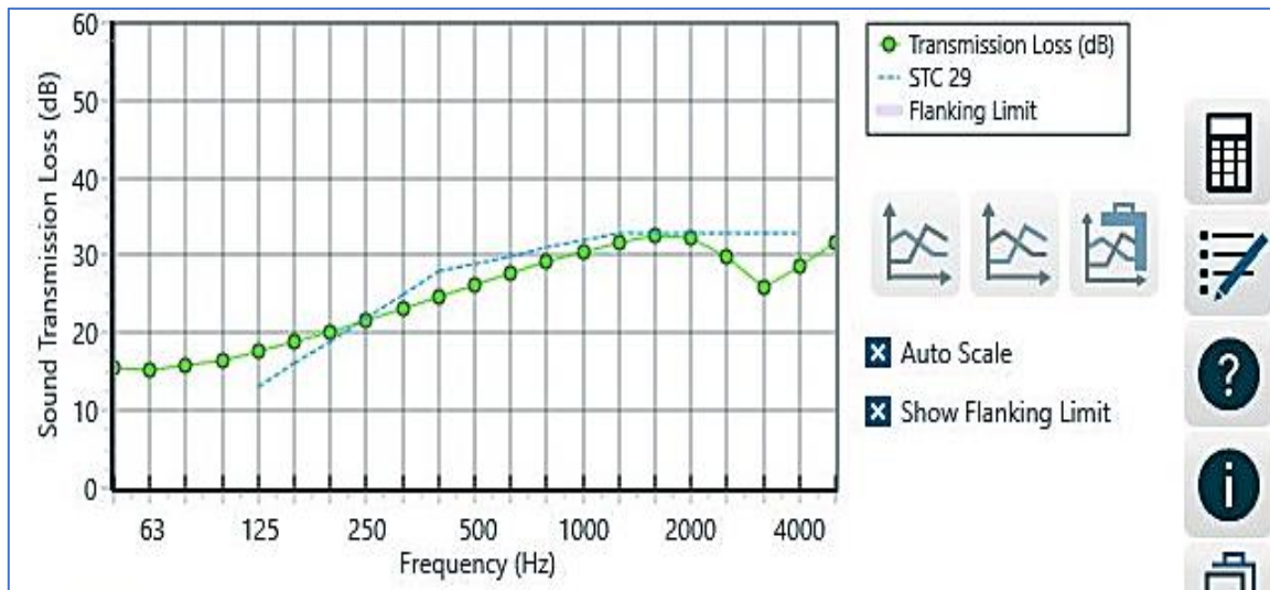
Figure 139 : Performance acoustique d'un simple vitrage de 4mm. Source : INSUL, 2022
