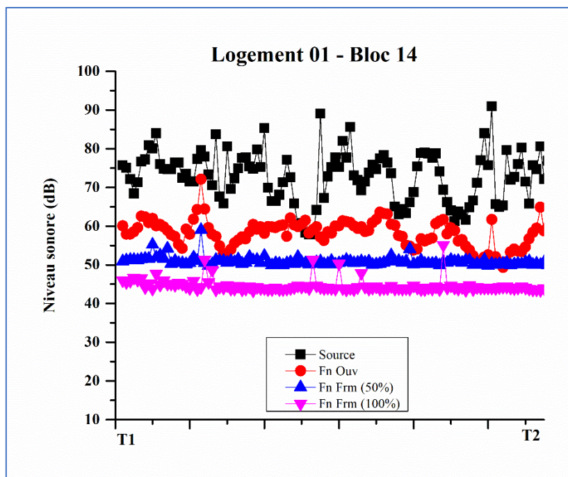
Figure 125 : Spectres sonores des niveaux de pression ( L_p ) du logement 01 avant rénovation. Source : Auteur, 2022
