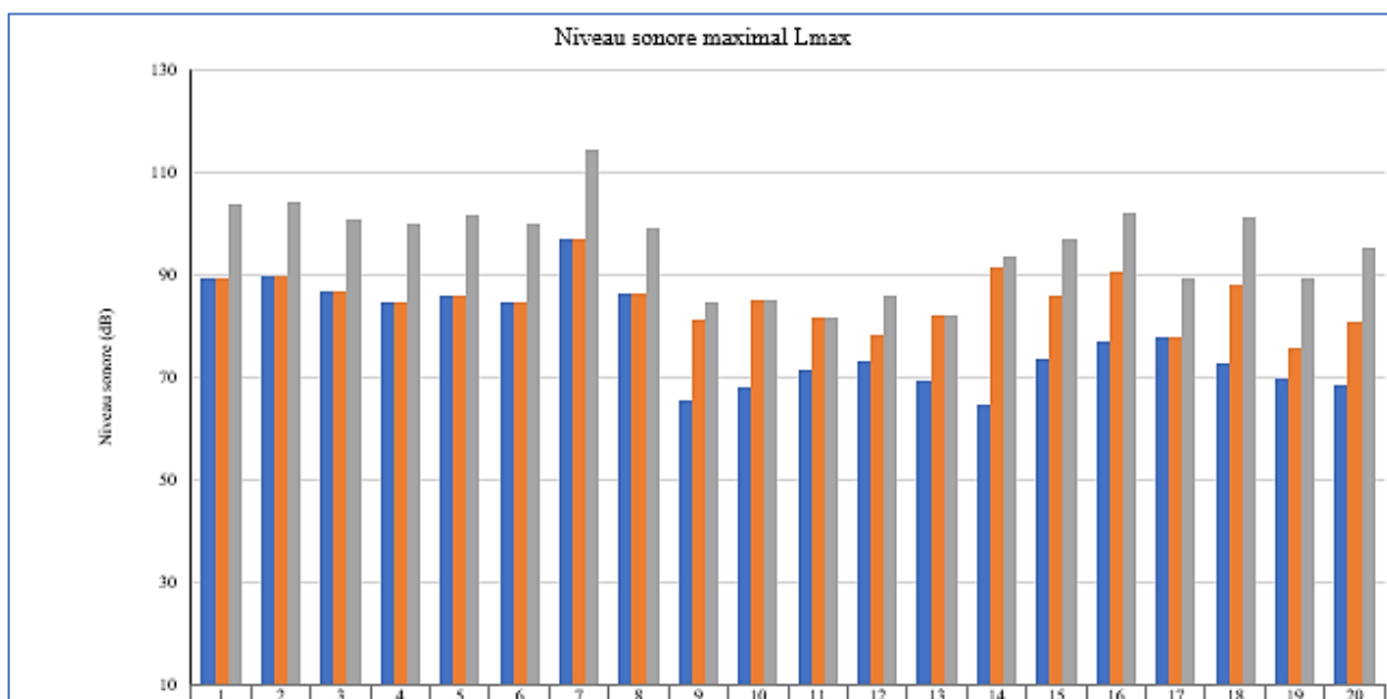
Figure 109 : Fluctuations de niveau sonore maximale L_{max} sur les 20 stations en mois de Juillet. Source : Auteur, 2022
