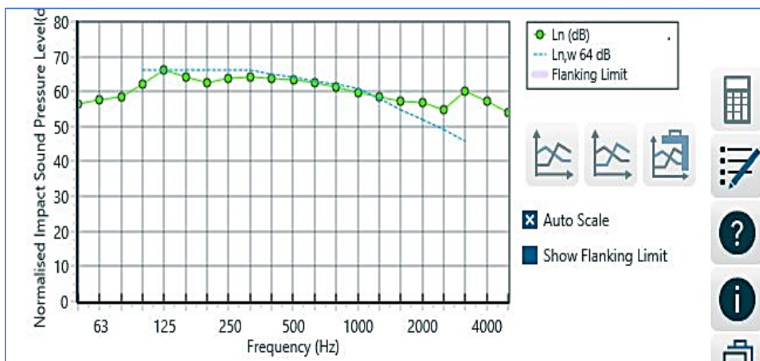
Figure 154 : Performance acoustique du plancher en béton de 20cm, lame d'air de 5cm et un panneau de plaque de plâtre de 1cm suspendu. Source : INSUL, 2022
