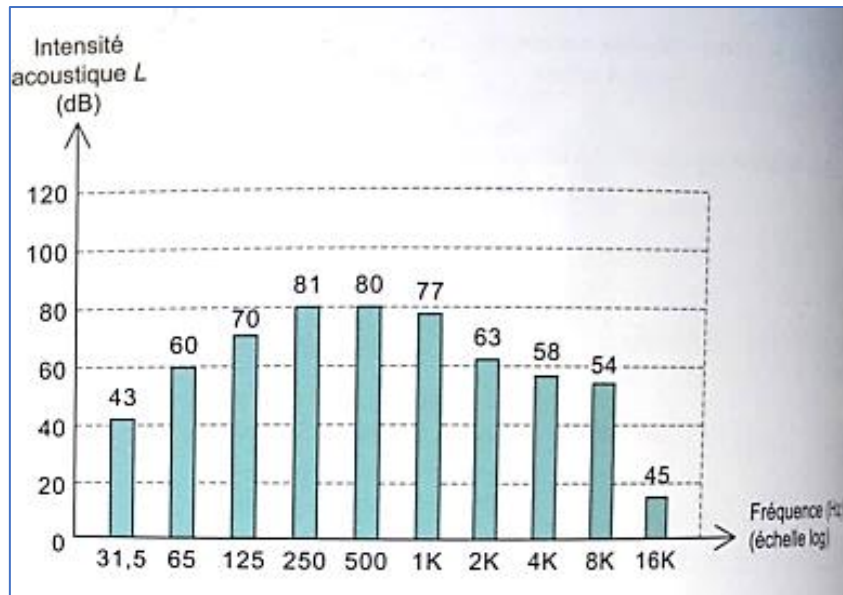
Figure 15 : Exemples de spectre en bandes d'octave. Source : Simonine, 2004
