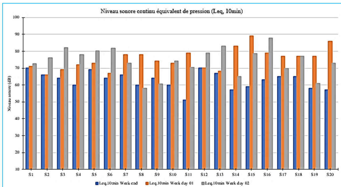
Figure 94 : Fluctuations de niveau sonore Leq,10min sur les 20 stations de mesure en mois de Février. Source : Auteur, 2022
