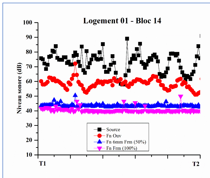
Figure 129 : Spectres sonores des niveaux de pression acoustique ( L_p ) du logement 01 après rénovation, par rapport au vitrage de 6mm. Source : Auteur, 2022
