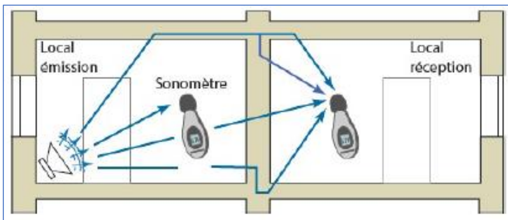
Figure 29 : Mesurage de l'isolement brut. Source : Rapin, 2017
