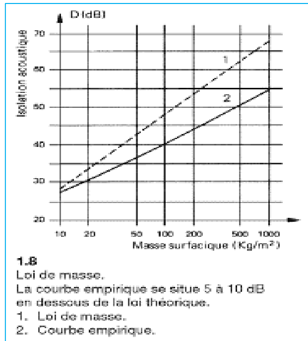
Figure 25 : Graphique sur la loi de masse. Source : Vitonne, 2010
