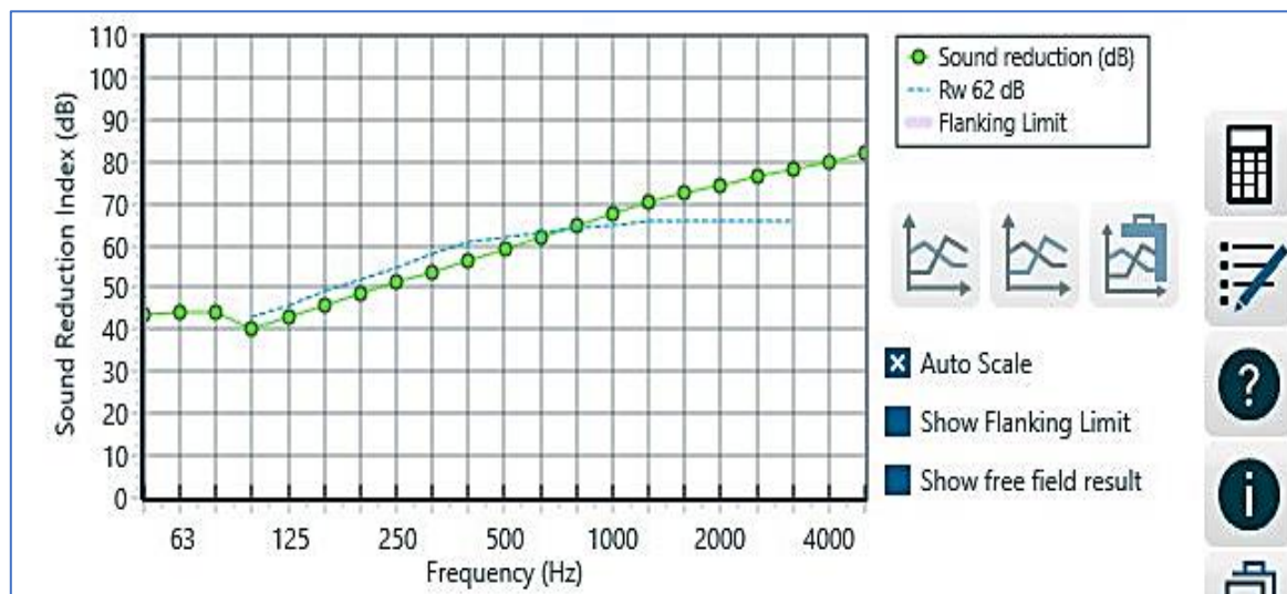
Figure 144 : Performance acoustique d'un mur en béton de 200mm. Source : INSUL, 2022
