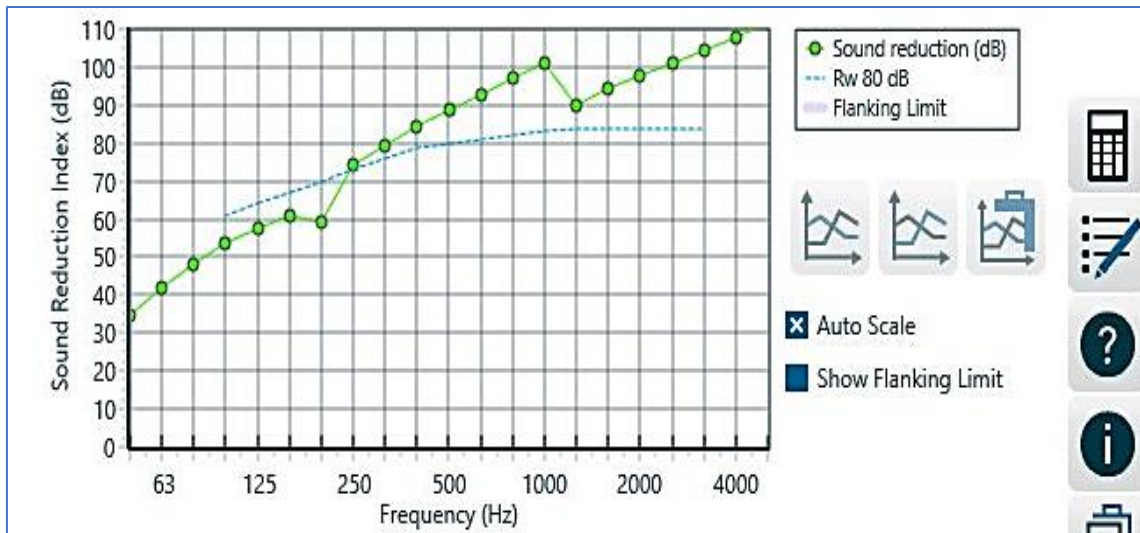
Figure 147 : Performance acoustique de mur en brique et laine de verre semi rigide de 5cm (INSUL, 2022)
