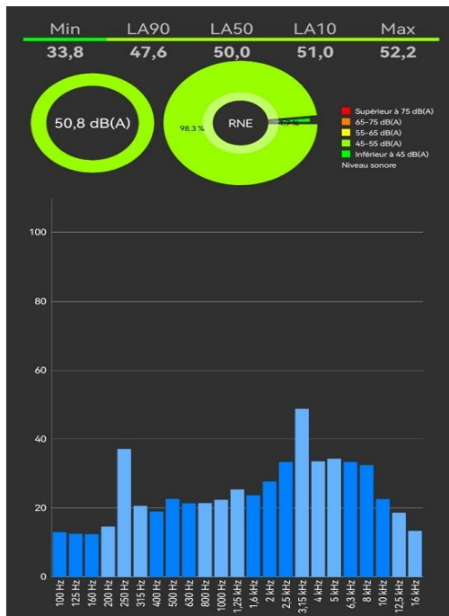
Figure 130 : Spectres sonores du bruit perçu à l'intérieur du logement 01 à l'aide de l'application NoiseCapture avec vitrage 2mm fermé. Source : Auteur, 2022
