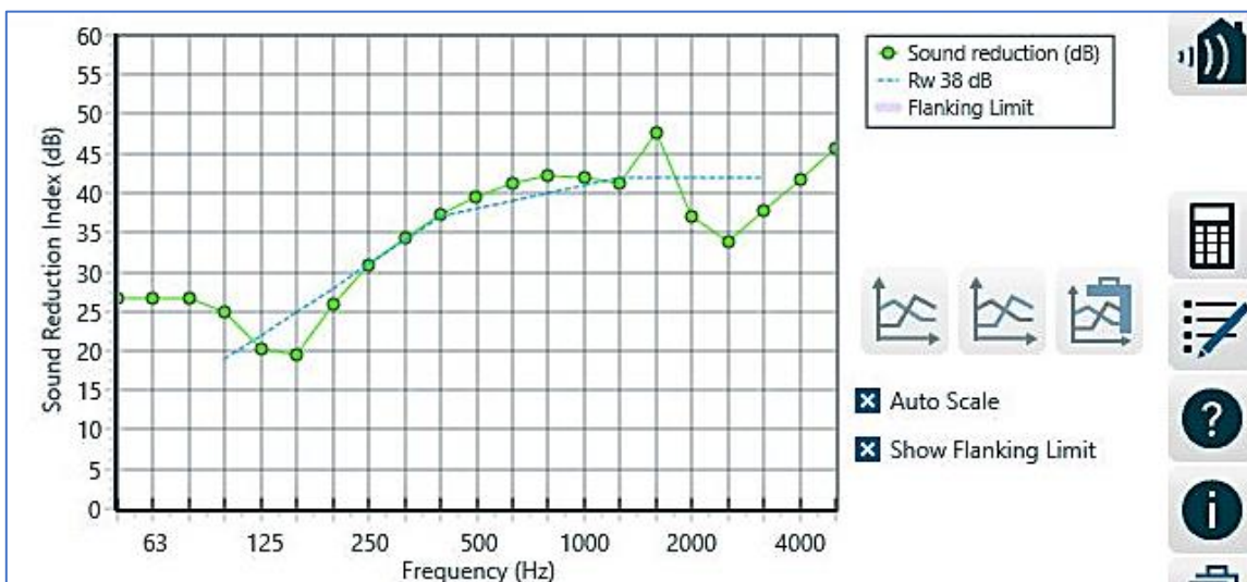
Figure 143 : Performance acoustique du double vitrage asymétrique de 6-20-10mm. Source : INSUL, 2022
