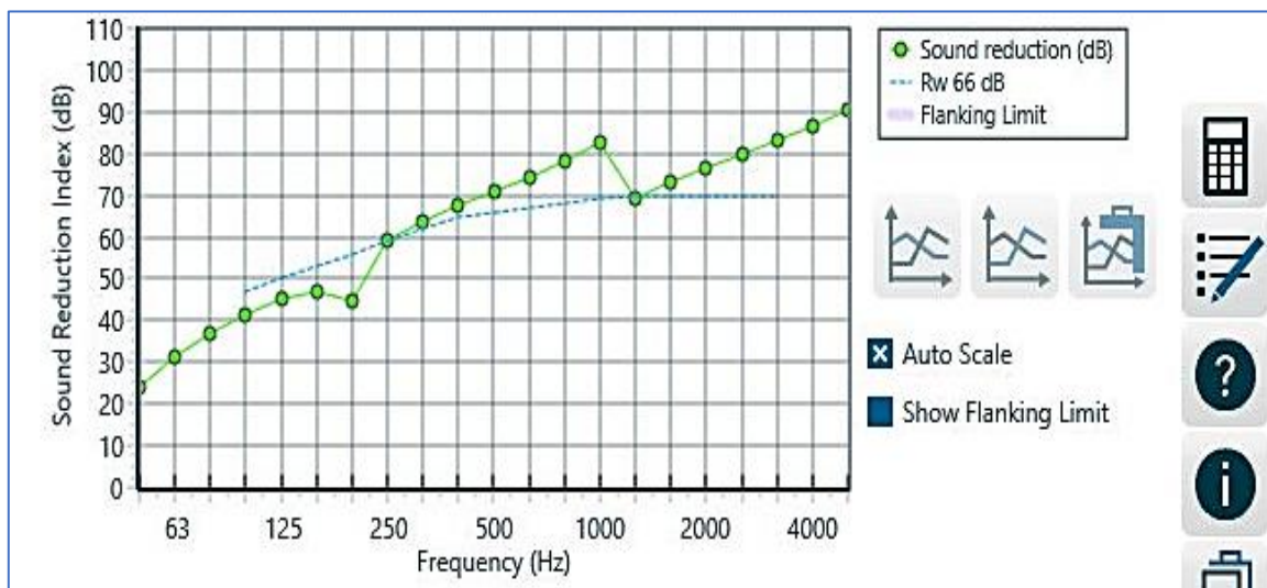
Figure 146 : Performance acoustique du mur en brique et plaque de liège de 15cm (INSUL, 2022)
