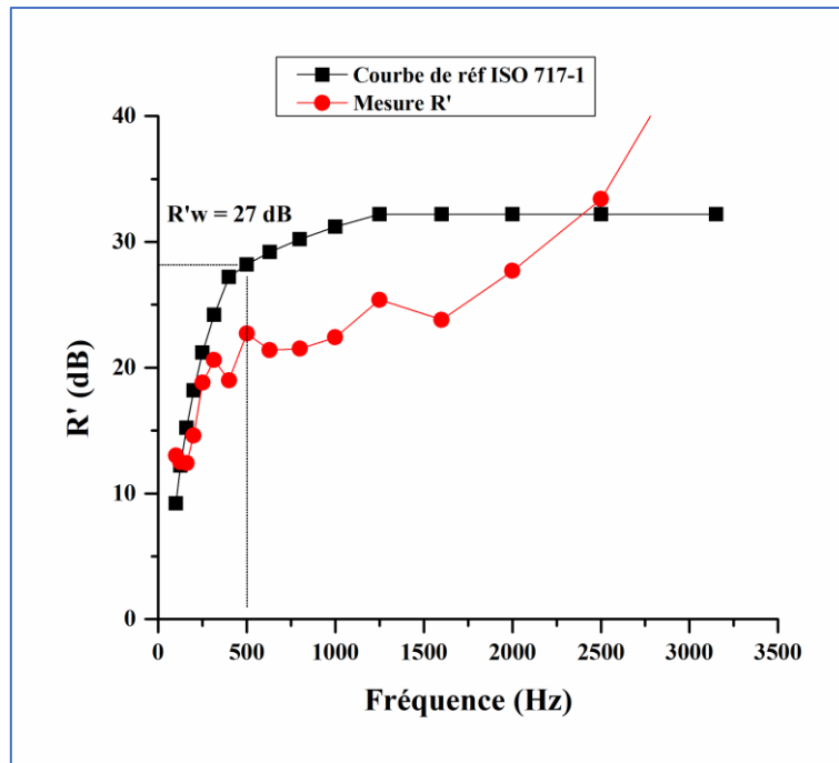
Figure 135 : Résultat de l'indice d'affaiblissement acoustique apparent pondéré R'_w du vitrage de 2mm. Source : Auteur, 2022
