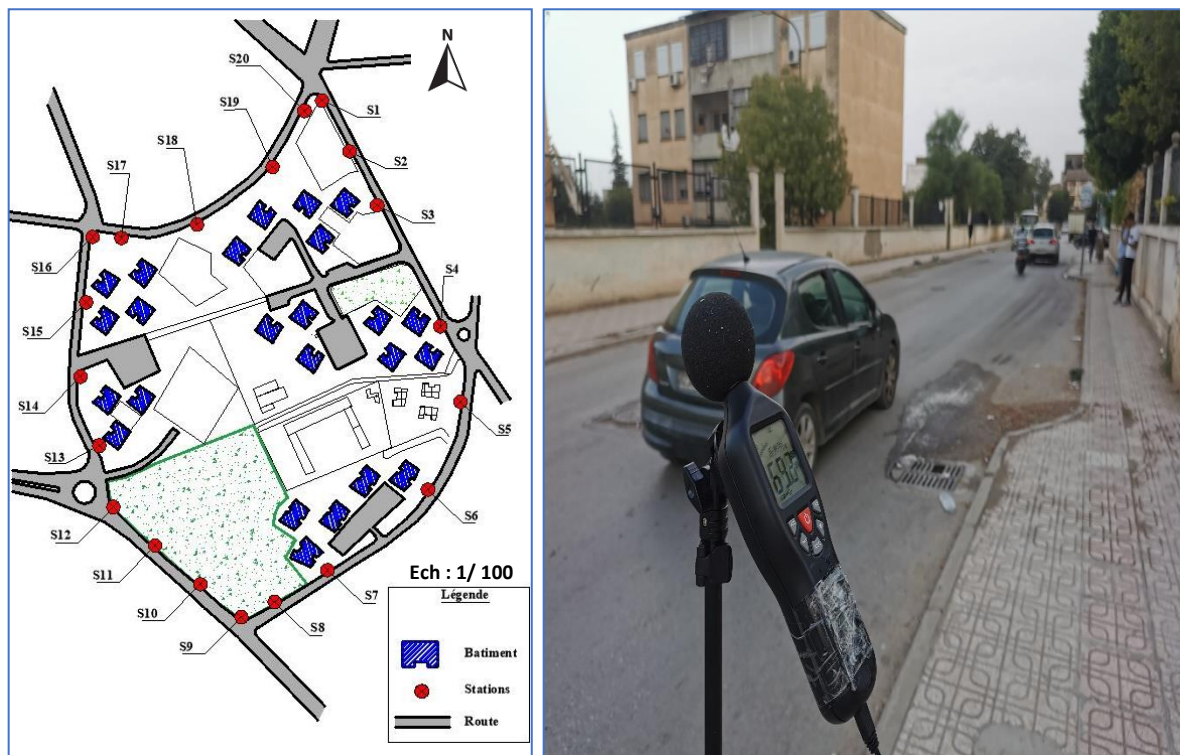
Figure 67 : Distribution spatiale des 20 stations de mesure de bruit routier. Source : Auteur, 2022
