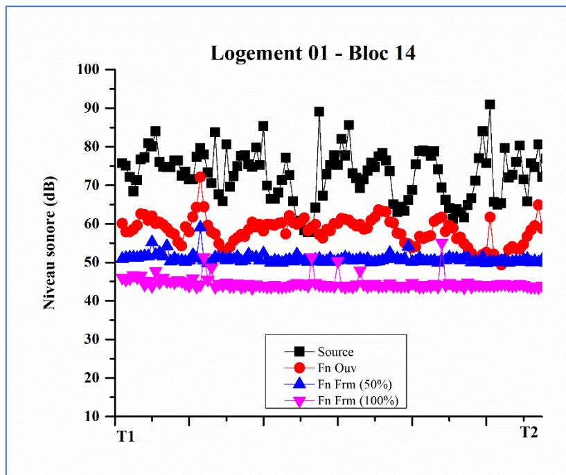
Figure 116 : Spectres sonores des niveaux de pression acoustique ( L_p ) du logement 01. Source : Auteur, 2022
