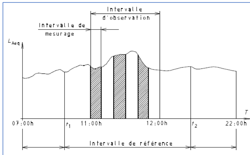
Figure 68 : Schéma explicatif des intervalles de mesurage, d'observation et de référence. Source : AFNOR, 1996
