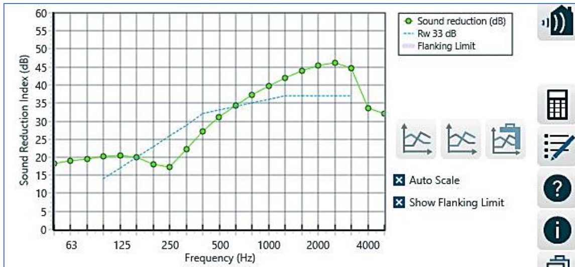
Figure 142 : Performance acoustique d'un double vitrage symétrique 3-20-3mm. Source : INSUL, 2022
