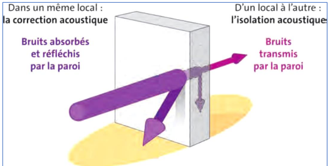
Figure 23 : Différence entre l'isolation et la correction acoustique. Source : Saint Gobain, 2012
