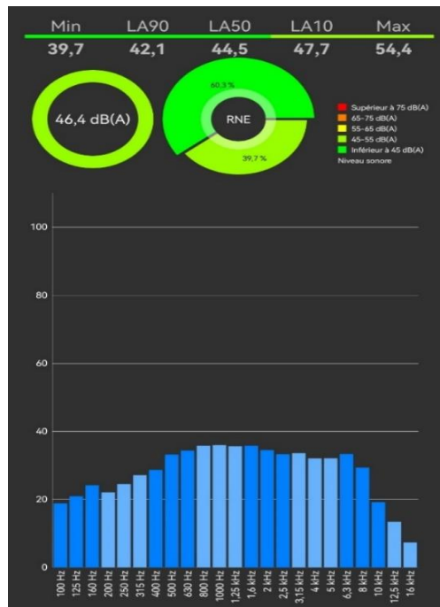
Figure 131 : Spectres sonores du bruit perçu à l'intérieur du logement 01 à l'aide de l'application NoiseCapture avec vitrage 2mm et persienne fermée. Source : Auteur, 2022
