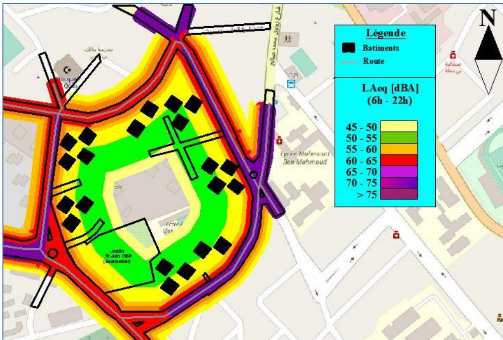
Figure 114 : Carte du bruit en courbes isophones pour la cité CDM en période estivale. Source : Auteur, 2022
