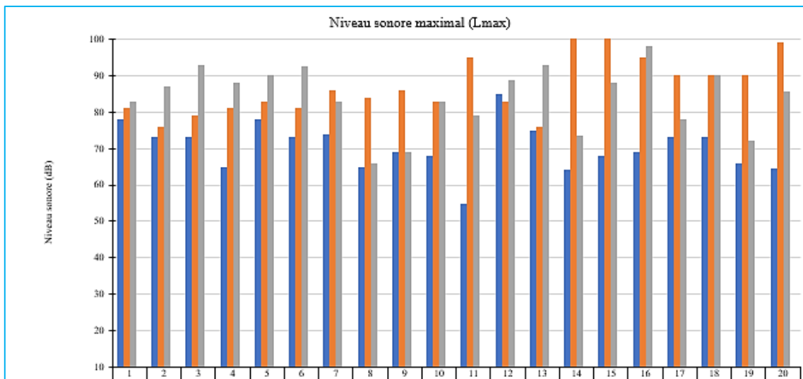
Figure 97 : Variation des niveaux sonores L_{max} sur les 20 stations en mois de Février. Source : Auteur, 2022
