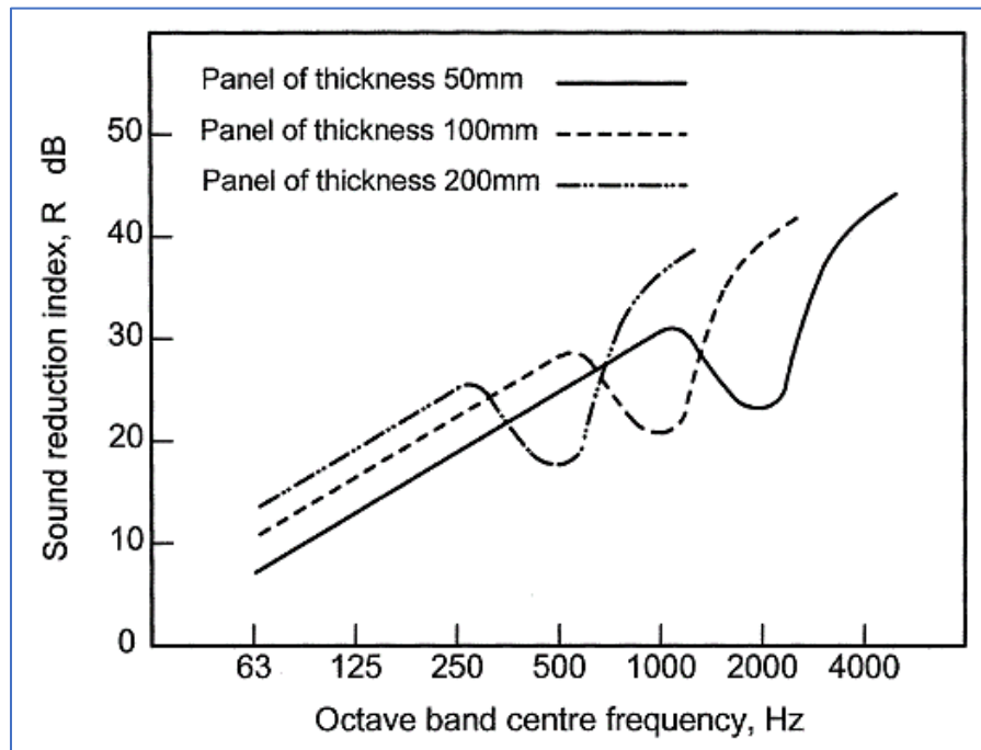
Figure 134 : Effet de l'augmentation de la masse surfacique sur l'indice d'affaiblissement acoustique. Source : Simons, 2008
