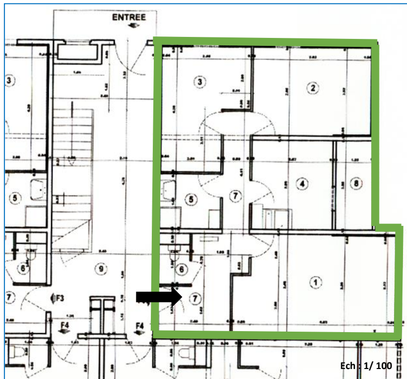
Figure 78 : Disposition spatiale en plan du logement 03 en bloc 07. Source : Auteur, 2022
