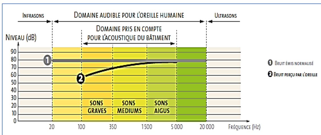
Figure 11 : Plages d'audibilité de l'oreille humaine. Source : Isover, 2007
