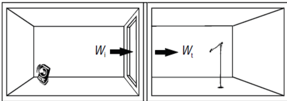
Figure 30 : Mesurage de l'indice d'affaiblissement acoustique en laboratoire. Source : Vigran, 2008
