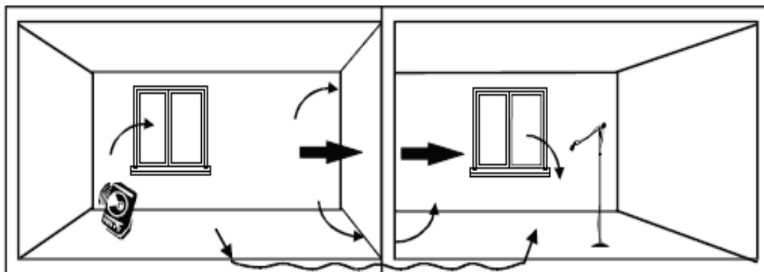
Figure 32 : Mesurage de l'indice d'affaiblissement acoustique apparent in-situ (Vigran, 2008)
