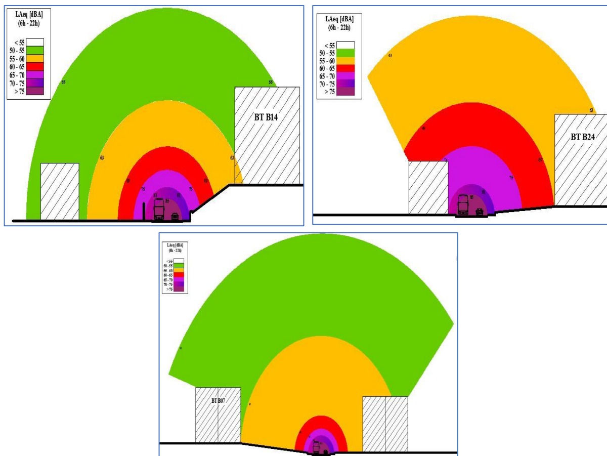
Figure 115 : Effet de l'éloignement de la source par des contours des niveaux sonores en segment I, II et IV, respectivement. Source : Auteur, 2022
