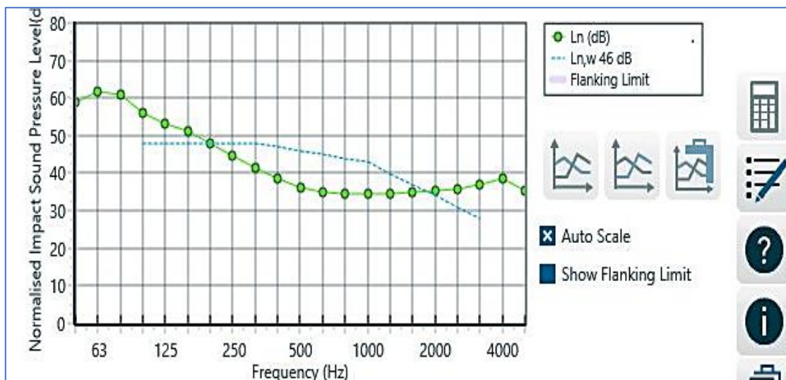
Figure 151 : Performance acoustique du plancher en béton de 20cm, laine de verre semi rigide de 10cm et panneau de plaque de plâtre de 10cm suspendu. Source : INSUL, 2022
