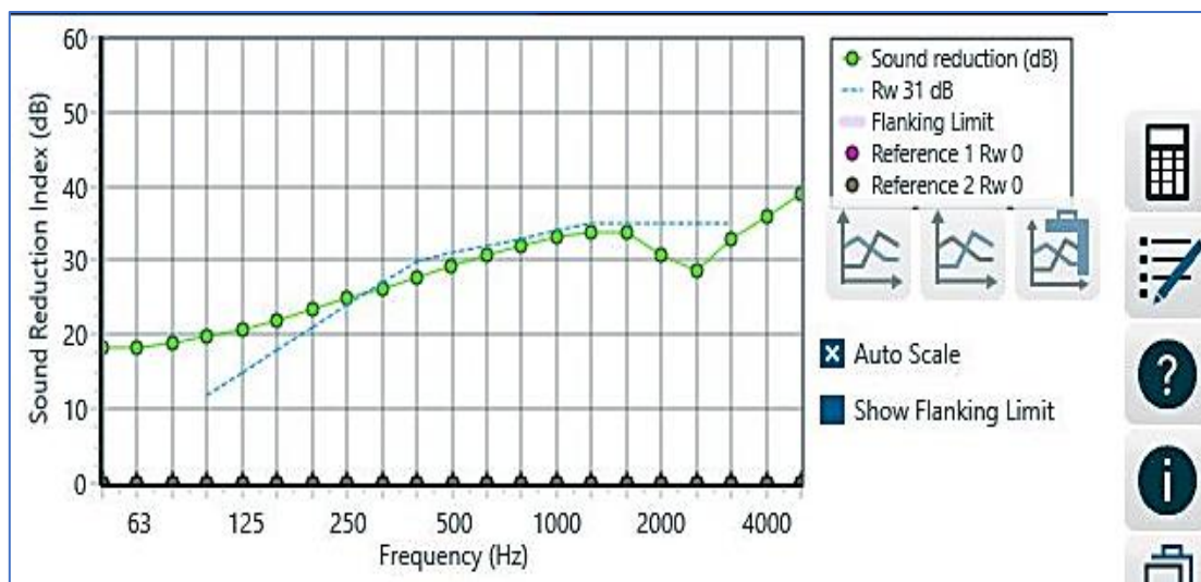
Figure 140 : Performance acoustique d'un simple vitrage de 6mm. Source : INSUL, 2022
