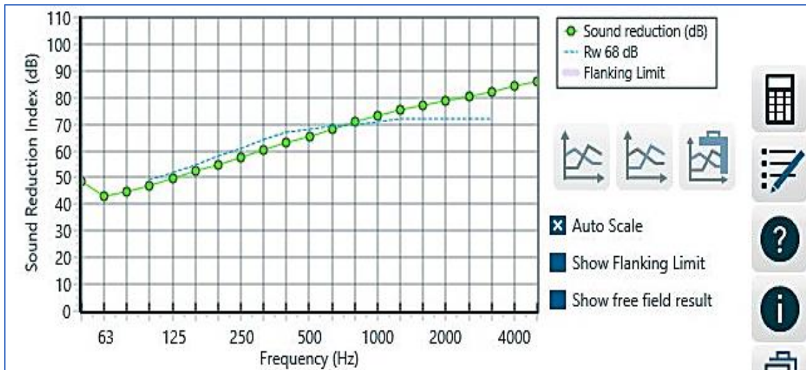
Figure 145 : Performance acoustique d'un mur en béton de 300mm. Source : INSUL, 2022
