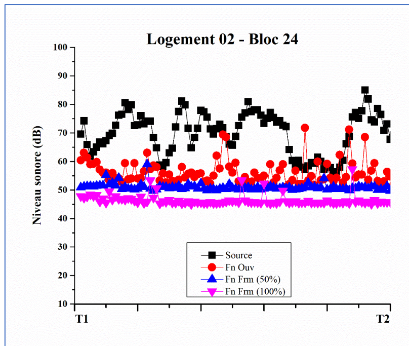
Figure 117 : Spectres sonores des niveaux de pression acoustique ( L_p ) du logement 02. Source : Auteur, 2022
