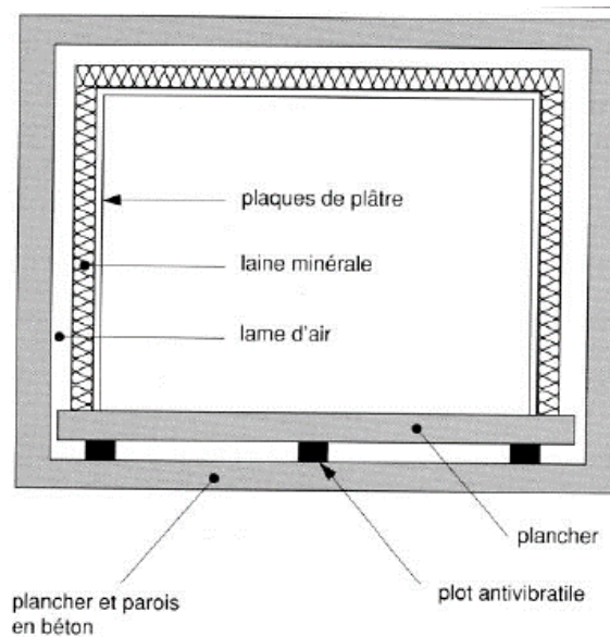
Figure 28 : Principe de la boîte dans la boîte. Source : Rapin, 2017
