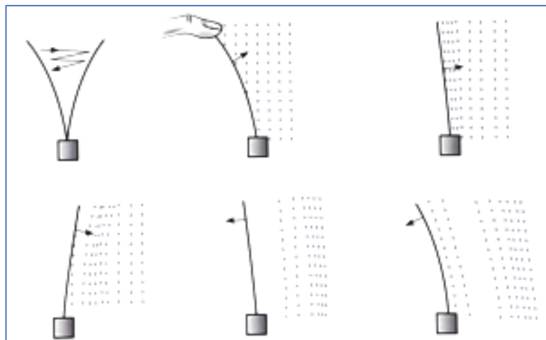
Figure 10 : Oscillations d'une lame d'acier. Source : Michel, 2001
