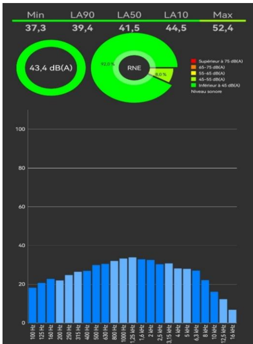
Figure 132 : Spectres sonores du bruit perçu à l'intérieur du logement 01 à l'aide de l'application NoiseCapture avec vitrage 6mm fermé. Source : Auteur, 2022
