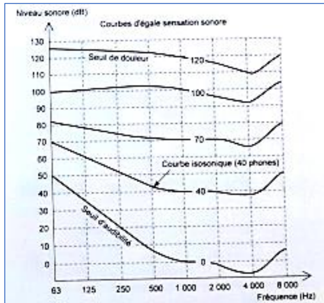
Figure 12 : Courbes d'égale sensation sonore. Source : Saint Gobain, 2012
