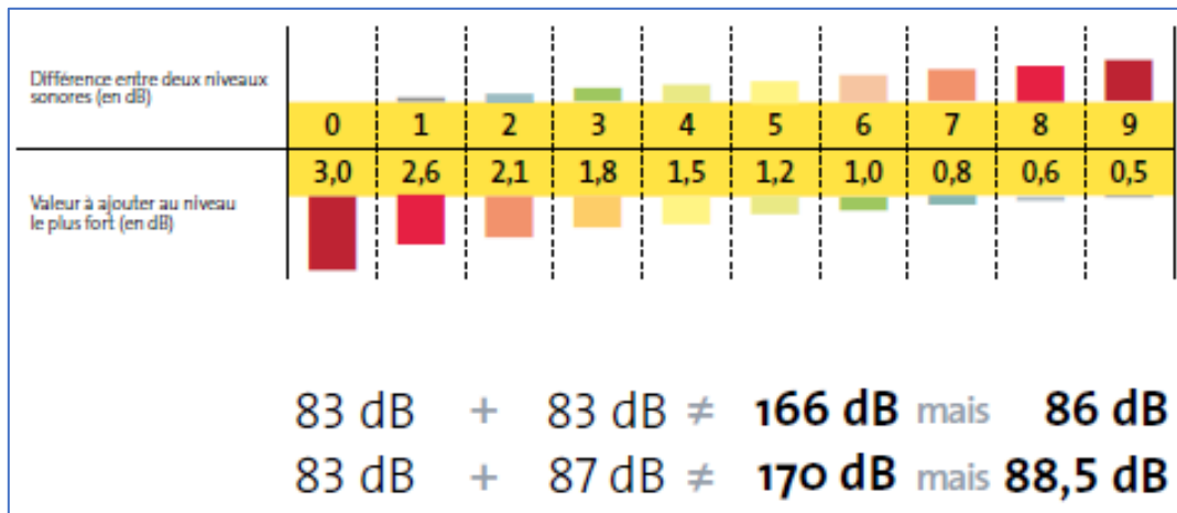
Figure 22 : Règles d'addition des niveaux sonores. Source : ISOVER, 2007
