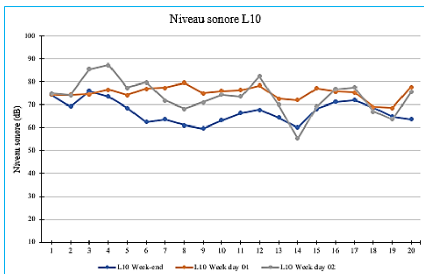
Figure 100 : Fluctuations de niveau sonore statistique L10 sur les 20 stations en mois de Mars. Source : Auteur, 2022
