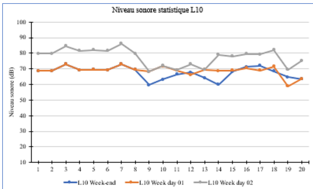
Figure 108 : Fluctuation de niveau sonore statistique L10 sur les 20 stations en mois de Juillet. Source : Auteur, 2022
