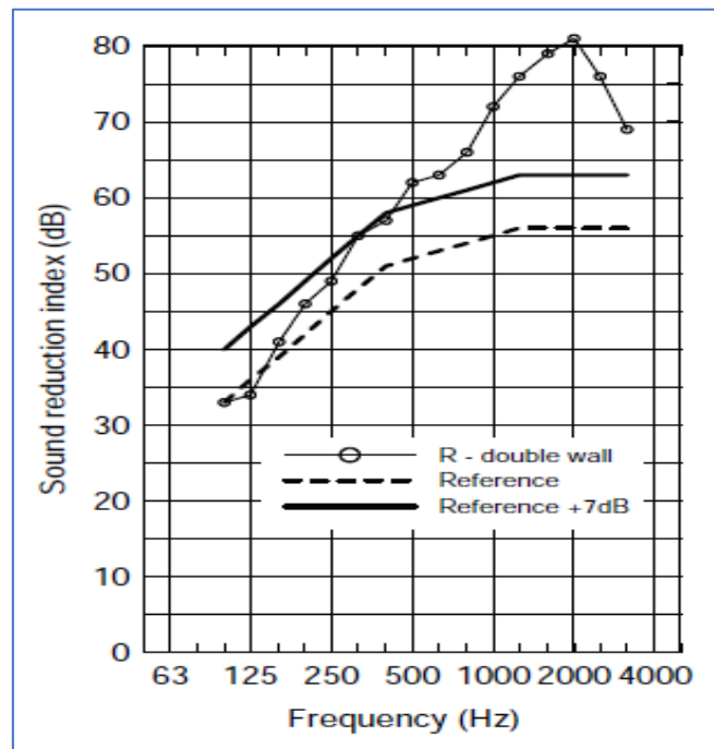
Figure 31 : Courbe de référence selon ISO717-1. Source : Vigran, 2008
