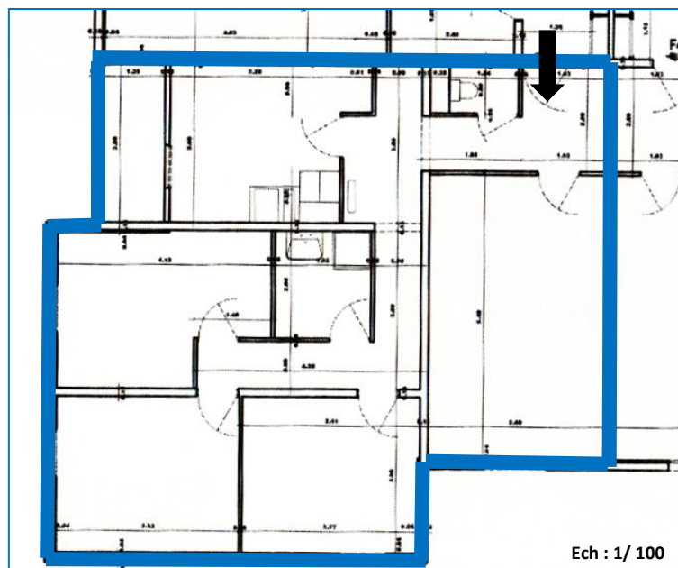
Figure 75 : Disposition spatiale en plan du logement 2 en bloc 24. Source : Auteur, 2022
