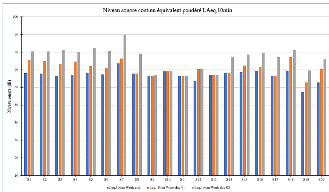
Figure 106 : Fluctuations de niveau sonore LA_{eq,10min} sur les 20 stations en mois de Juillet. Source : Auteur, 2022
