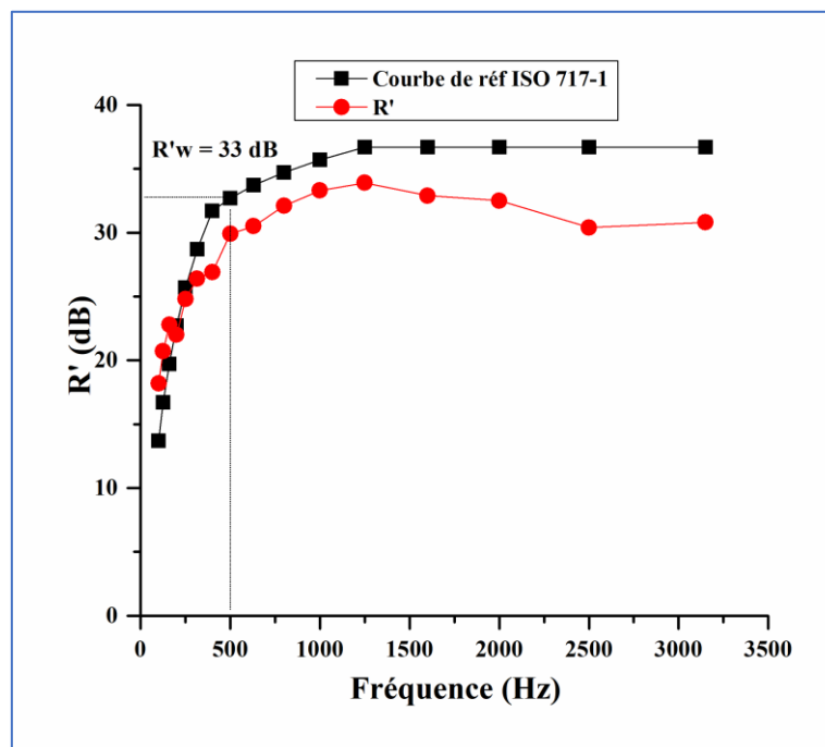
Figure 136 : Résultat de l'indice d'affaiblissement acoustique apparent pondéré R'_w du vitrage de 6mm. Source : Auteur, 2022
