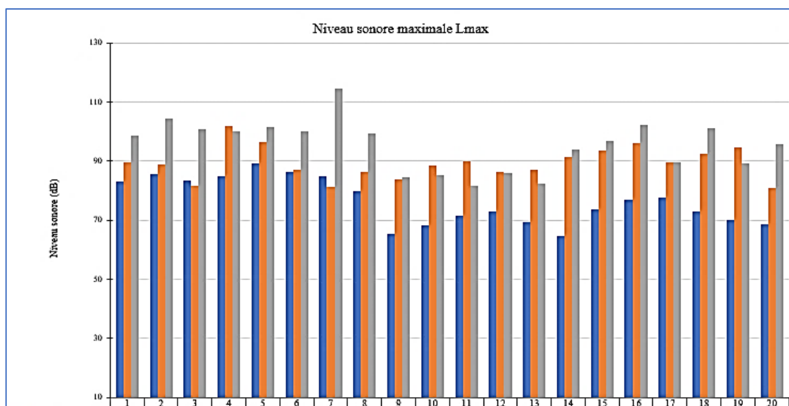
Figure 105 : Fluctuations de niveau sonore maximale Lmax sur les 20 stations en mois de Juin (Auteur, 2022)
