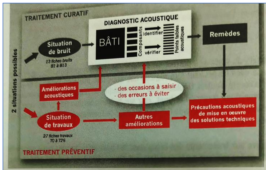
Figure 24 : Schéma de traitement acoustique dans l'habitat existant. Source : Simonine, 2004
