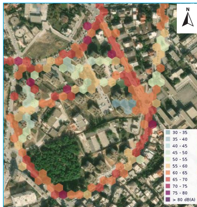
Figure 91 : Image satellitaire de la cartographie sonore de la cité Champs de Manoeuvre via Noise Capture0 Source : https://noise-planet.org/map_noisecapture/index.html#17/36.45839/7.43003/ , 2022
