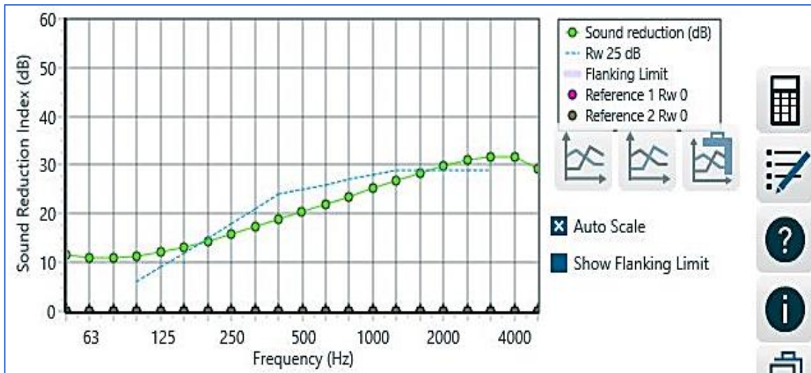
Figure 138 : Performance acoustique d'un simple vitrage de 2mm. Source : INSUL, 2022
