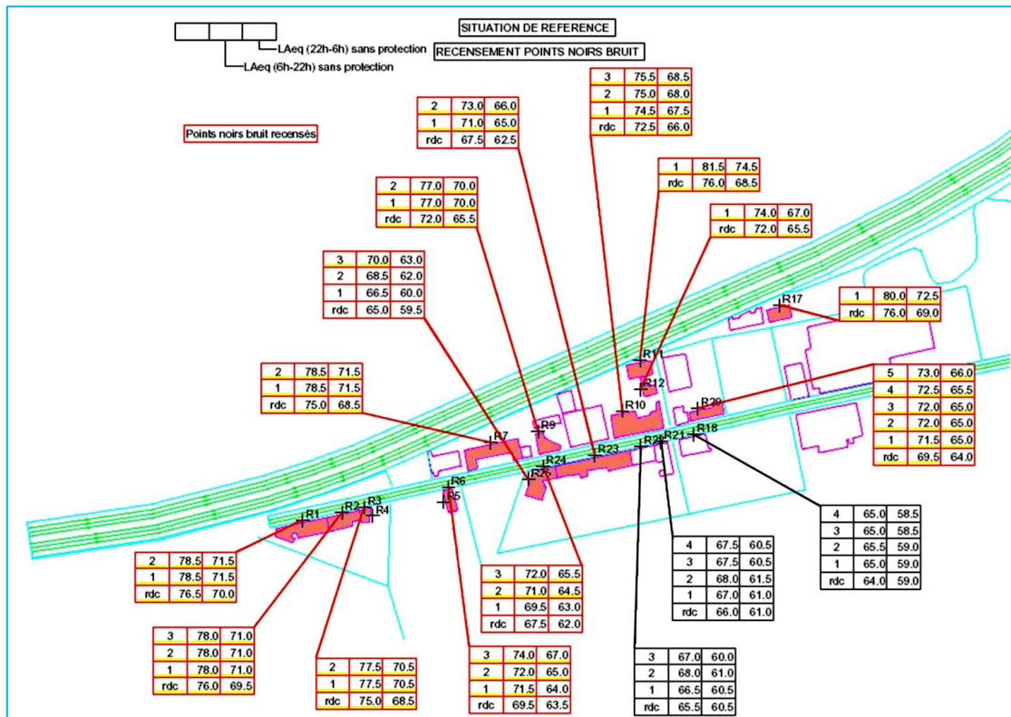
Figure 110 : Exemple d'une carte stratégique de bruit en étiquettes chiffrées. Source : Certu, 2003
