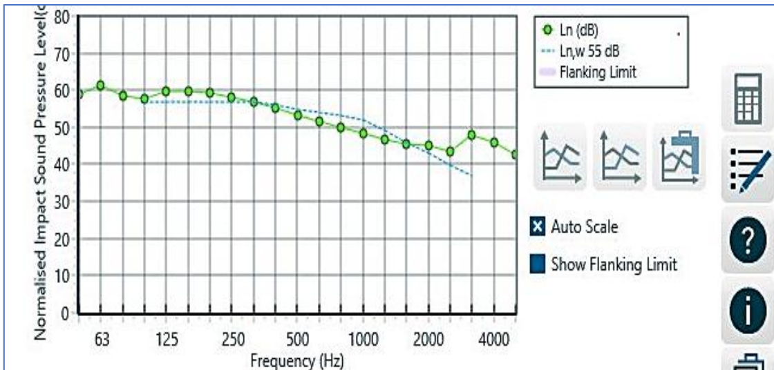
Figure 152 : Performance acoustique du plancher en béton de 20cm, lame d'air de 20cm et un panneau de plaque de plâtre de 1cm suspendu. Source : INSUL, 2022
