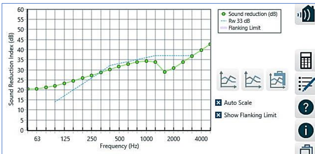
Figure 141 : Performance acoustique d'un simple vitrage de 8mm. Source : INSUL, 2022
