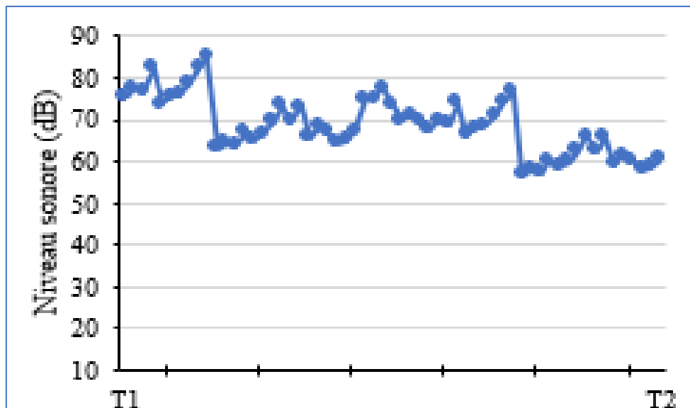
Figure 92 : Fluctuations des valeurs de LA_{eq,1min} durant le mesurage acoustique préliminaire. Source : Auteur, 2022
