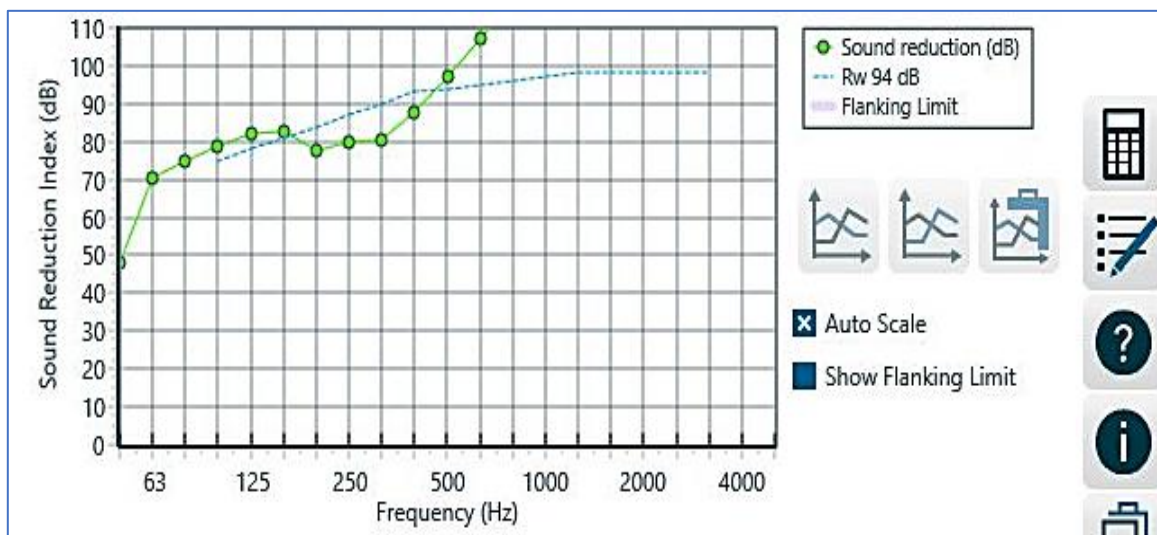
Figure 148 : Performance acoustique de mur en brique, avec la laine de verre de 10cm et un panneau de 10cm de béton. Source : INSUL, 2022
