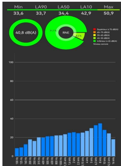
Figure 133 : Spectres sonores du bruit perçu à l'intérieur du logement 01 à l'aide de l'application NoiseCapture avec vitrage 6mm et persienne fermée. Source : Auteur, 2022
