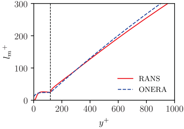
(a) Longueur de mélange l_m^+ pour la configuration H1
