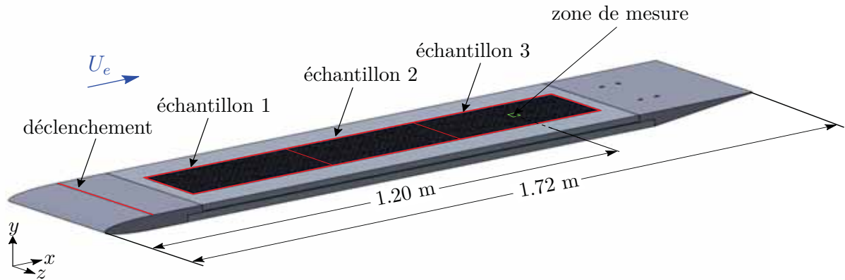
FIGURE 4.1. – Vue schématique de la maquette d'étude
