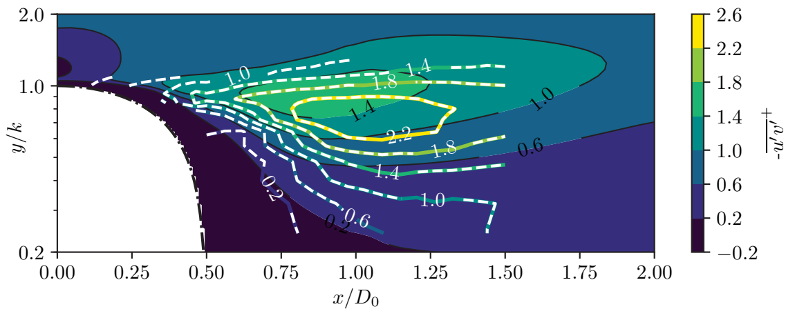
(c) Contours des contraintes de Reynolds -\bar{u}'v'^+ dans le plan (xy) à z/D_0 = 0 pour le cas H0.
