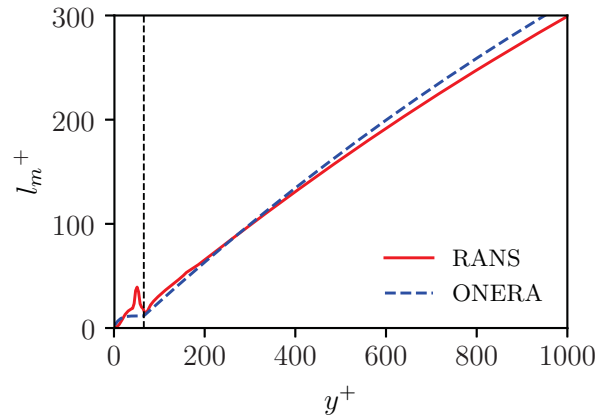
(d) Longueur de mélange l_m^+ la configuration C2
