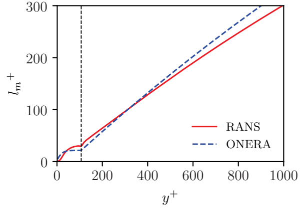
(b) Longueur de mélange l_m^+ pour la configuration H2
