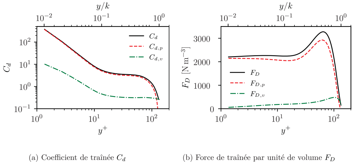
FIGURE 6.1. – Tracé des profils (a) du coefficient de traînée C_d et (b) de la force de traînée par unité de volume F_D le long d'un hémisphère de la configuration H0. La ligne - - - représente la contribution de la pression tandis que la ligne - · - · celle de la viscosité.
