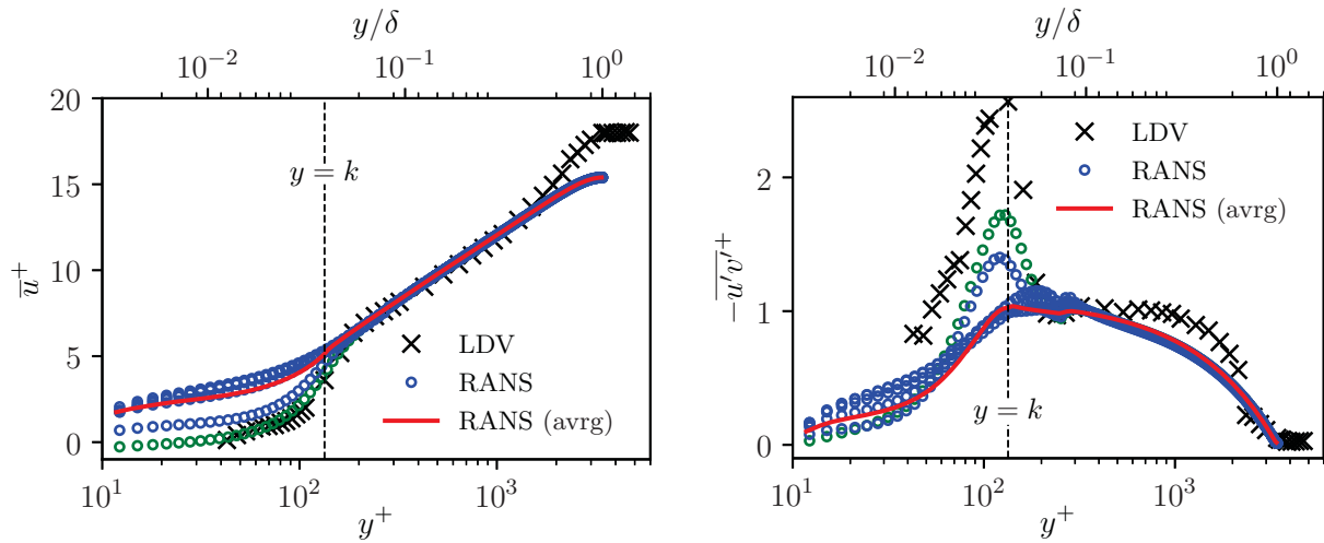
(a) Profil de vitesse longitudinale moyenne \bar{u}^+ (b) Profil des tensions de Reynolds -\overline{u'v'}^+
