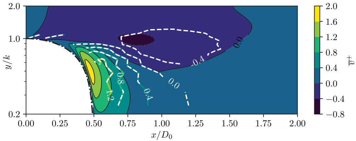
(b) Contours de la vitesse normale \bar{v}^+ dans le plan (xy) à z/D_0 = 0 pour le cas H0.
