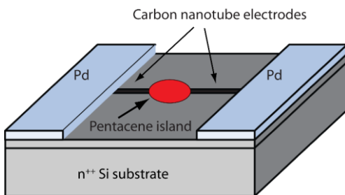
Figure VI-3 : Représentation schématique du nanotransistor à pentacène. Un îlot de pentacène est contacté par deux électrodes (source et drain) en nanotubes de carbone. Les deux électrodes sont formées à partir d'un nanotube de carbone métallique ouvert en son milieu par claquage électrique.
