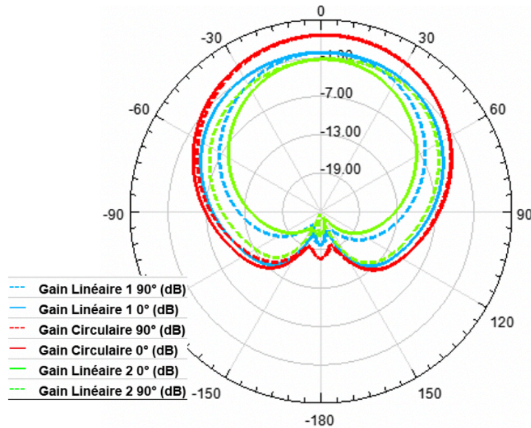
Figure 150. Résultat du diagramme de rayonnement simulés dans les différentes configurations [62].
