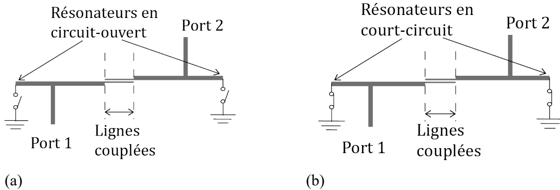
Figure 101. Dessin du filtre interdigités accordable. (a) A l'état OFF. (b) A l'état ON.
