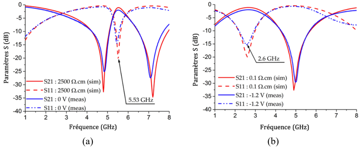
Figure 112. Comparaison entre les résultats simulés et mesurés du filtre accordable \text{DBR}_2 . (a) A l'état OFF. (b) A l'état ON [53].
