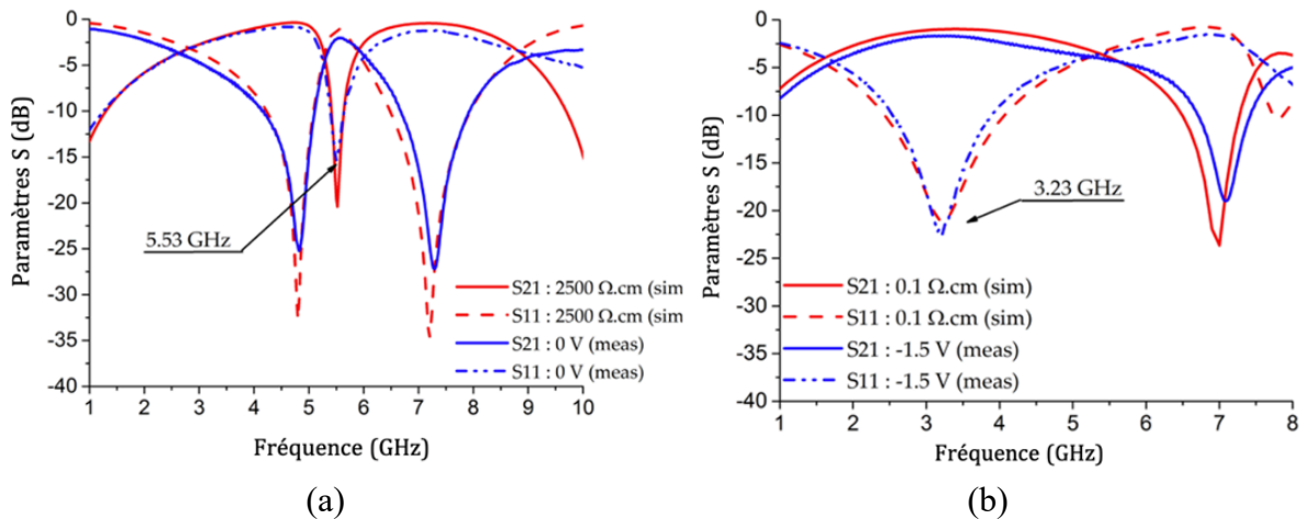
Figure 113. Comparaison entre les résultats simulés et mesurés du filtre accordable \text{DBR}_3 . (a) A l'état OFF. (b) A l'état ON [53].
