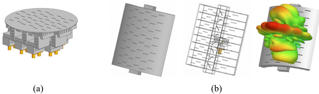
Figure 54. (a) Antenne réseaux 24 voies. (b) Antenne réseaux conformée et son diagramme de rayonnement [30].
