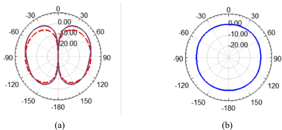
Figure 21. Diagramme de rayonnement. (a) Élévation (Phi=0deg en trait plein et Phi=90deg en pointillé). (b) Azimuth [17].
