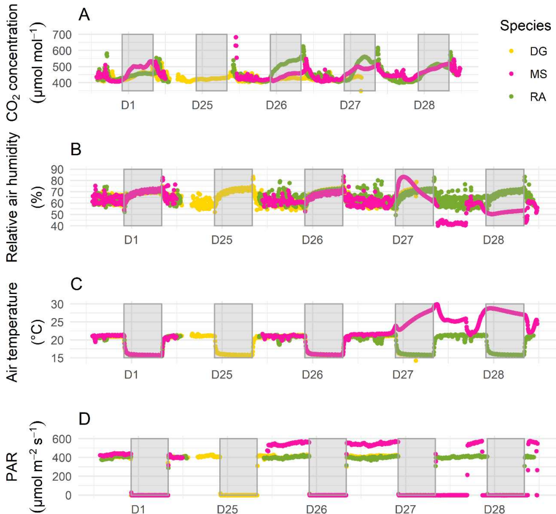
Figure 35. Évolution temporelle de la concentration en \text{CO}_2 (A), de l'humidité relative de l'air (B), de la température de l'air (C) et du rayonnement photosynthétiquement actif (D) dans la chambre climatique durant les expérimentations sur D. glomerata en jaune, M. sativa en rose et R. acetosa en vert. L'alternance des rectangles blancs et gris représente le cycle jour/nuit dont la photopériode est de 14 heures.
