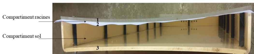
Figure 28. Visualisation de l'organisation du rhizotron. 1. Plaque transparente, 2. Toile, 3. Contenant. Le compartiment « racines » est situé entre la plaque transparente et la toile (entre 1 et 2) et le compartiment « sol » dans l'espace restant (entre 2 et 3).
