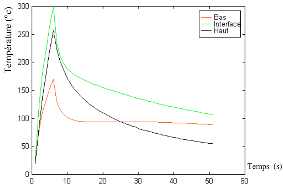
Figure V-32 : Evolution des températures dans les conditions de soudure
