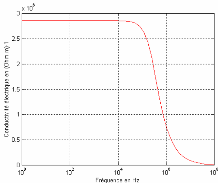
Figure IV-23 : Evolution de la conductivité équivalente en fonction de la fréquence.
