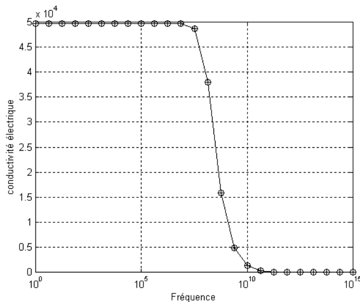
Figure V-6 : Evolution de la conductivité électrique \sigma_x et \sigma_y en fonction de la fréquence
