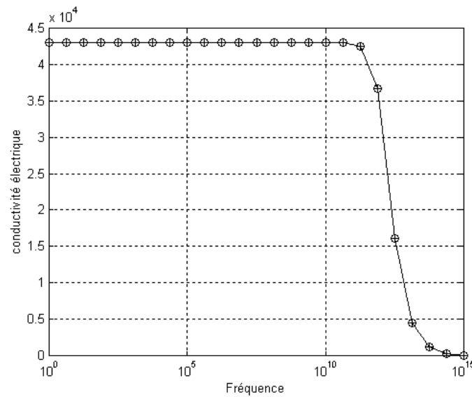
Figure V-11 : Variation de \sigma_z en fonction de la fréquence
