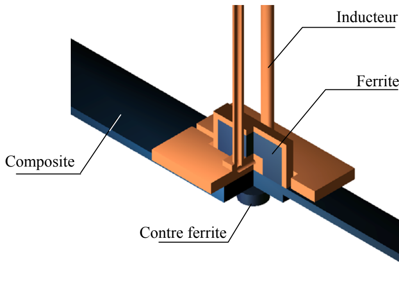
Figure V-23 : Tête de soudage par point 1
