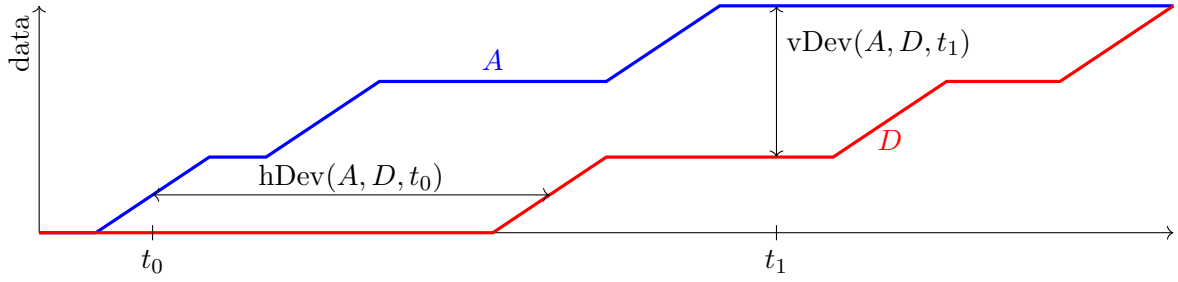
FIGURE 6.3 – Déviations horizontales à t_0 et verticales à t_1
