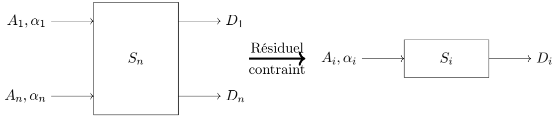
FIGURE 6.7 – Serveur résiduel contraint
