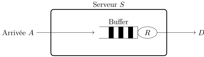
FIGURE 3.2 – Exemple d'un serveur S avec une arrivée A , un buffer, un débit R et un départ D . Les données entrantes arrivant en A sont stockés dans le Buffer avant d'être émise en D avec un débit R .
