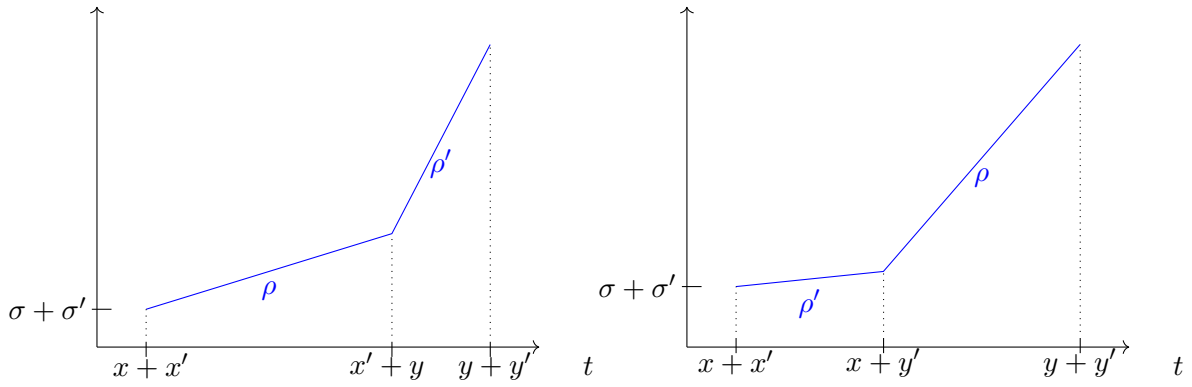
FIGURE 7.5 – Convolution de deux segments. Soit f et f' deux fonctions qui sont respectivement (\rho, \sigma) -affine sur [x; y[ et (\rho', \sigma') -affine sur [x'; y'[ et valent +\infty ailleurs. Nous avons tracé les deux cas de f * f' sur [x + x', y + y'[ : à gauche pour \rho < \rho' et à droite pour le cas \rho' < \rho .
