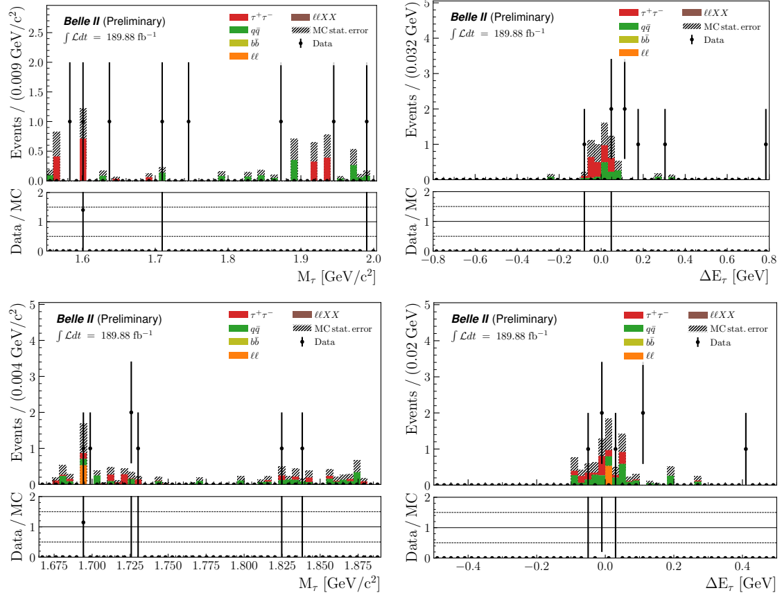
FIGURE 3 : Comparisons données-MC des distributions de M_\tau (gauche) et \Delta E_\tau (droite) dans les bandes latérales à 5 - 20\sigma , dans les canaux \tau \rightarrow e\phi (haut) et \tau \rightarrow \mu\phi (bas), après application de la présélection, du critère du BDT et de la coupure 2D.
