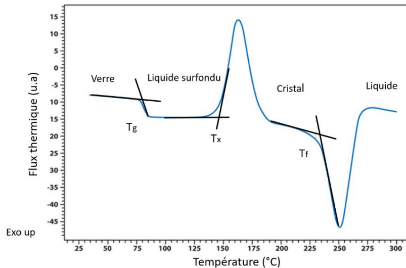
Figure I 1-4 : Thermogramme caractéristique d'un verre.
