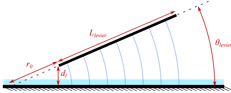
FIGURE B.4 : Illustration des paramètres géométriques importants pour le calcul de la force due au corps du levier. Les lignes en pointillés bleus représentent les lignes de champs.
