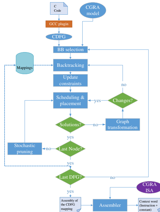
FIGURE 3.2 – Flot de projection d'une application spécifiée en langage C sur une architecture type CGRA
