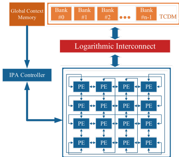
FIGURE 3.1 – IPA, Integrated Programmable Array , le CGRA que nous avons proposé
