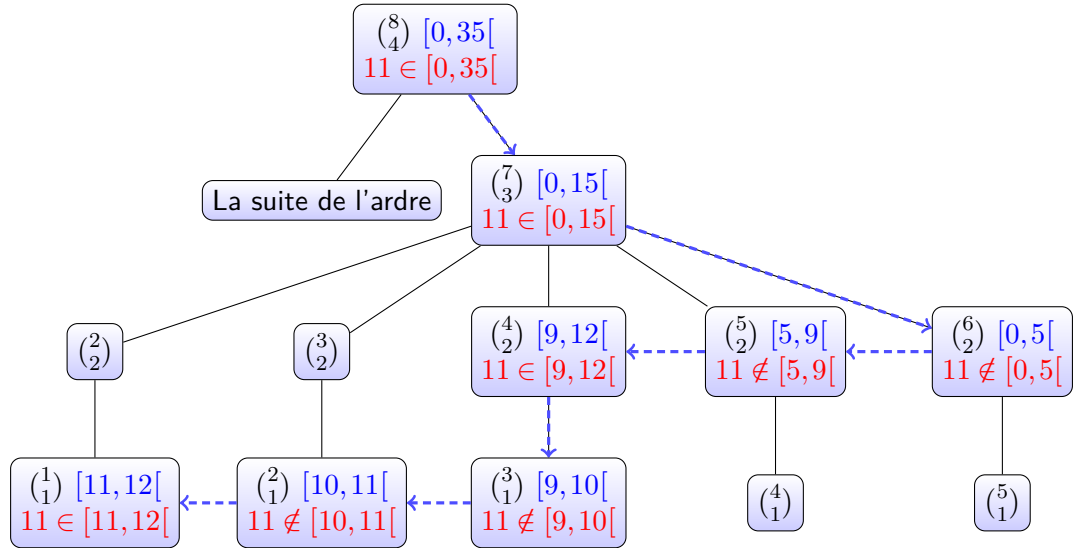
FIGURE IV.7 – Exemple du parcours pour déterminer les successeur d'un entier b
