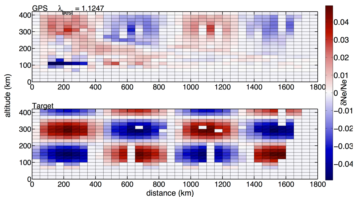
Figure 1.9: L'inversion conjointe des données simulées du radar trans-horizon et du GPS (haut) pour un test de damier.
