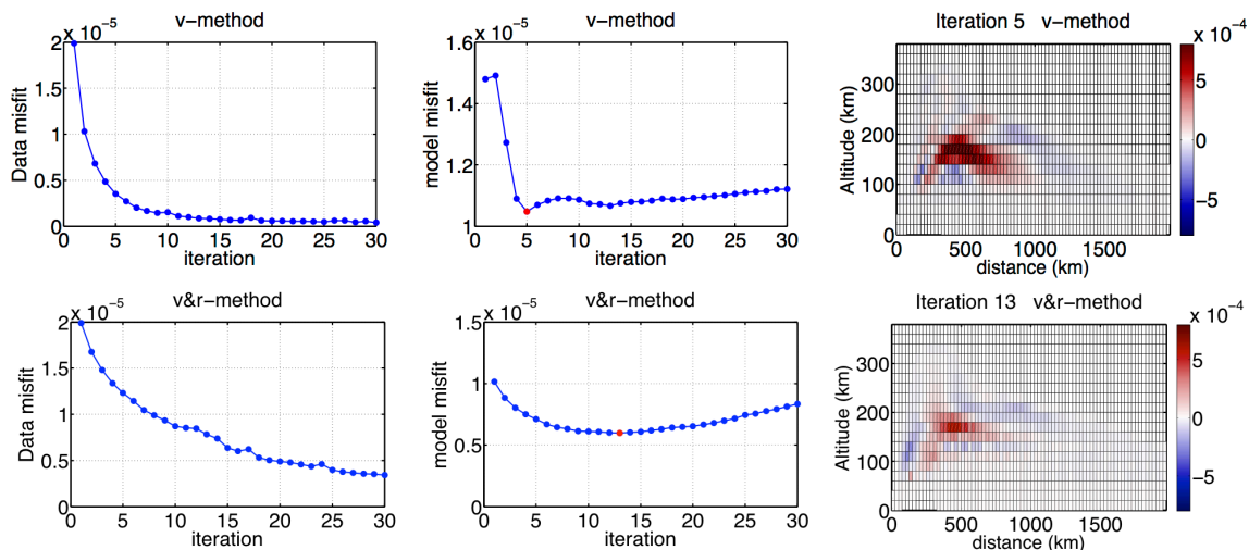
Figure 1.7: Ecarts en temps de propagation et des écarts par rapport au modèle cible avec les itérations pour la méthode v (haut) et la méthode v&r (bas). Roy et al. (2014)
