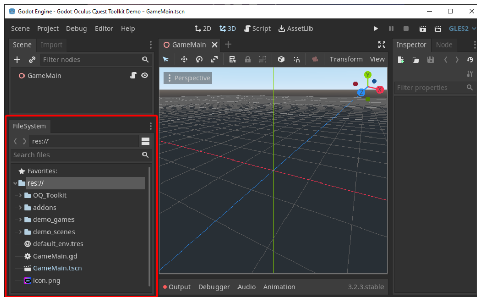
FIGURE I.2.3 – Asset manager (encadré en rouge) dans Godot.
