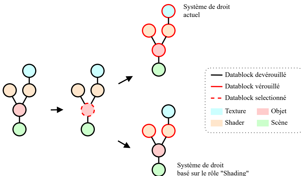
FIGURE II.3.6 – Comportement du système de droit actuel et idéal lors de la sélection d’un objet dans la scène.
