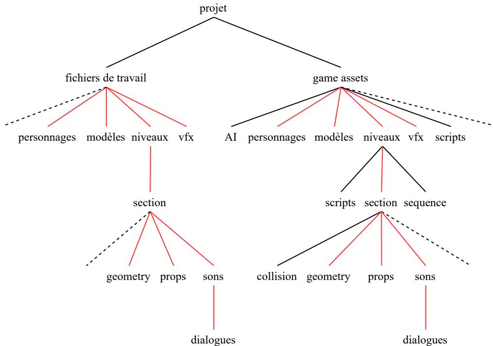
FIGURE I.2.2 – Exemple de structure de dossier en miroir (représentée en rouge).
