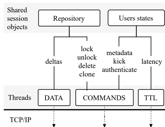
FIGURE II.1.3 – Architecture interne du serveur avec une réception synchrone des paquets réseau.
