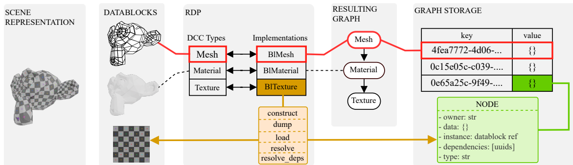
FIGURE II.1.4 – Traduction des données avec le RDP
