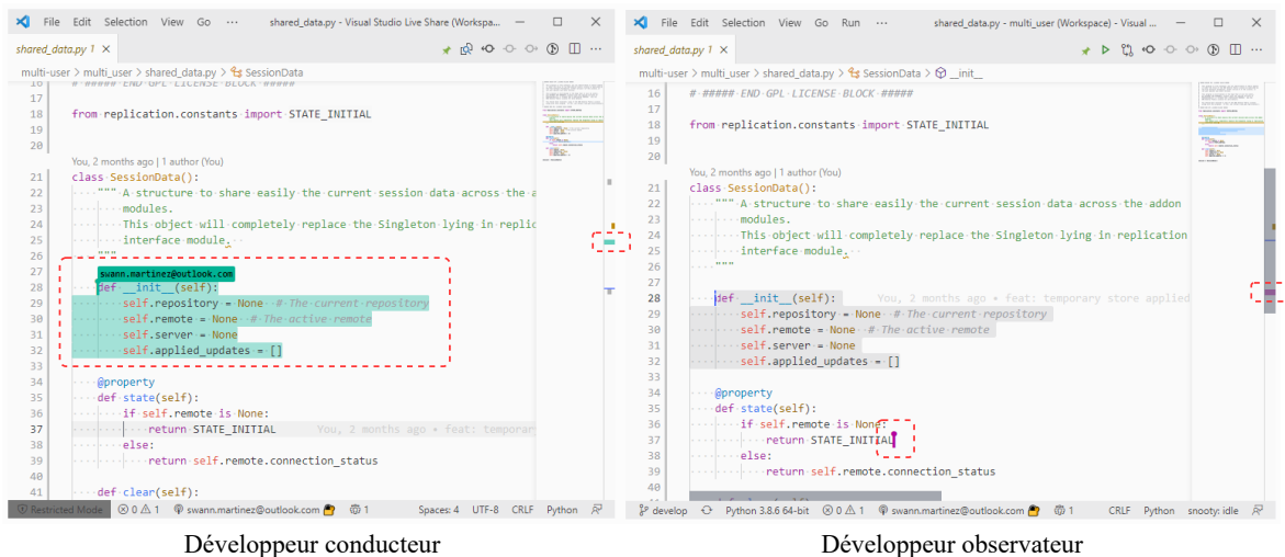
FIGURE I.3.3 – Pair programming en temps réel entre deux développeurs sur l'éditeur VS-Code .
