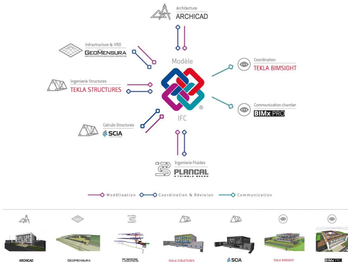
FIGURE I.3.2 – Exemple d'utilisation de BIM en se basant sur l' change de fichiers IFC dans diff rents corps de m tiers du BTP. Source : https://openbim.fr
