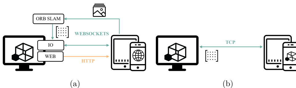
FIGURE I.2.10 – Architecture de la première (a) et de la seconde (b) itération de la Smartphone Remote .
