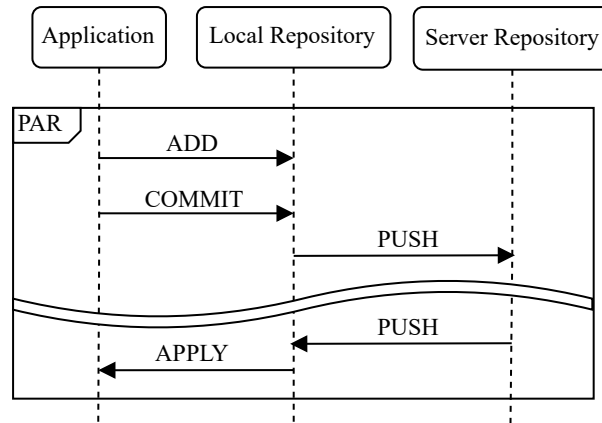
FIGURE II.1.5 – Pipeline des fonctions primitives de collaboration
