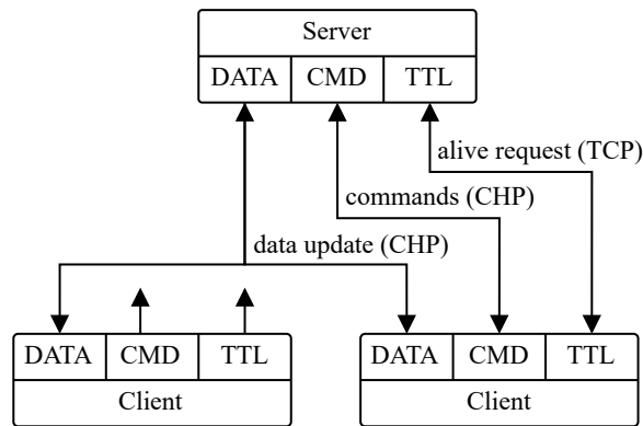
FIGURE II.1.2 – Couche de communication réseau
