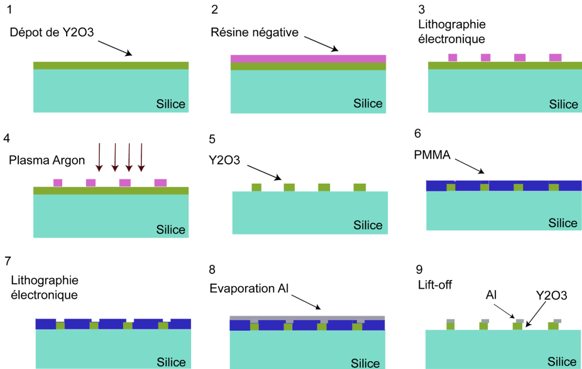
Figure 4.9 – Représentation schématique des différentes procédures de la nano-fabrication. 1) dépôt de Y_2O_3:Eu^{3+} , 2) dépôt d'une résine négative par spin coating, 3) nano-fabrication de bandelettes dans la résine par lithographie électronique, 4) attaque par Plasma Argon 5) ne laissant place qu'à des bandelettes de Y_2O_3:Eu^{3+} , 6) dépôt de PMMA par spin coating, 7) lithographie électronique pour placer et fabriquer les nano-antennes, 8) Évaporation thermique d'aluminium et 9) lift off et obtention de nano-antennes sur les bandelettes.
