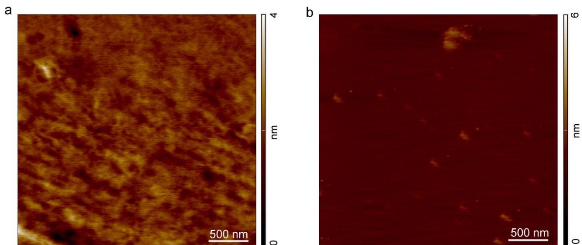
Figure 4.8 – a) Topographies de l'échantillon sur lequel une couche d'euporium d'une épaisseur de 100 nm a été déposée avec un recuit de 600°C et b) celui sur lequel une couche d'euporium d'une épaisseur de 16 nm a été déposée sans recuit.
