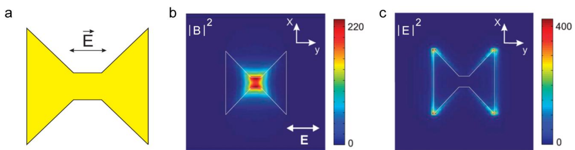
Figure 1.5 - a) schéma de la nano-antenne diabolo. b) distributions normalisées de l'intensité du champ magnétique et c) du champ électrique dans le plan transverse xy à 10 nm de distance de la nano-antenne à la longueur d'onde de 1940 nm. Le vecteur E représente la polarisation. 35
