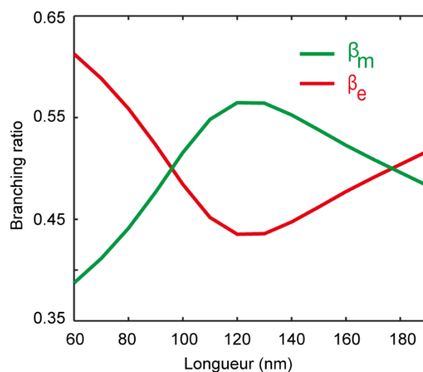
Figure 3.3 – Branching ratio théoriques associés aux dipôles isotropes magnétique (vert) et électrique (rouge) placés au centre d'une nano-antenne dipolaire en aluminium de longueur variable.
