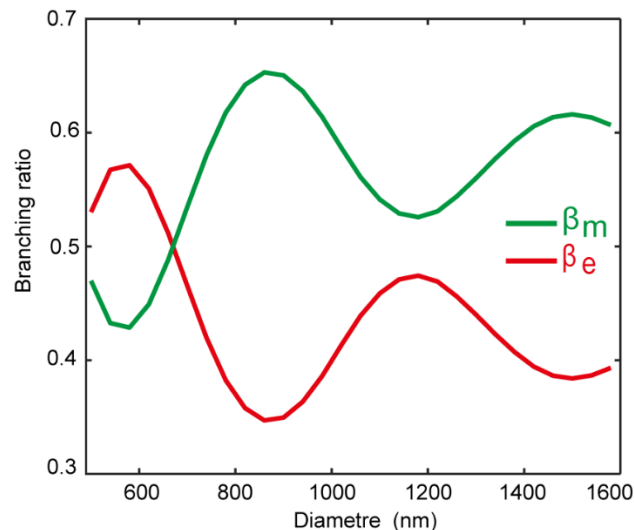
Figure 3.7 – Branching ratio théoriques associés aux dipôles isotropes magnétique (vert) et électrique (rouge) placés au centre d'une cavité plasmonique circulaire de diamètre variable.
