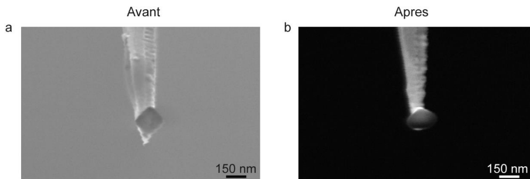
Figure 3.5 – a) Image MEB d'une pointe contenant une nano-particule dopée en euporium \text{Eu}^{3+} avant et b) après usinage de la pointe par FIB.
