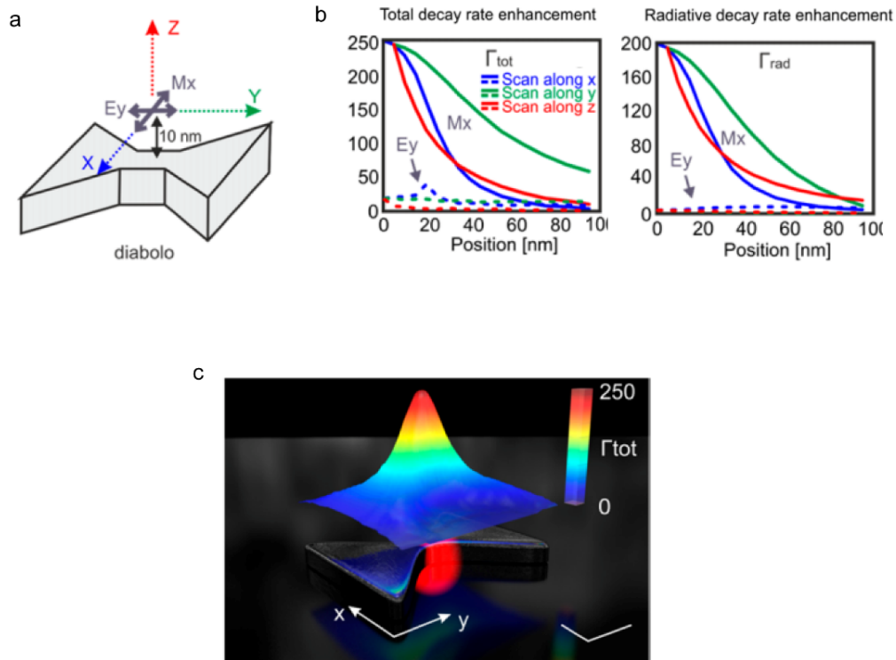
Figure 1.15 - a) Représentation en 3D d'un dipôle magnétique M_x et électrique E_y à proximité de la jonction métallique de la nano-antenne diabolique. b) Taux de décroissance total et c) radiatif du dipôle électrique (ligne discontinue) et du dipôle magnétique (ligne continue) en fonction de la position des dipôles par rapport à la structure. c) MLDOS dans un plan transverse à proximité de la nano-antenne diabolique. 25
