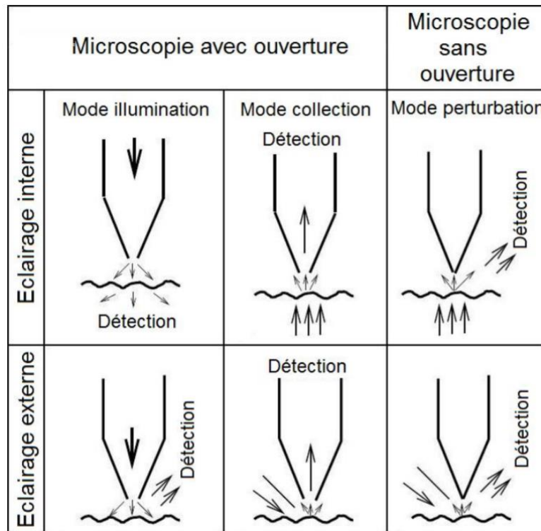
Figure 2.1 - Principales configurations du microscope optique en champ proche suivant le type d'éclairage (interne ou externe) et suivant la forme de la sonde ( avec ou sans ouverture). 1
