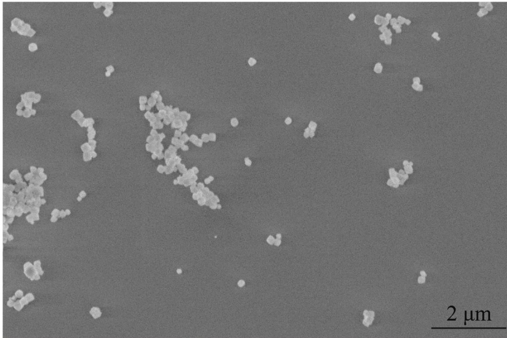
Figure 2.8 - Image MEB des nano-particules de KY_7F_{22} dopées à 5% d'europium Eu^{3+} déposées sur un substrat de silice.
