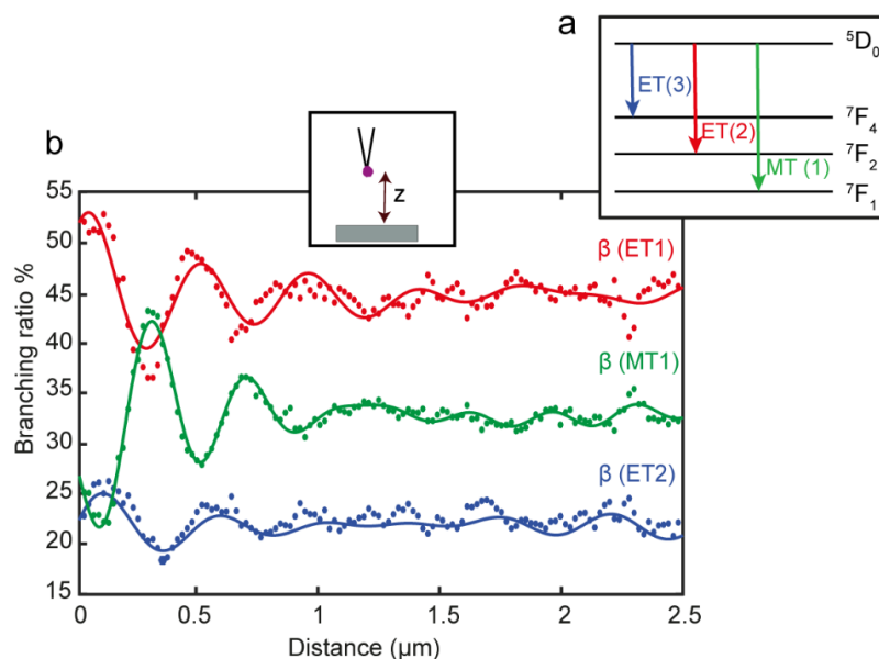
Figure 2.9 – a) Diagramme de bande partiel des ions europium. b) Taux de branchement associés aux transitions électriques et magnétiques de l'europium \text{Eu}^{3+} en fonction de la distance par rapport à un miroir en aluminium. Les points rouges, verts et bleus représentent respectivement les données expérimentales pour les transitions ET (2), MT (1) et ET (3), les traits pleins correspondent à un ajustement de type smoothing spline.
