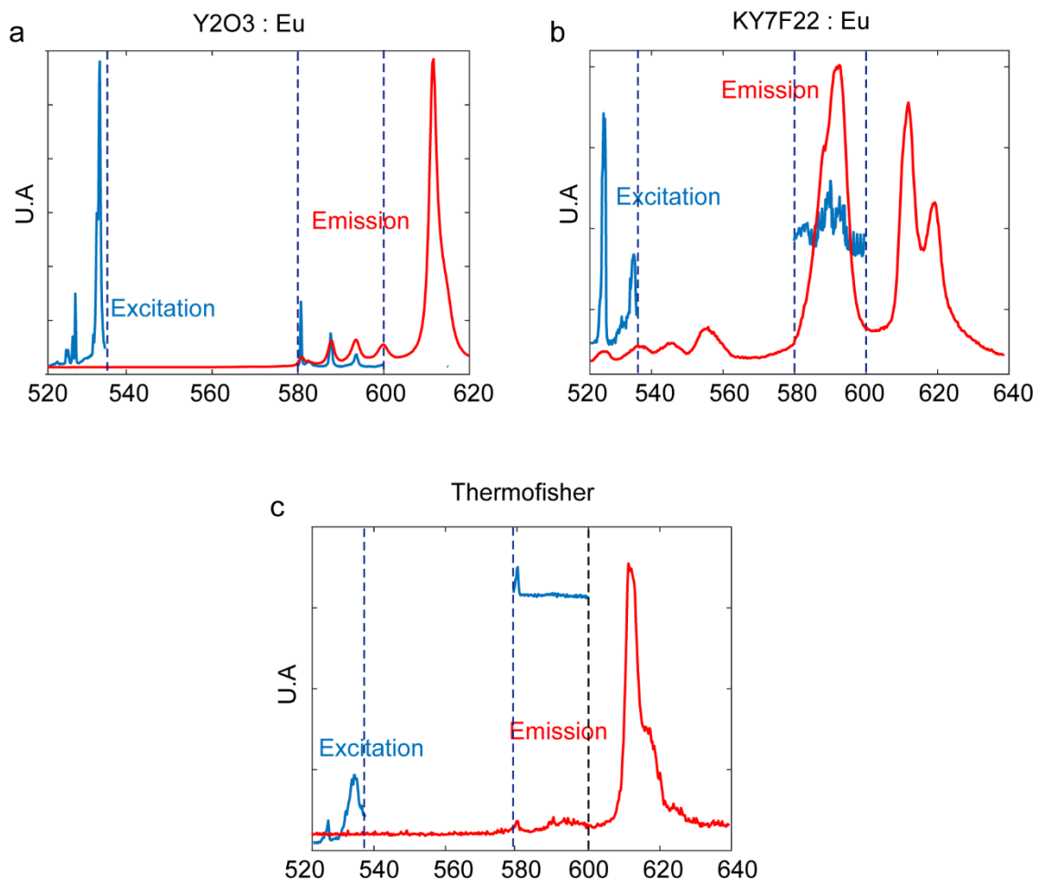
Figure 4.6 – Spectres d'excitation (bleu) et d'émission (rouge) des différentes nano-particules : a) \text{Y}_2\text{O}_3 : \text{Eu}^{3+} , b) \text{KY}_7\text{F}_{22} : \text{Eu}^{3+} et c) les nano-particules d'euporium de chez Thermofisher. Les spectres d'émission sont tracés pour une longueur d'onde d'excitation de a) 533,8 nm, b) 525,6 nm et c) 534,6 nm. Les spectres d'excitation sont obtenus en traçant la valeur crête de l'émission de la transition dipolaire électrique {}^5\text{D}_0 \rightarrow {}^7\text{F}_2 en fonction de la longueur d'onde d'excitation comprise entre 520 à 535 nm et 580 à 600 nm. Les lignes en pointillé indiquent la zone où les spectres d'excitation sont calculés
