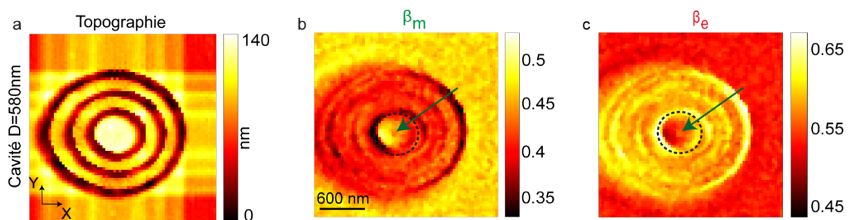
Figure 3.10 – a) Topographie de la surface scannée contenant la cavité plasmonique de diamètre D = 560 nm. La taille de l'image est de 3 \times 3 \mu\text{m}^2 . b) Branching ratio magnétique et c) électrique de la partie scannée. Les cercles noirs en pointillé délimitent la cavité, et les flèches indiquent le centre de la cavité. Durée approximative d'obtention de l'image : une heure.
