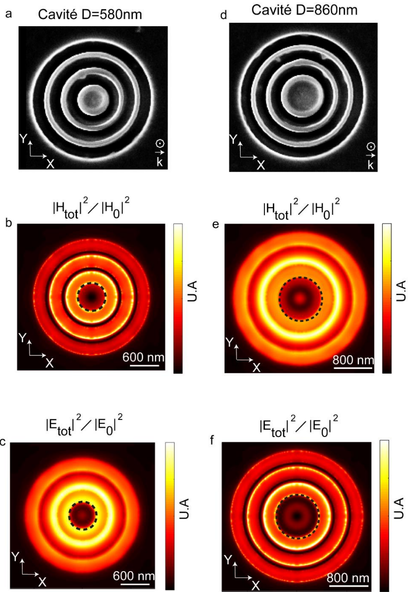
Figure 3.8 – a) Images MEB des cavités circulaires électrique (diamètre D= 580\text{nm} ) et d) magnétique (diamètre D = 860 \text{ nm} ) étudiées en vue de dessus (plan XY), où k est la direction de propagation du faisceau incident dans les simulations. E est polarisé circulairement. Simulations des distributions de l'intensité des champs b,e) magnétiques et c,f) électriques dans le plan longitudinal XY à 20 nm des cavités b,c) électriques et e,f) magnétiques. Sur les distributions, les cercles noirs en pointillés délimitent les groove de l'intérieur des cavités.
