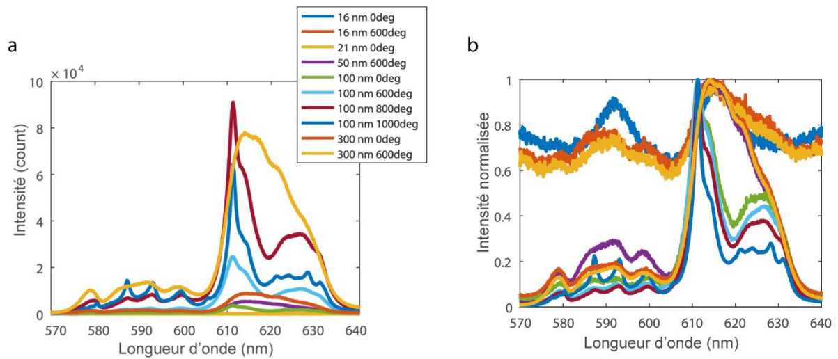
Figure 4.7– a) Spectres d’émission des différentes épaisseurs de Y 2 O 3 dopées en europium avec et sans recuit (en encart) obtenus lors d’une excitation par un laser pulsé de 473 nm. b) est le spectre normalisé de a).
