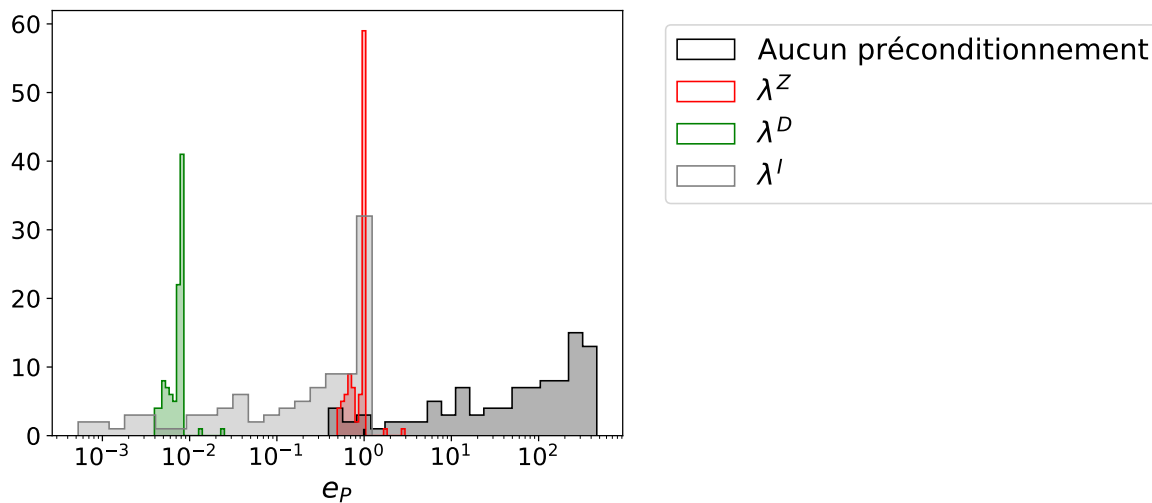
FIGURE 2.9 – Histogrammes de e_p(\mathbf{x}, \lambda(\mathbf{x})) défini dans l'Eq. (2.67) pour le PIO obtenu pour les différents coefficients ainsi que sans préconditionnement pour le cas 1D.
