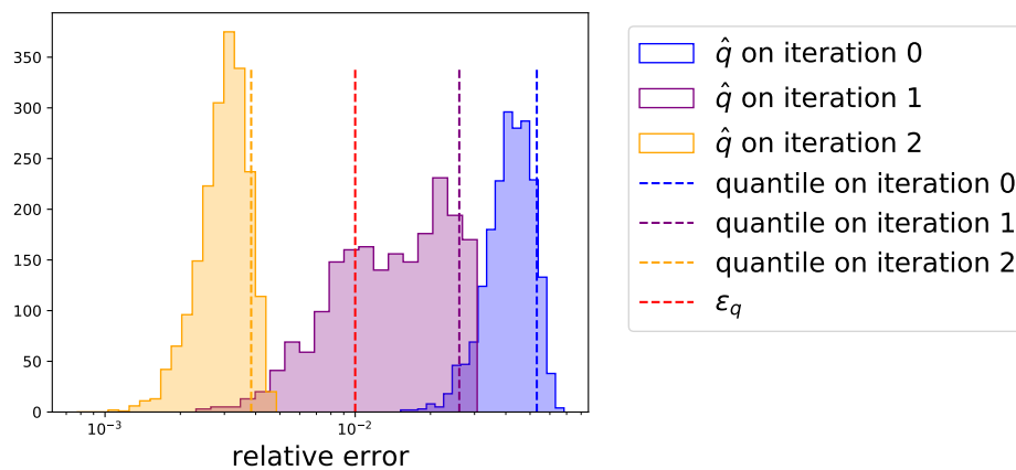
FIGURE 3.28 – Problème à 8 variables de design, histogramme et quantile à 90% de \hat{q} au cours des itérations de l'Algorithme 13 lors de la résolution de la MDA \mathbf{x} = \mathbf{x}_1^{\text{DoE}} avec le solveur DPOD+I.
