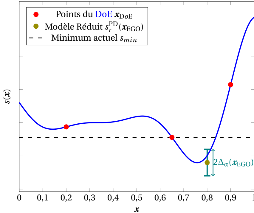
FIGURE 2.6 – Illustration du cas où la réduction de modèle ne permet pas de conclure sur la non-optimalité de \mathbf{x}_{EGO} , un appel au solveur sera nécessaire pour calculer s(\mathbf{x}_{EGO}) .
