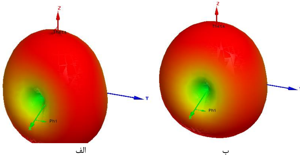
شکل 3-8: پترن تشعشی اندازه گیری شده ی آنتن فراکتال تک قطبی در فرکانس های 2/45، 2/6، 5/2، 5/8 گیگاهرتز الف) صفحه H ب) صفحه E با مقادیر اشاره شده در جدول 3-1 و پترن تشعشی سه بعدی آنتن مذکور در فرکانسهای الف) 5/8 و ب) 2/6 گیگاهرتز.
