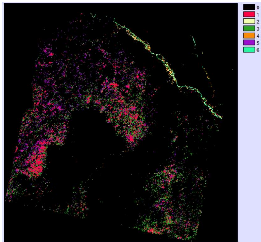
Figure 27 : Classification non dirigée du masque « brûlis-sol humide-eau » en six classes à partir des composantes principales
