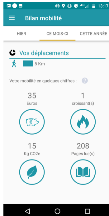
Figure 34 : Bilan mensuel (coût, calories, CO2 et pages lues)
