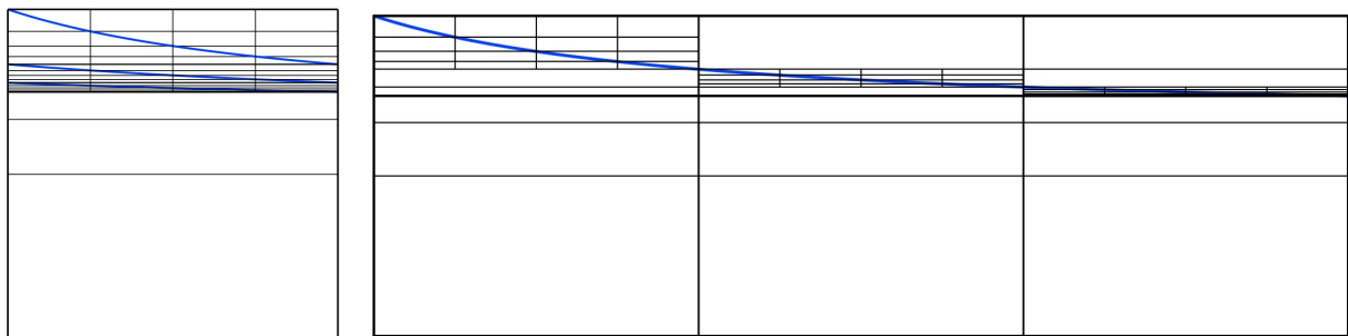
Exemple pour p = 4 (A gauche la figure dans le carré unité, à droite le recollement)
