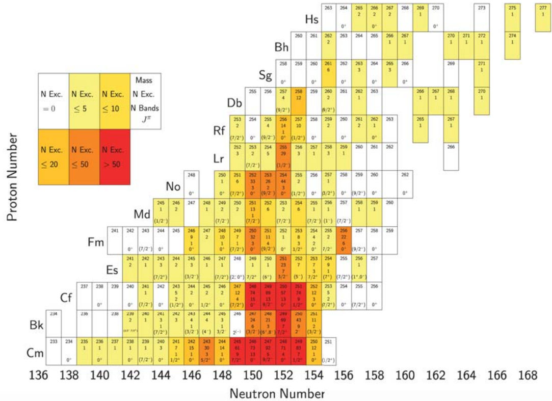
FIGURE 3.3 – Résumé des données expérimentales disponibles du Cm (Z=96) au Hs (Z=108). On y retrouve le nombre de masse A, le nombre d'états excités connus, le nombre de bande de rotations connues et le spin du niveau fondamental pour chaque isotope. Figure extraite de [128].
