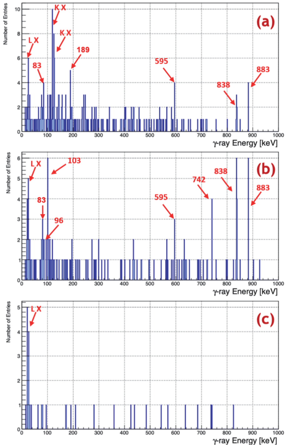
FIGURE 4.15 – Spectre des rayons \gamma observés en coïncidence avec les cascades de 3 (ER- e_1 - e_2 - e_3 ). (a), (b) et (c) correspondent respectivement aux coïncidences avec e_1 , e_2 et e_3 . \gamma spectrum in coincidence with cascades of 3 (ER- e_1 - e_2 - e_3 ). (a), (b) and (c) shows respectively the coincident \gamma -rays with e_1 , e_2 and e_3 .
