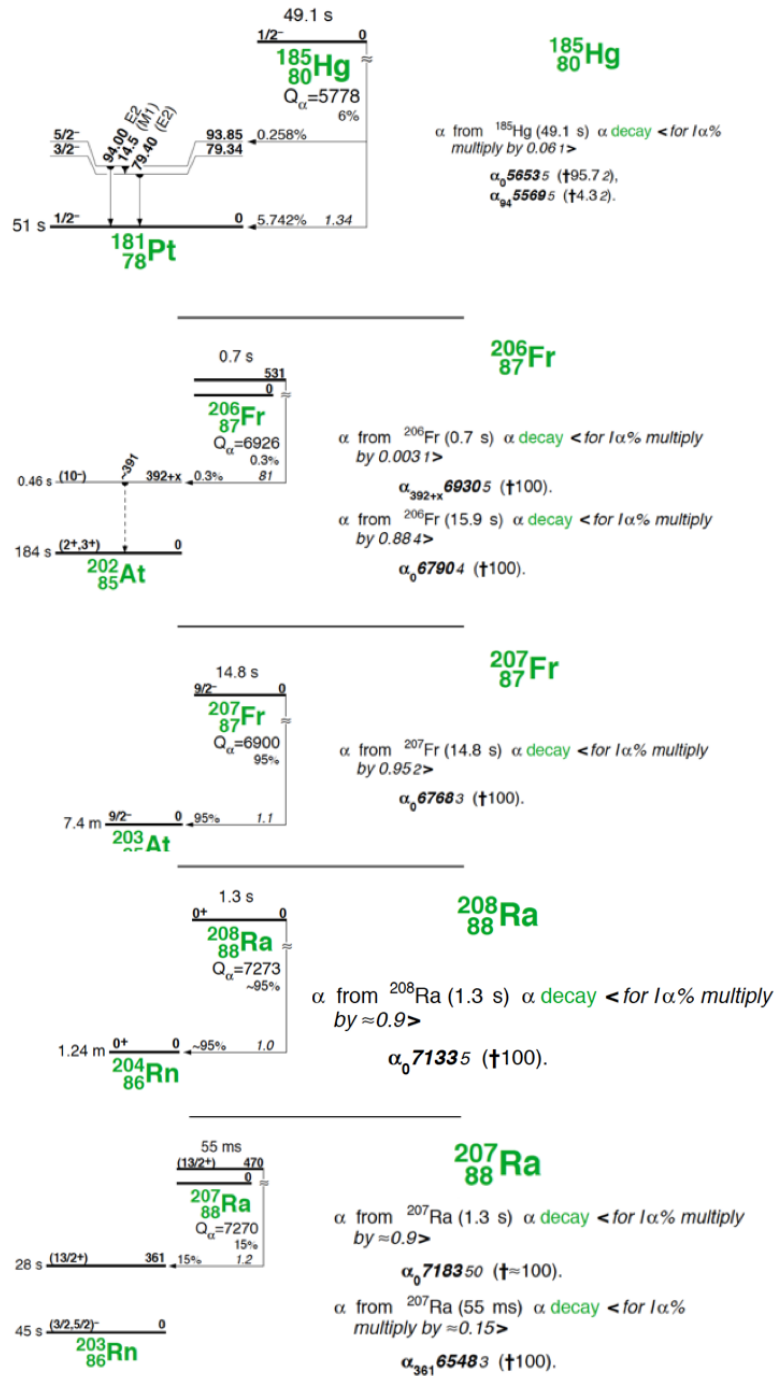
FIGURE 5.7 – Schémas de niveau des isotopes utilisés pour étalonner nos détecteurs, issus des réactions ^{51}\text{V}+^{139}\text{La}\rightarrow^{185}\text{Hg}+5n et ^{51}\text{V}+^{159}\text{Tb}\rightarrow^{210-xn}\text{Ra}+xn [57]. Level scheme of isotopes used for the detectors calibrations, synthesized through the fusion-evaporation reactions ^{51}\text{V}+^{139}\text{La}\rightarrow^{185}\text{Hg}+5n et ^{51}\text{V}+^{159}\text{Tb}\rightarrow^{210-xn}\text{Ra}+xn [57].
