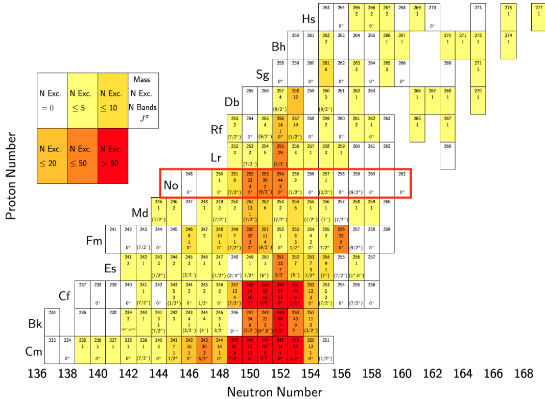
FIGURE 4.1 – Résumé des données expérimentales disponibles du Cm ( Z=96 ) au Hs ( Z=108 ). On y retrouve le nombre de masse, le nombre d'états excités connus, le nombre de bande de rotations connues et le spin du niveau fondamental pour chaque isotope. Figure extraite de [128].
