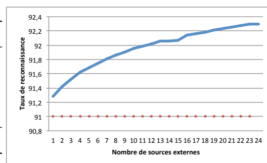
Figure 2.5: Tableau de gauche : taux de reconnaissance intra-domaine sur Books , DVD , Electronics et Kitchen . Courbe de droite : évolution du taux (moyenné sur les 4 expériences) lorsque l'ensemble d'apprentissage est enrichi avec des sources externes.
