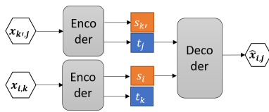
Figure 4.14: Procédure d'apprentissage de représentation démêlée : la reconstruction du signal associé aux contextes i, j est effectuée à partir de deux autres signaux i, k et k', j afin de capturer les aspects spécifiques aux contextes i et j .
