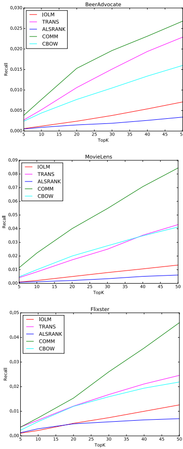
Figure 3.9: Performance dans la prédiction du prochain item visité, au sens du rappel@ k , en fonction de k . Les différents modèles testés correspondent à l'état de l'art : IOLM [Che+12b], ALSRank [TT12], CBOW (=word2vec) [Mik+13]. Trans et Comm correspondent à nos deux modèles, respectivement en translation simple ou avec un endomorphisme appris par communauté.
